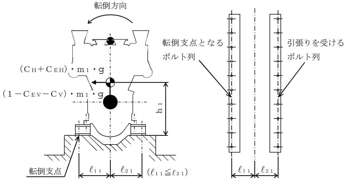
図 3-2 計算モデル（軸直角方向転倒）
