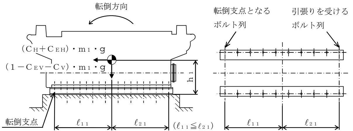
図 3-3 計算モデル（軸方向転倒）
