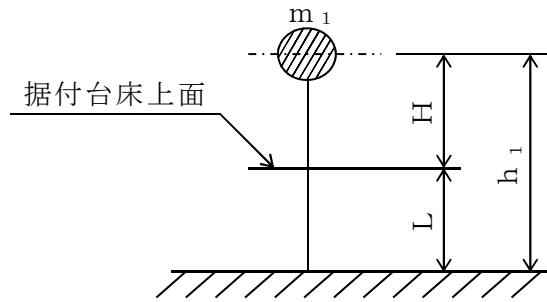
図 3-1 固有周期の計算モデル
