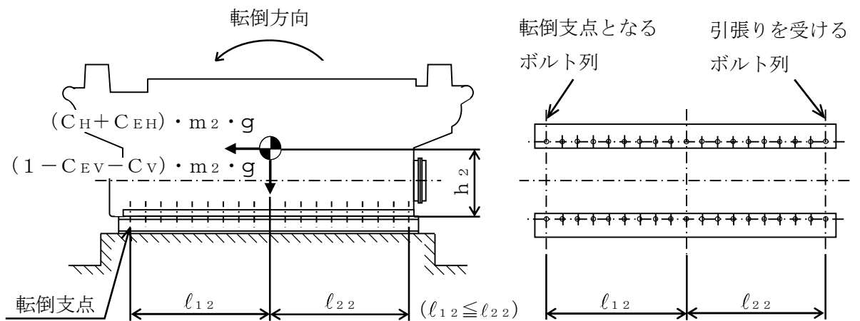
図 3-5 計算モデル（軸方向転倒）
