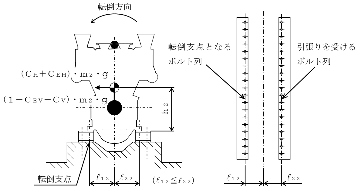
図 3-4 計算モデル（軸直角方向転倒）
