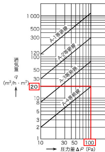
図 1—気密等級線
