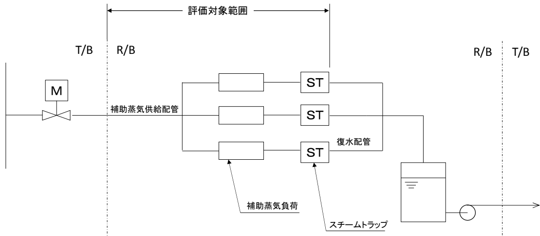
2-3 図 所内蒸気系統 概要図
