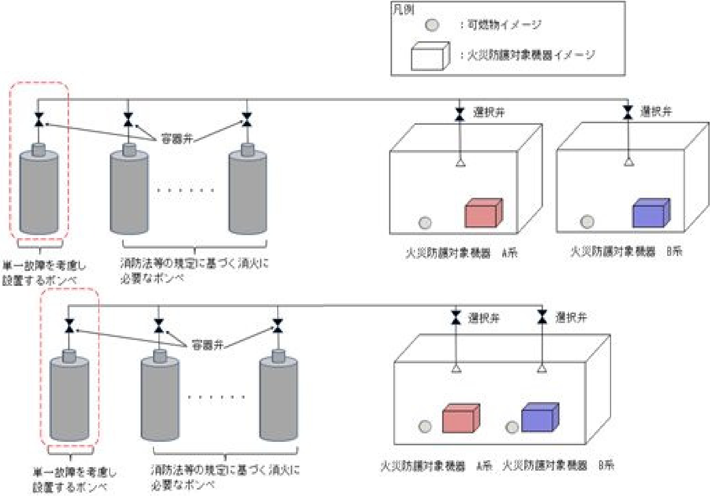
第6-7図 ハロゲン化物自動消火設備（全域）の系統構成
