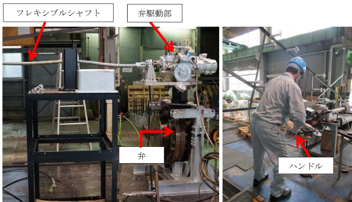
第6図 モックアップ試験の概要 (2/2)
