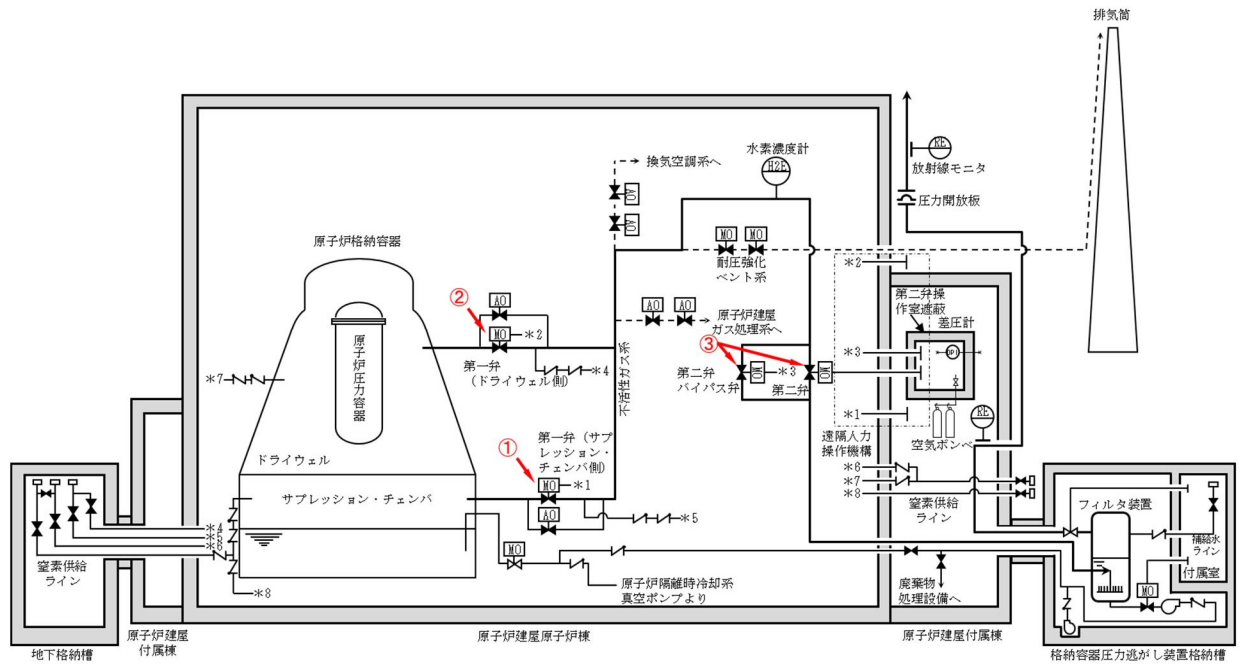
第4-1図 格納容器圧力逃がし装置機能検査対象弁
