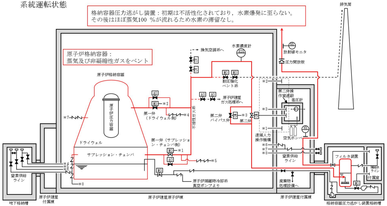
第8図 水素爆発防止対策（系統運転状態）
