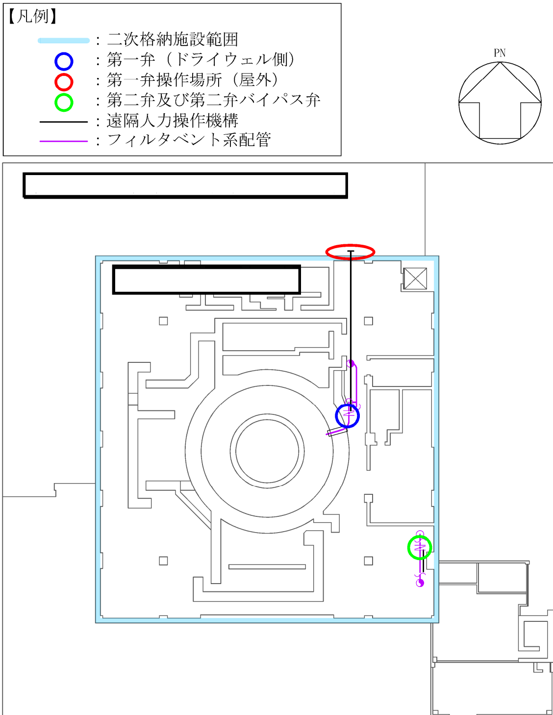
第 2 図 隔離弁の操作場所 (2/3)
