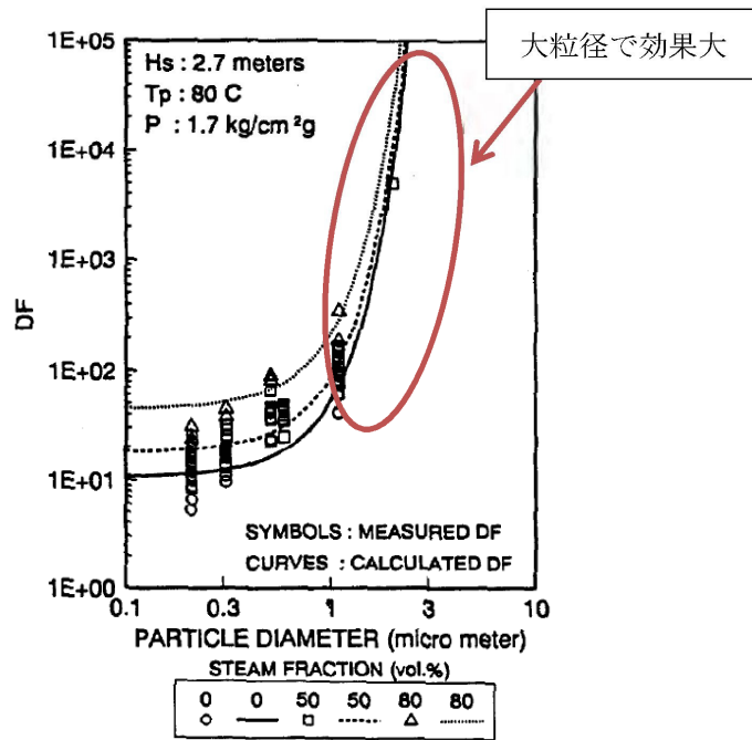
第 13 図 プールスクラビングによる除去性能の例 (参考図書 3)
