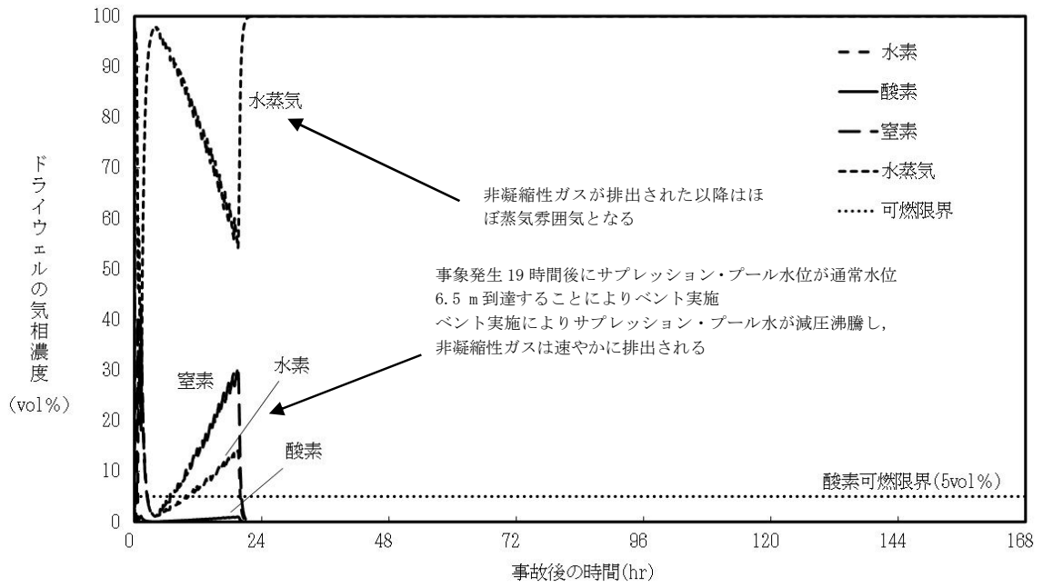
第 14 図 「雰囲気圧力・温度による静的負荷（格納容器過圧・過温破損） （代替循環冷却系を使用できない場合）」における ドライウエルの気相濃度の推移（ウェット条件）
