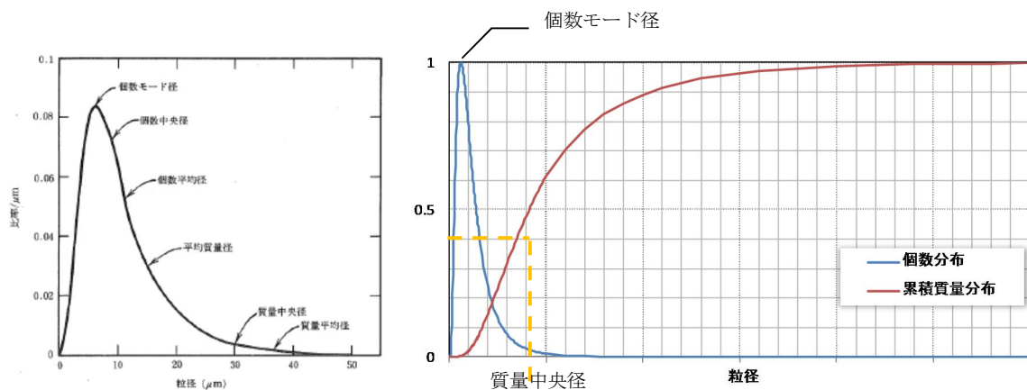
第5図 個数分布と累積質量分布
