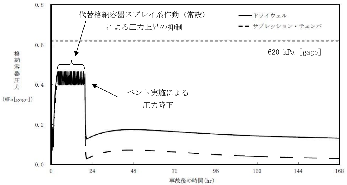
第1図 「雰囲気圧力・温度による静的負荷（格納容器過圧・過温破損）（代替循環冷却を使用できない場合）」における格納容器圧力の推移
