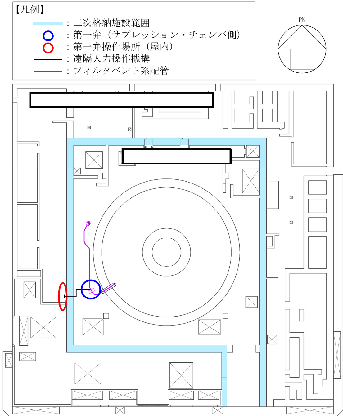
第 1 図 隔離弁の操作場所 (1/3)
