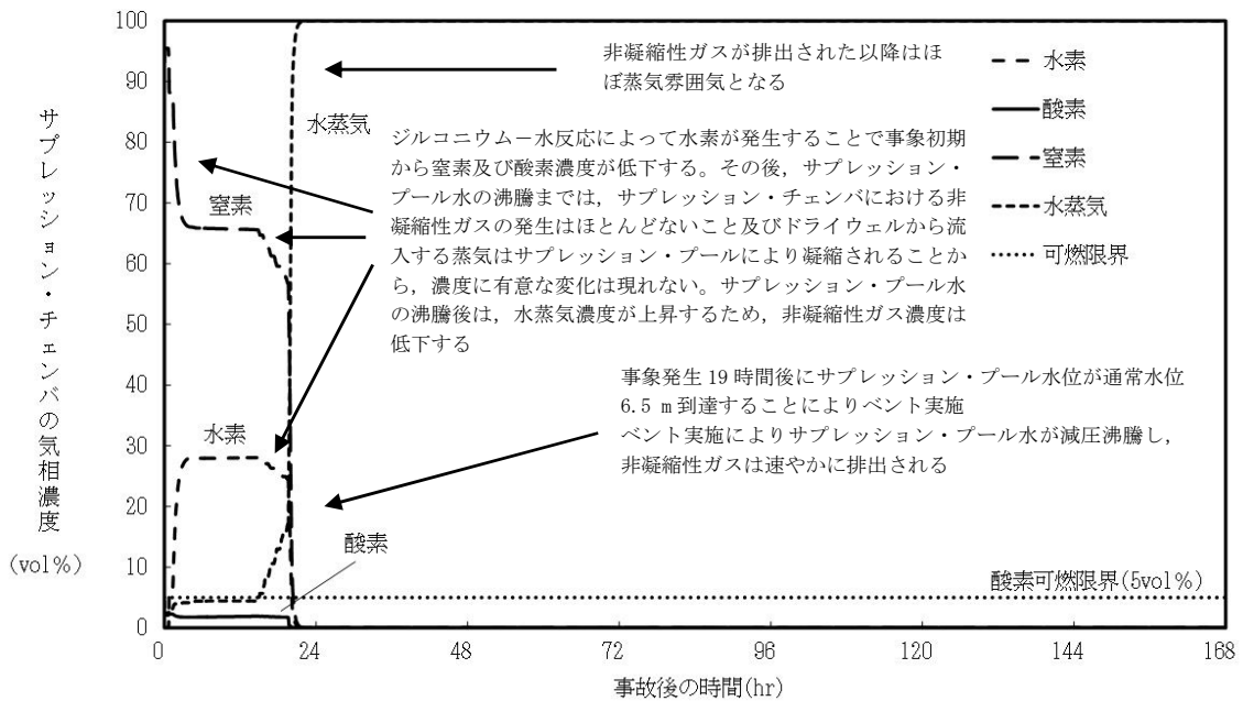
第 15 図 「雰囲気圧力・温度による静的負荷（格納容器過圧・過温破損） （代替循環冷却系を使用できない場合）」における サブプレッション・チェンバの気相濃度の推移（ウェット条件）
