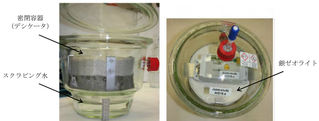
第3図 銀ゼオライトの保管の様子
