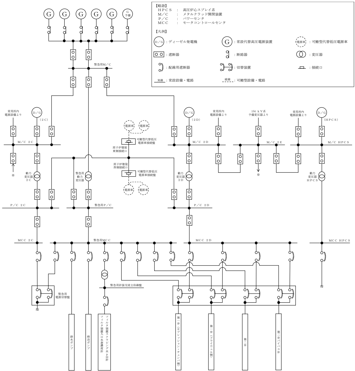
第 2.4.2-1 図 格納容器圧力逃がし装置 電源構成図 (交流電源)
