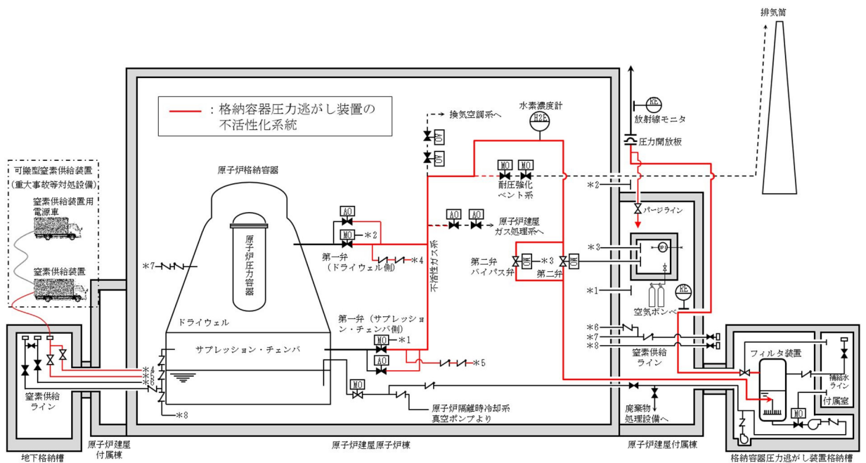
第16図 格納容器圧力逃がし装置の不活性化系統
