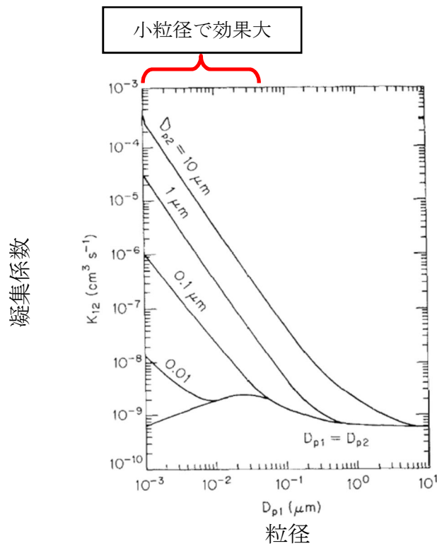
第9図 凝集効果の例
