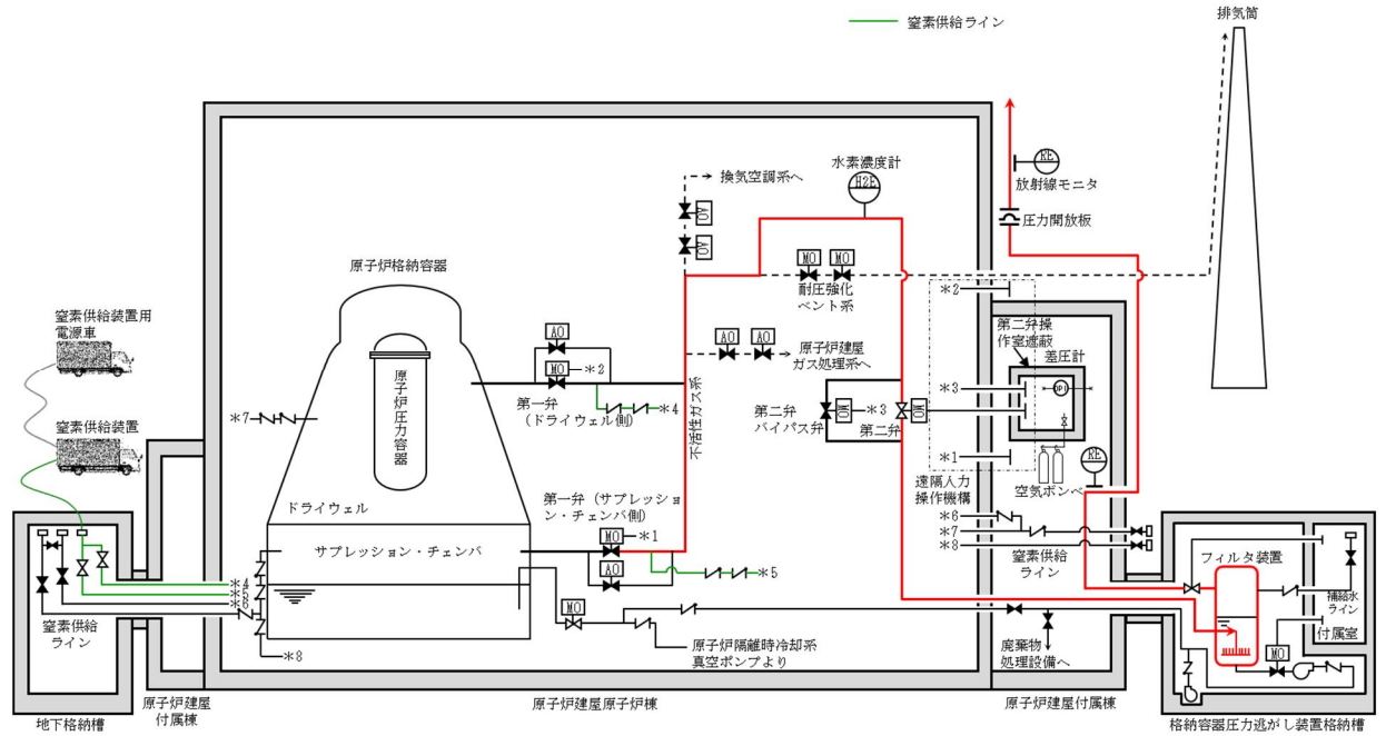
第 2. 4. 4-1 図 可搬型窒素供給装置概要図
