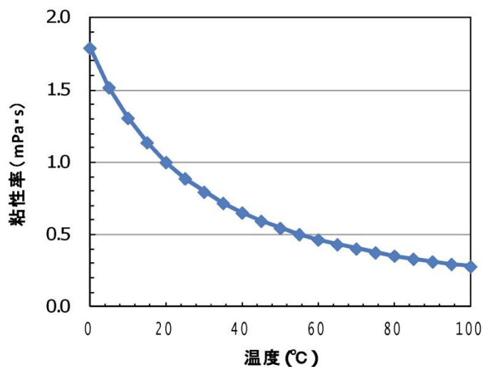
第7図 水の粘性率に及ぼす温度の影響
