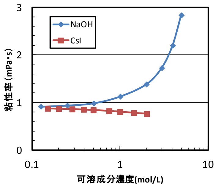
第5図 \text{NaOH} と \text{CsI} が水に溶解した場合の粘性率の変化（25℃） （ \text{NaOH} ：参考図書6， \text{CsI} ：参考図書7）
