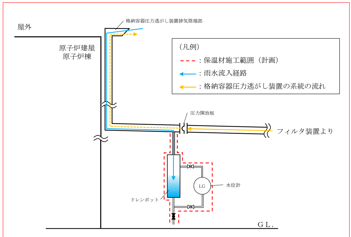
第2.4.6-1図 格納容器圧力逃がし装置排気筒排水設備概要図
