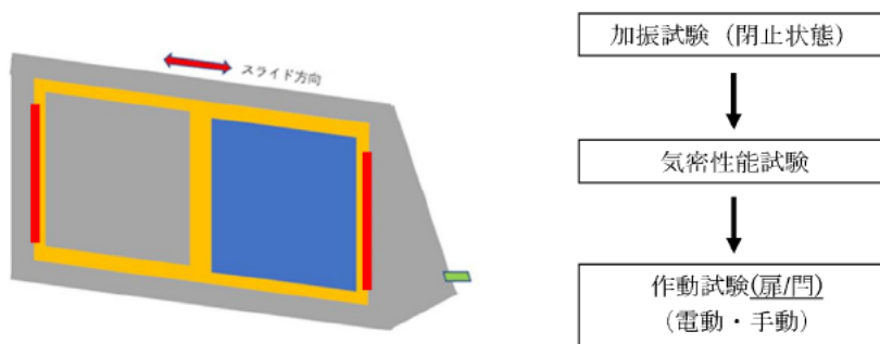
第1図 試験治具概念図
