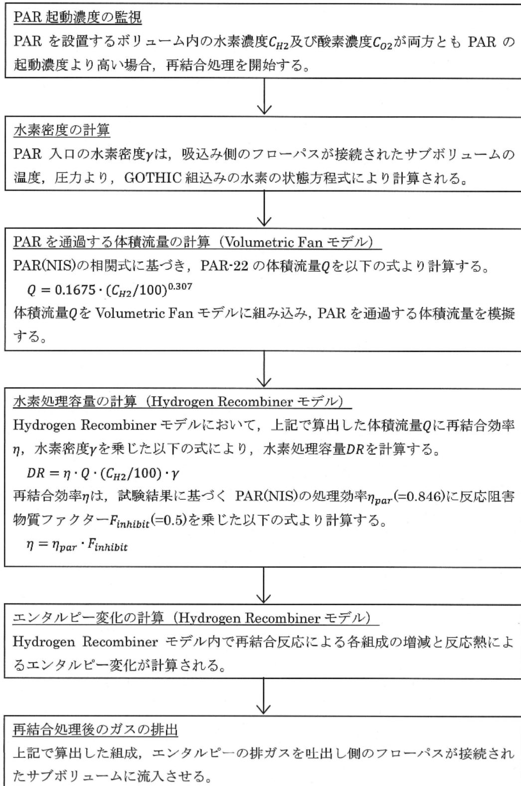
図14 PARの組み込みロジック
