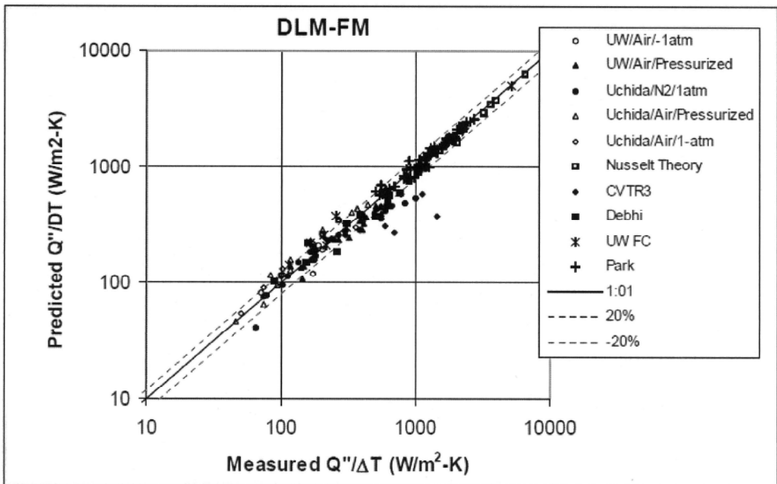
図11 DLM-FMモデルの試験データとの比較 (出典： [2] Fig.5-40)
