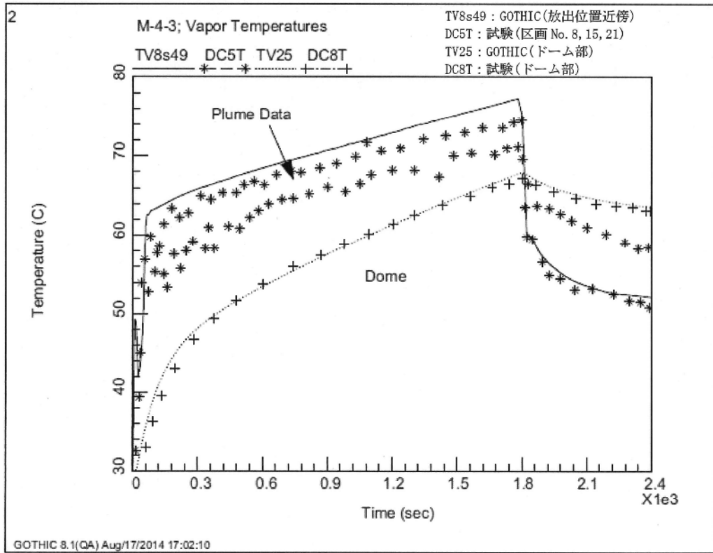
図9 格納容器温度 (出典: [2] Fig. 17-17)
