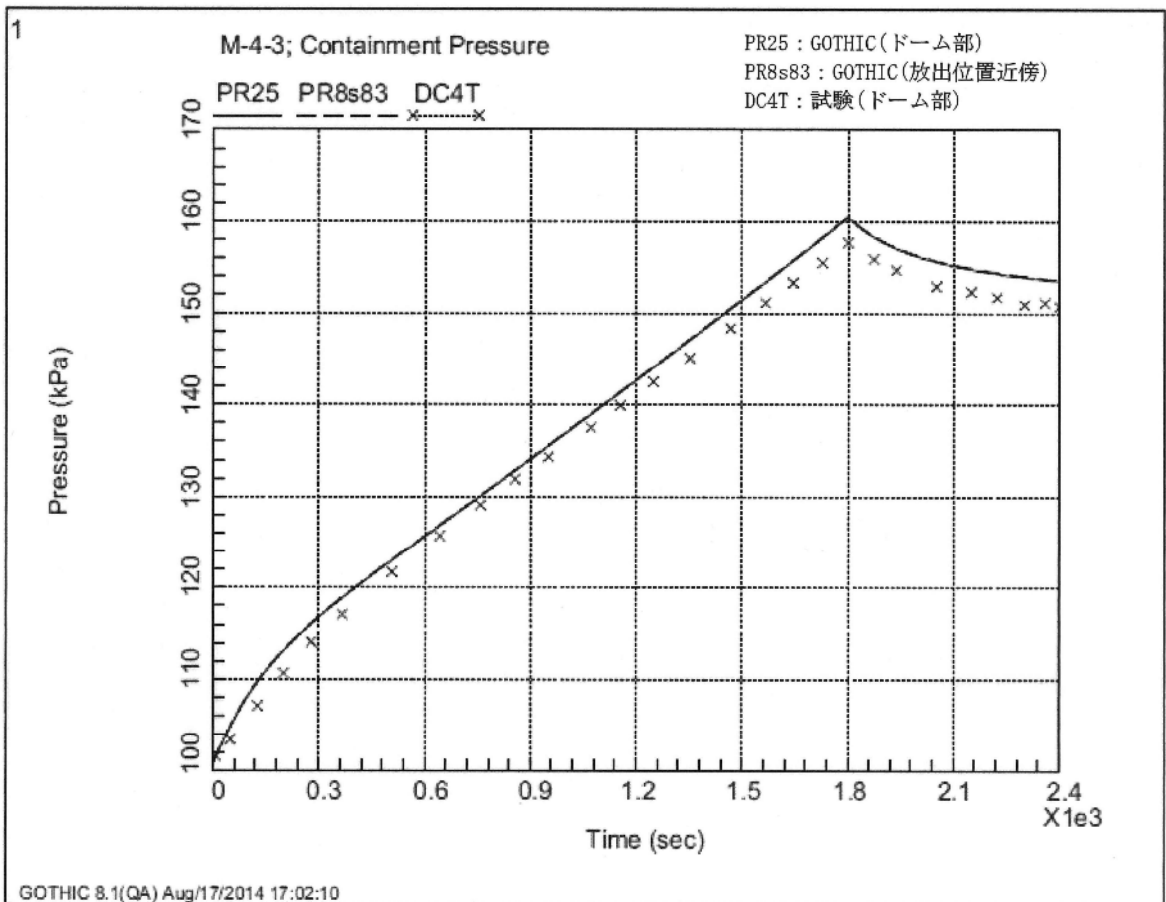
図8 格納容器圧力 (出典：[2] Fig.17-16)
