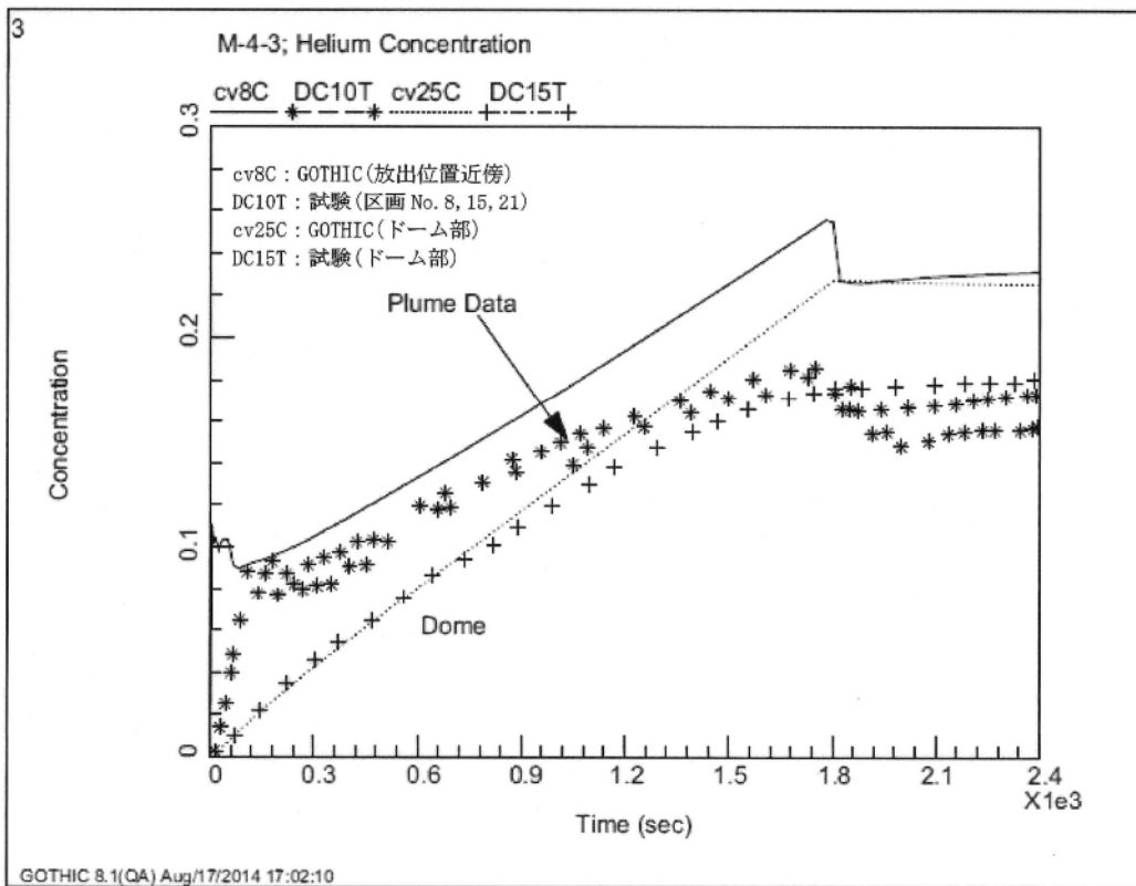
図10 ヘリウム濃度 (出典: [2] Fig. 17-19)
