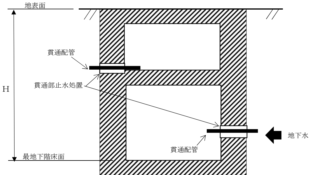
第4-1図 溢水による静水圧の算出に用いる浸水高さHの設定
