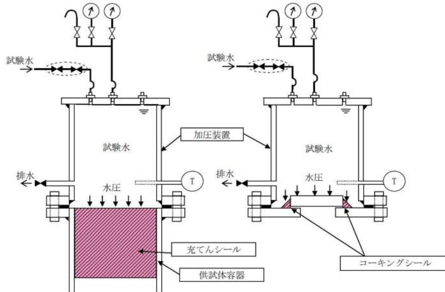
第3-1図 シール材の水圧試験の概要
