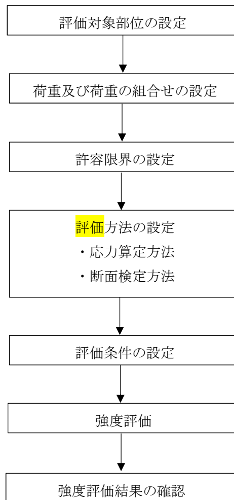
第2-2図 堰の強度評価フロー
