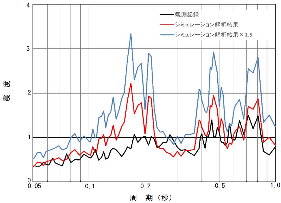
図 4-4 (4/4) 原子炉建屋 EL. -4.0m 床応答スペクトル比較 (減衰 1%)
