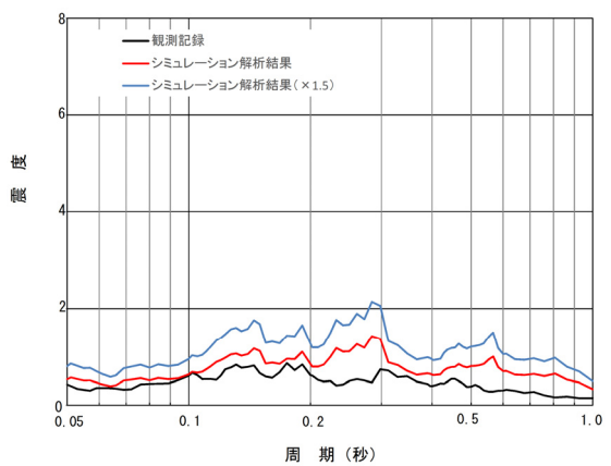
原子炉建屋 EL.14.0m 床応答スペクトル比較(減衰3.0%)
