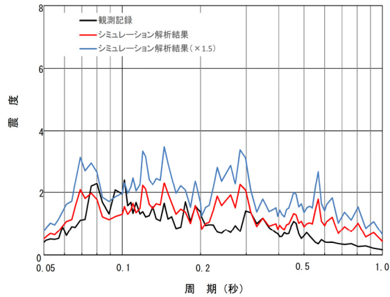
原子炉建屋 EL.29.0m 床応答スペクトル比較(減衰1.0%)
