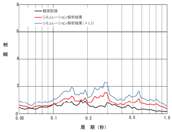
原子炉建屋 EL.14.0m 床応答スペクトル比較(減衰2.5%)
