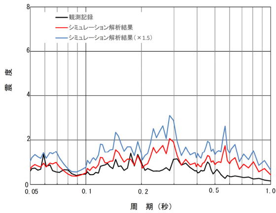
原子炉建屋 EL.-4.0m 床応答スペクトル比較(減衰1.0%)
