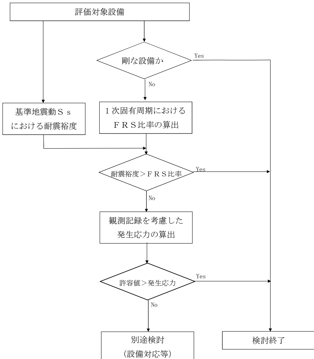
図 4-5 観測記録による影響評価フロー
