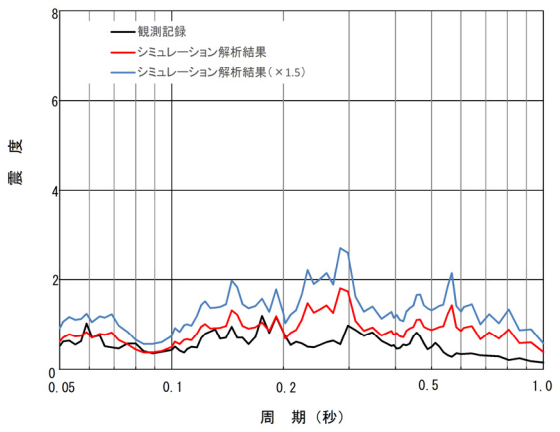
原子炉建屋 EL.-4.0m 床応答スペクトル比較(減衰1.5%)
