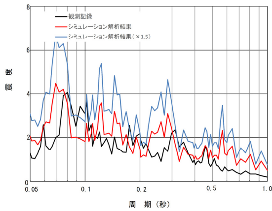
原子炉建屋 EL.46.5m 床応答スペクトル比較(減衰0.5%)
