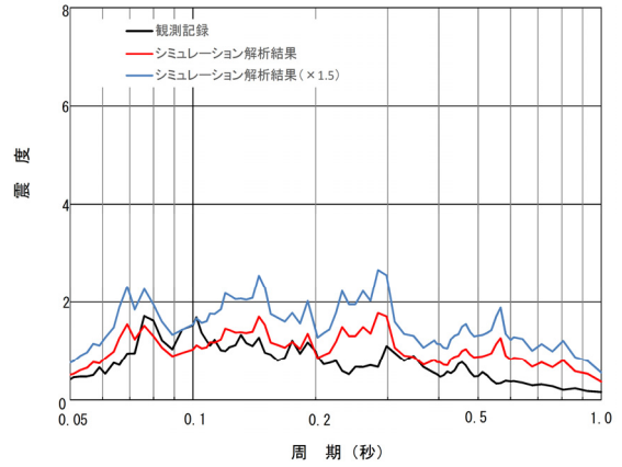
原子炉建屋 EL.29.0m 床応答スペクトル比較(減衰2.0%)
