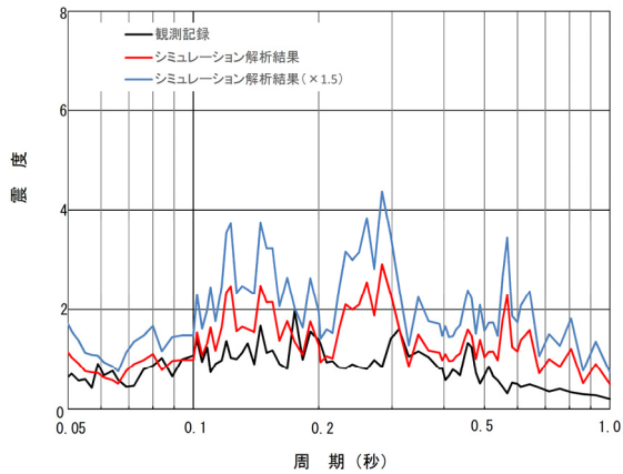
原子炉建屋 EL.14.0m 床応答スペクトル比較(減衰0.5%)
