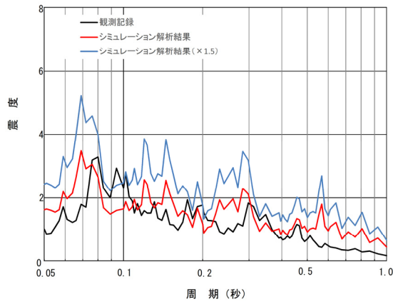
原子炉建屋 EL.46.5m 床応答スペクトル比較(減衰1.0%)
