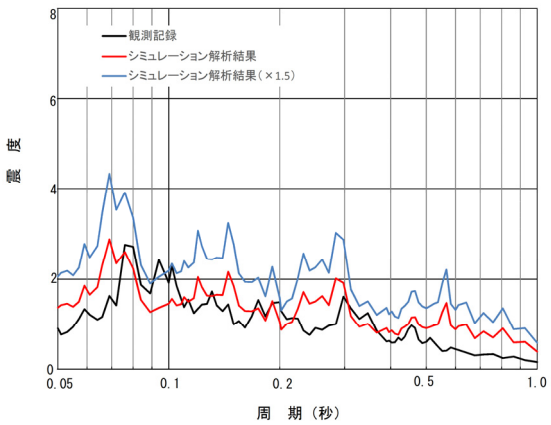
原子炉建屋 EL.46.5m 床応答スペクトル比較(減衰1.5%)
