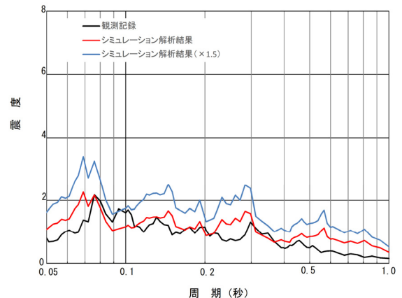
原子炉建屋 EL.46.5m 床応答スペクトル比較(減衰2.5%)
