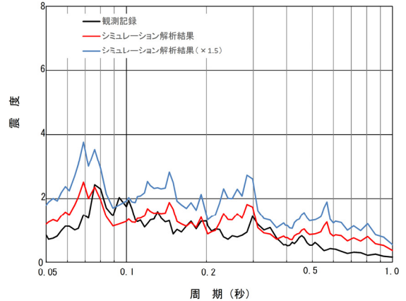
原子炉建屋 EL.46.5m 床応答スペクトル比較(減衰2.0%)
