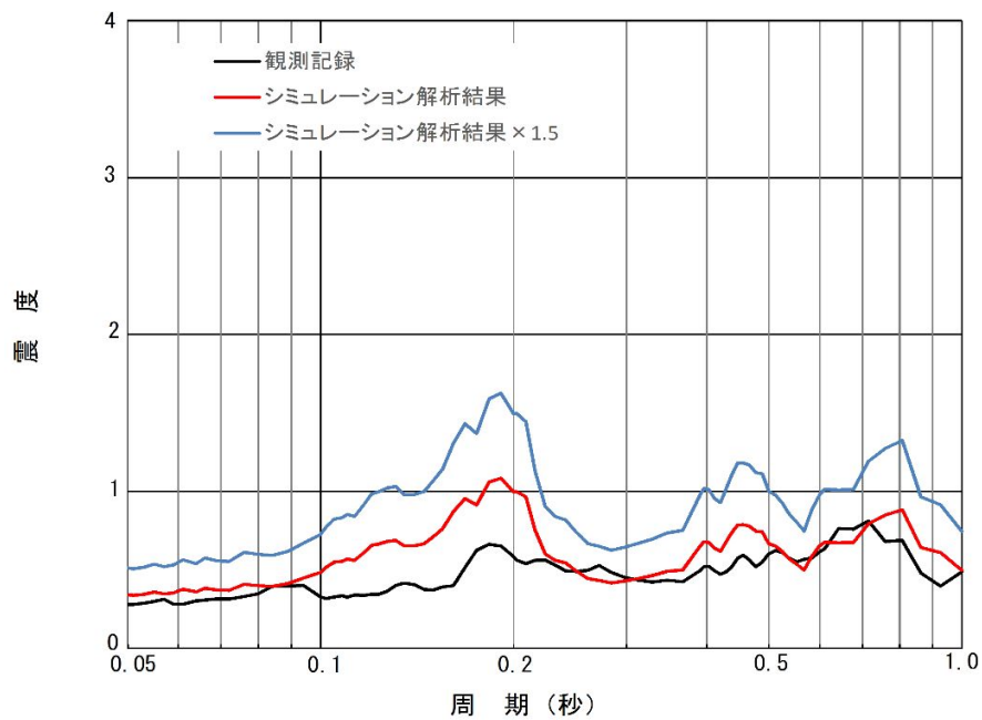
図 4-2 (4/4) 原子炉建屋 EL. -4.0m 床応答スペクトル比較 (減衰 5%)
