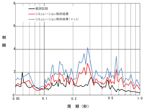
原子炉建屋 EL.-4.0m 床応答スペクトル比較(減衰0.5%)
