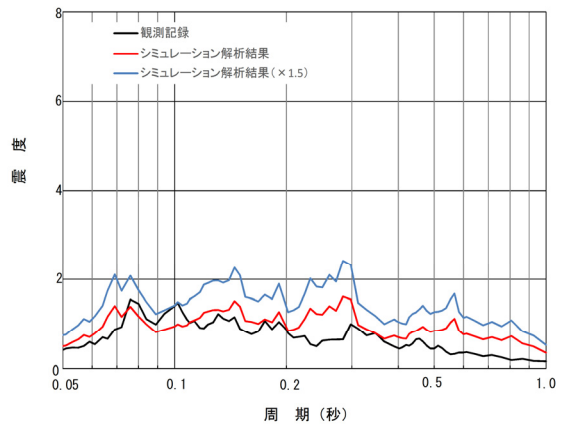
原子炉建屋 EL.29.0m 床応答スペクトル比較(減衰2.5%)
