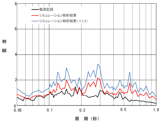
原子炉建屋 EL.14.0m 床応答スペクトル比較(減衰1.0%)
