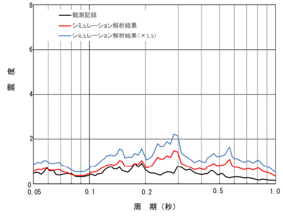
原子炉建屋 EL.-4.0m 床応答スペクトル比較(減衰2.5%)
