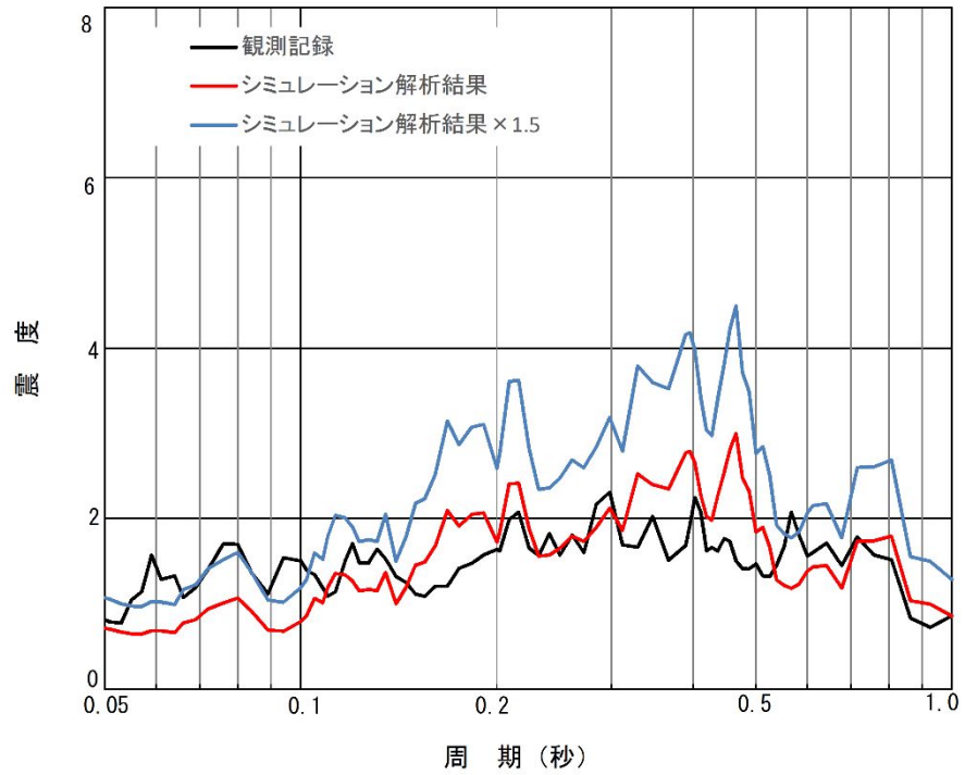
図 4-3 (1/4) 原子炉建屋 EL. 46.5m 床応答スペクトル比較 (減衰 2%)
