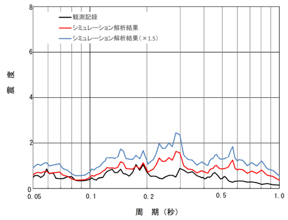
原子炉建屋 EL.-4.0m 床応答スペクトル比較(減衰2.0%)
