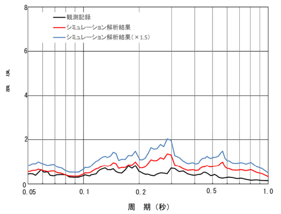
原子炉建屋 EL.-4.0m 床応答スペクトル比較(減衰3.0%)
