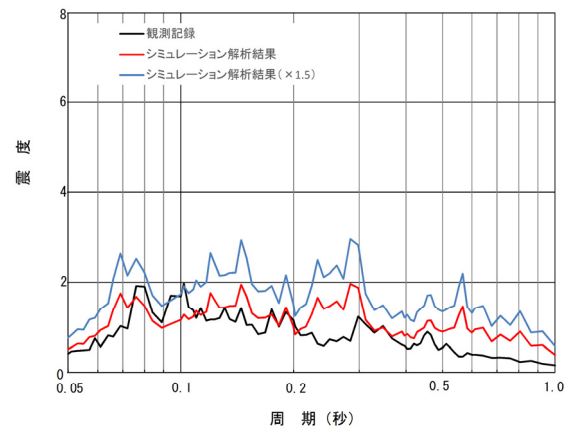
原子炉建屋 EL.29.0m 床応答スペクトル比較(減衰1.5%)
