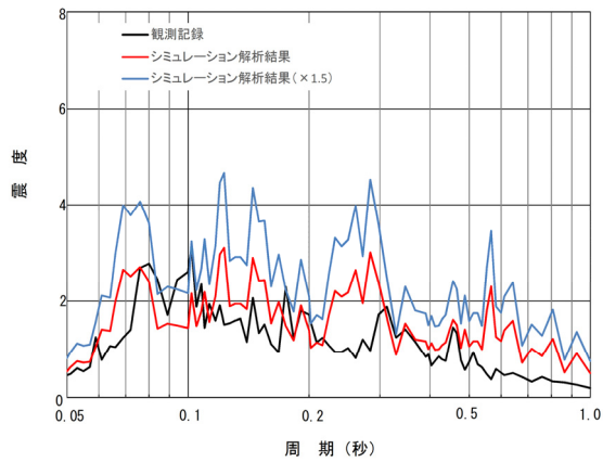
原子炉建屋 EL.29.0m 床応答スペクトル比較(減衰0.5%)
