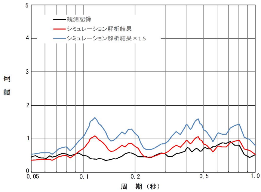
図 4-2 (3/4) 原子炉建屋 EL. 14.0m 床応答スペクトル比較 (減衰 5%)
