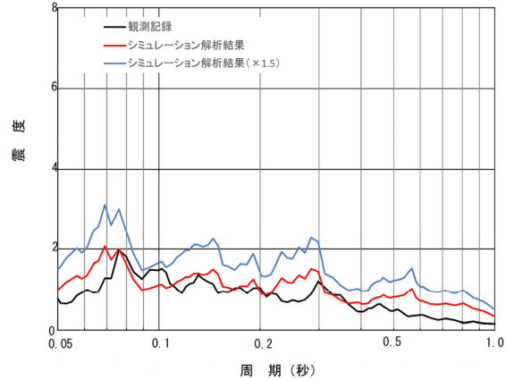
原子炉建屋 EL.46.5m 床応答スペクトル比較(減衰3.0%)
