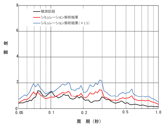
原子炉建屋 EL.29.0m 床応答スペクトル比較(減衰3.0%)
