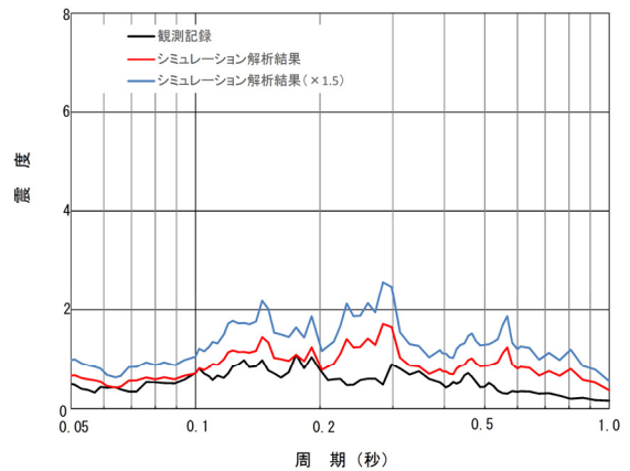
原子炉建屋 EL.14.0m 床応答スペクトル比較(減衰2.0%)
