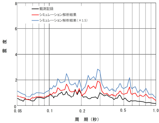
原子炉建屋 EL.14.0m 床応答スペクトル比較(減衰1.5%)
