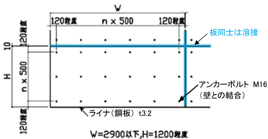
図2 ライナの取付計画
