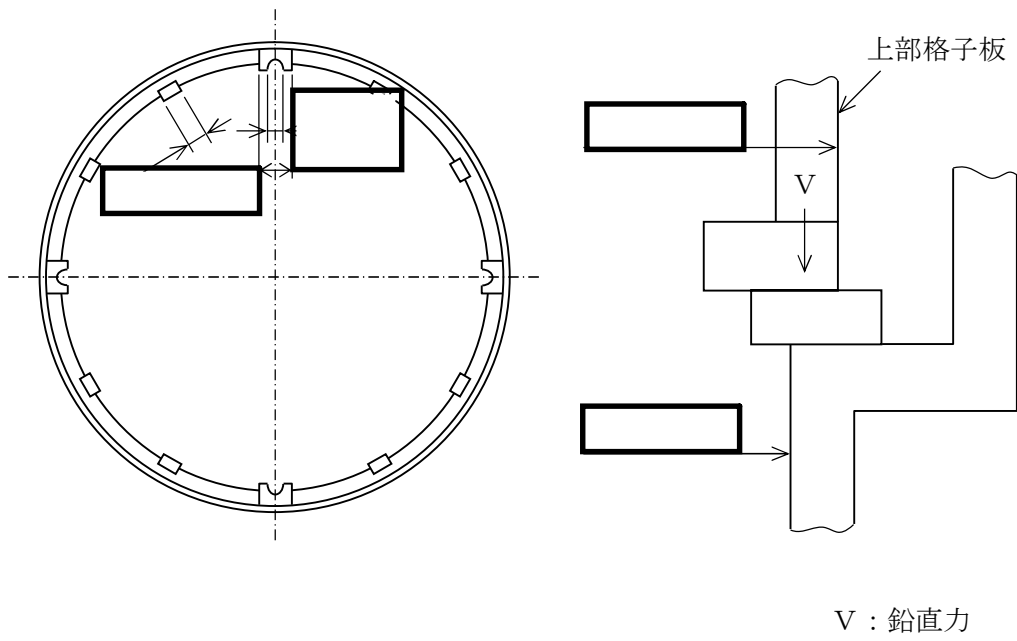
図 5-1(1) 支圧荷重の支持面（上部格子板）（単位：mm）
