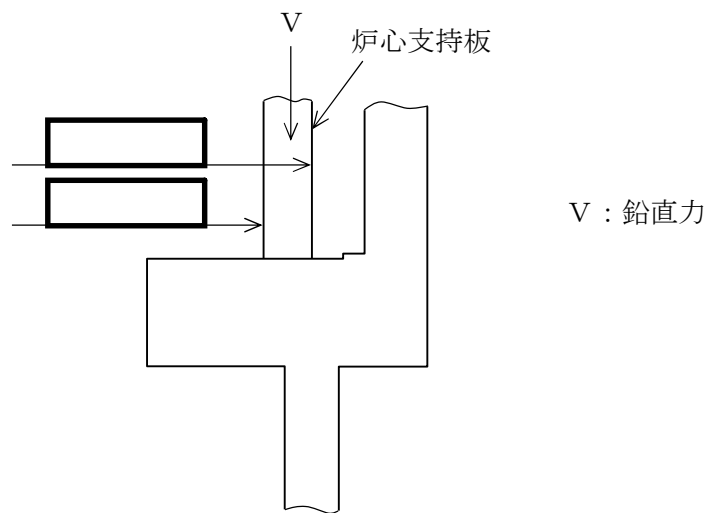
図 5-1(2) 支圧荷重の支持面（炉心支持板）（単位：mm）
