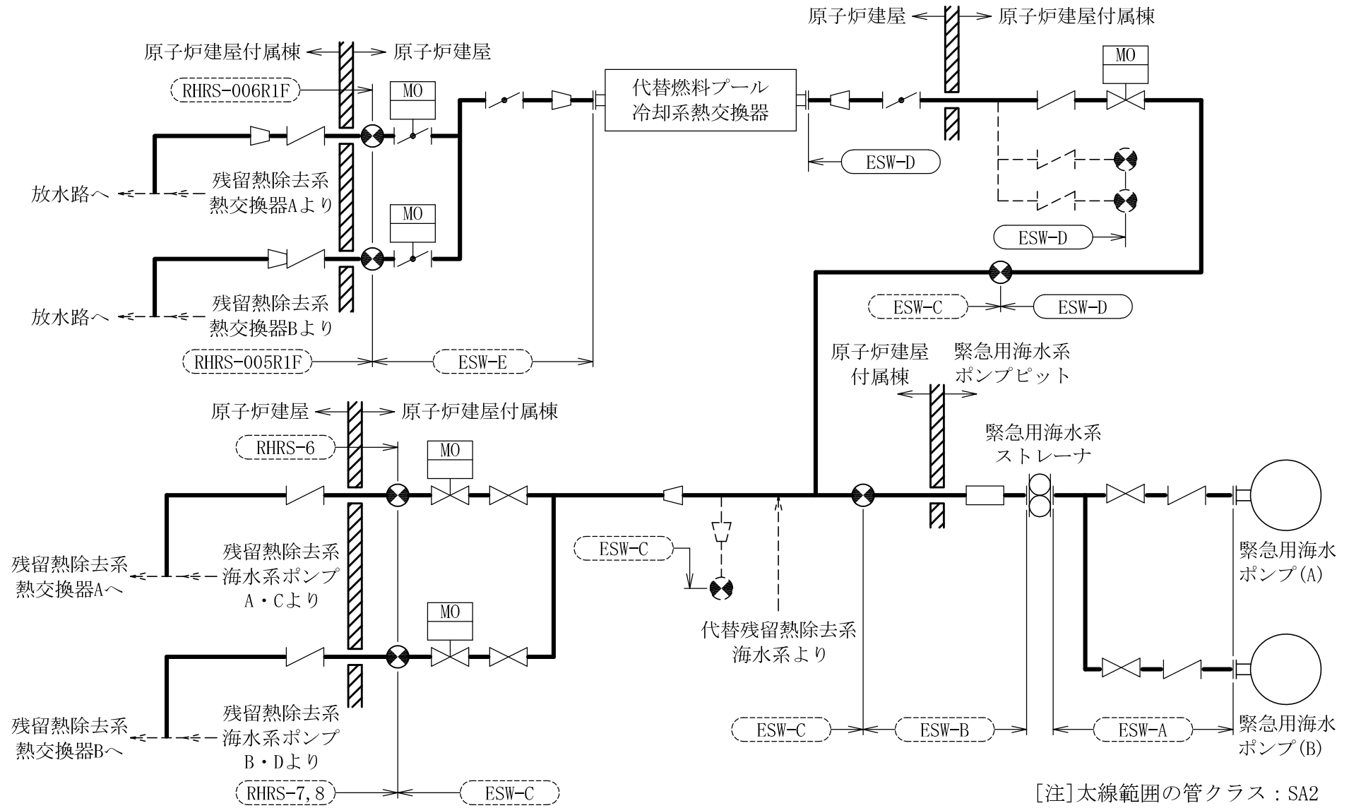
緊急用海水系概略系統図
