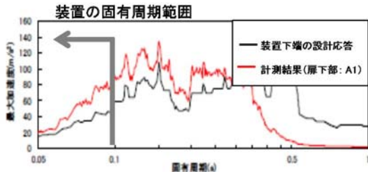
(a) 応答スペクトル(X方向)
