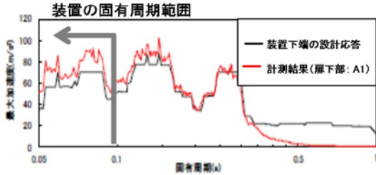
(c) 応答スペクトル(Z方向)
