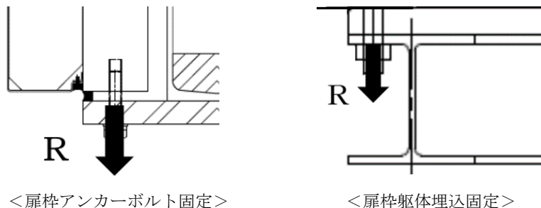
＜扉枠アンカーボルト固定＞ ＜扉枠躯体埋込固定＞ 図3-35 パネル取付部詳細図
