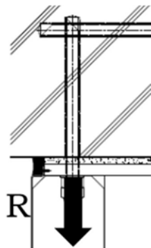
図3-36 アンカーボルト（外部側）詳細図
