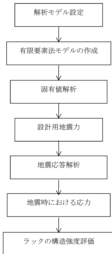
図 2-1 ラックの耐震評価フロー
