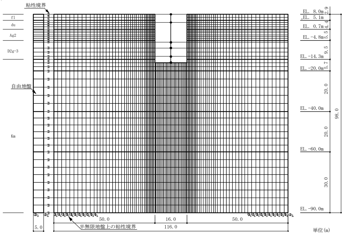
図3-8 地震応答解析モデル (UD方向全体)
