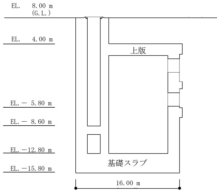
(NS方向, A-A断面)
