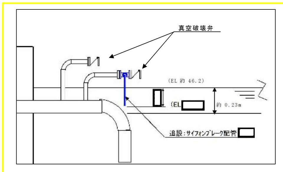
第1-2図 静的サイフォンブレーカ設置概要図
