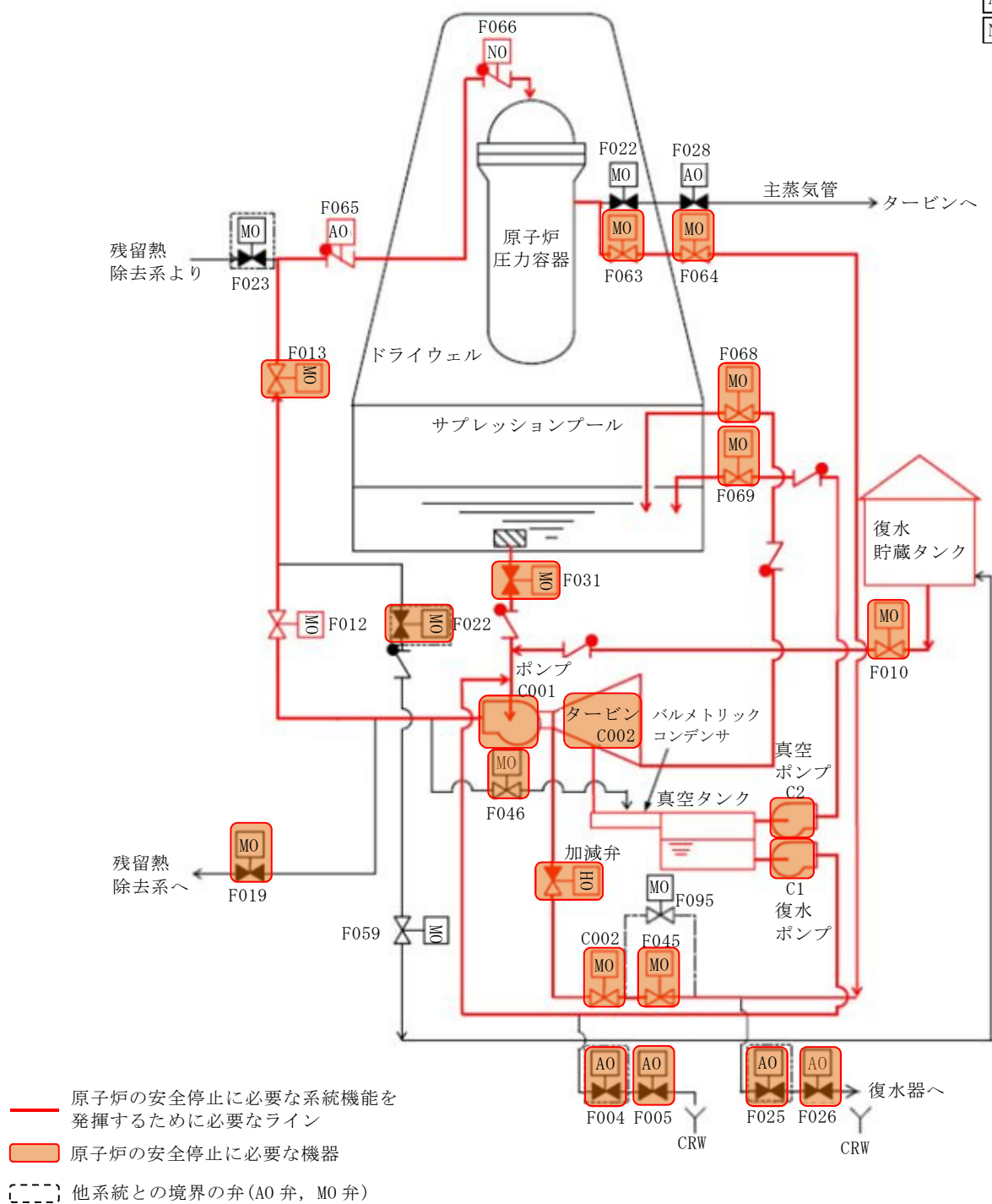
第 4 図 原子炉隔離時冷却系
