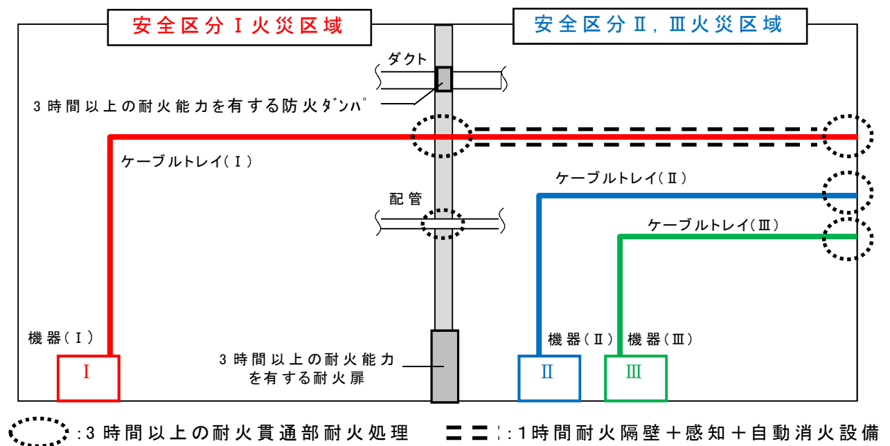
第2図 火災防護対象ケーブルの系統分離概要
