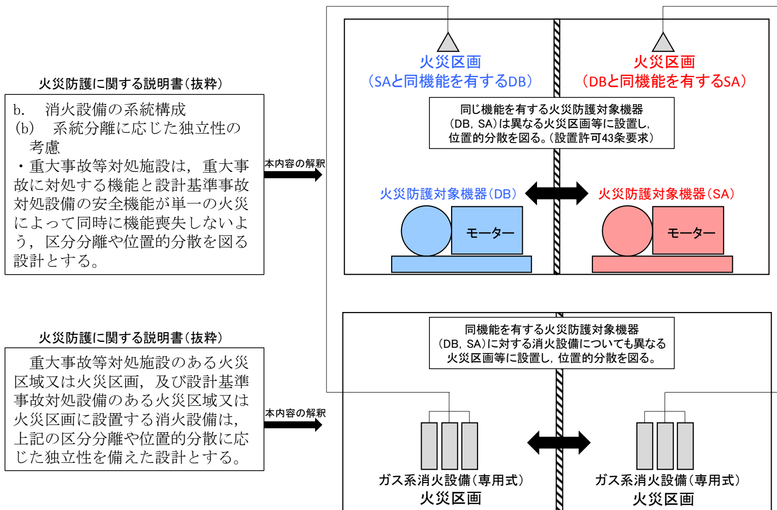
第1図 重大事故等対処施設及び設計基準対処設備の消火設備の 位置的分散に応じた独立性を備えた設計について (消火設備 (専用式の場合))
