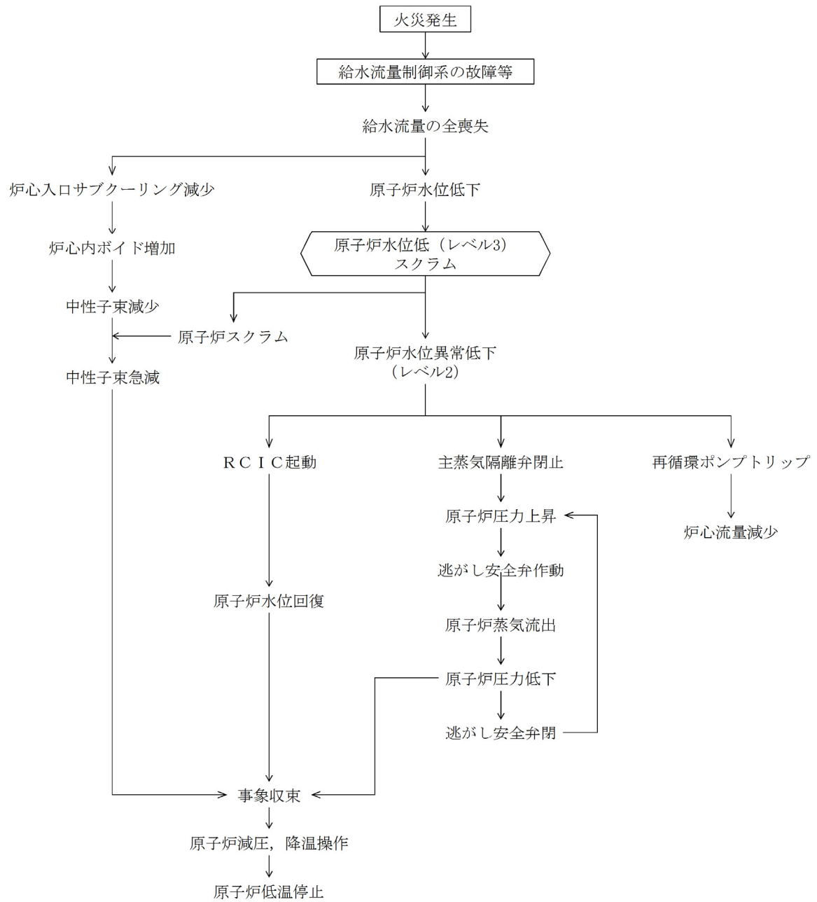
第 14 図 「給水流量の全喪失」の事象過程
