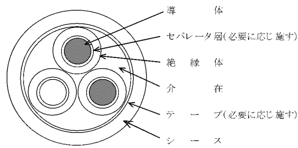
600V CV 構造
