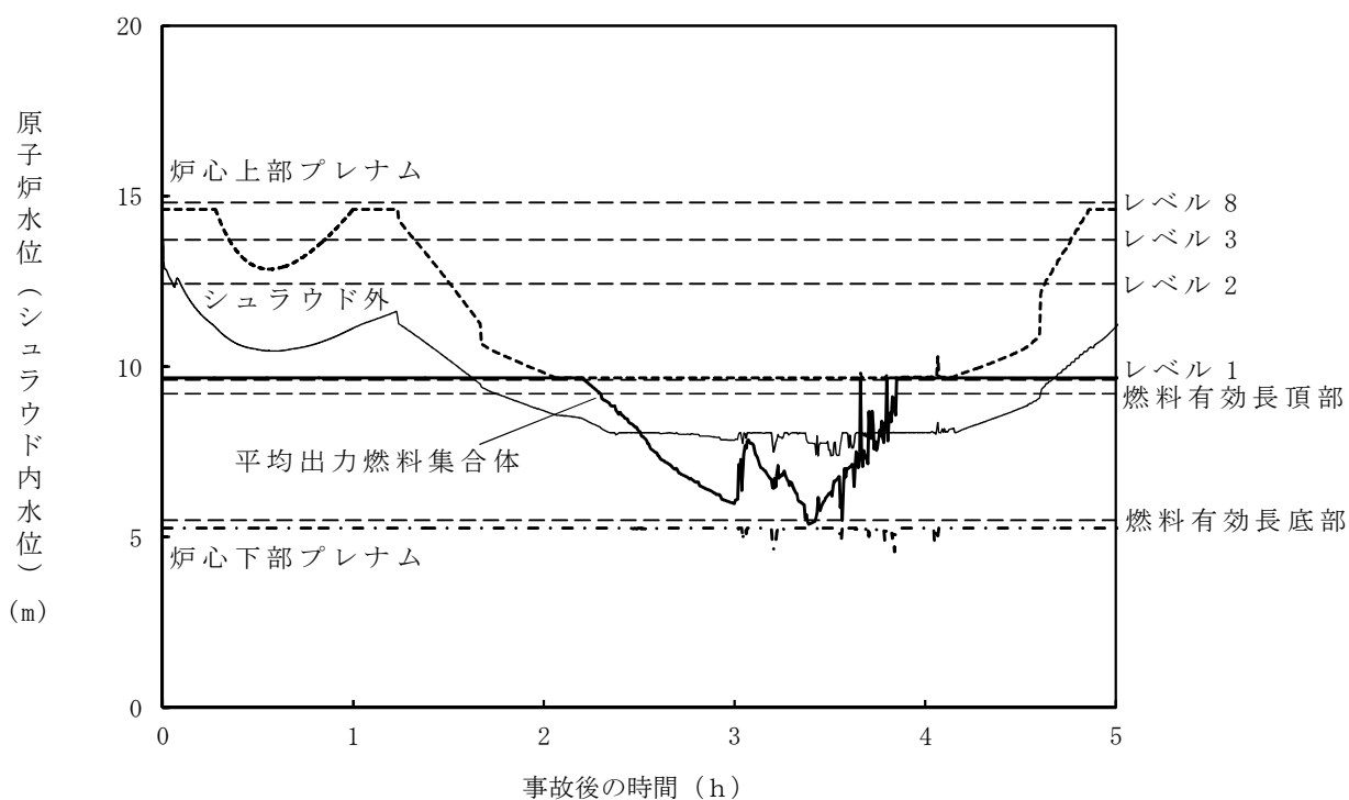
第 2 図 原子炉水位 (シュラウド内外水位) の推移
