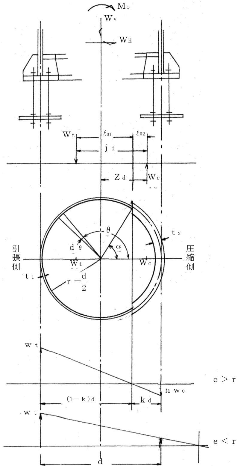
図 5-1 アンカーボルトの等価円筒及び荷重分布
