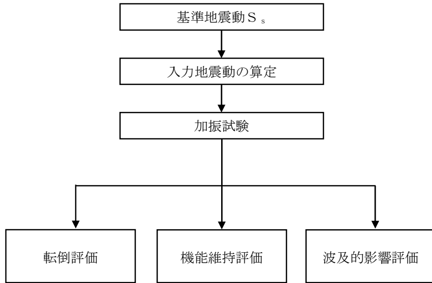
図 2-5 その他設備の評価フロー
