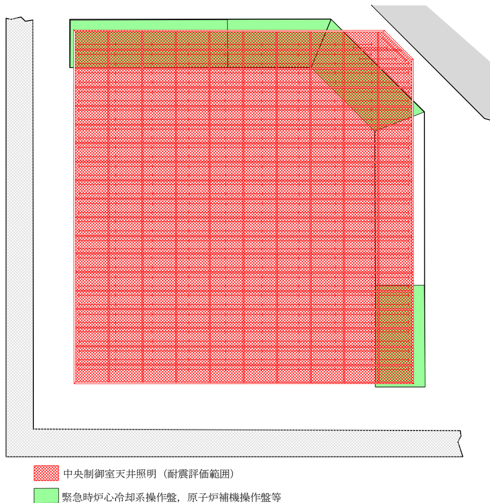
図2-1 中央制御室天井照明と緊急時炉心冷却系操作盤，原子炉補機操作盤等の位置関係図
