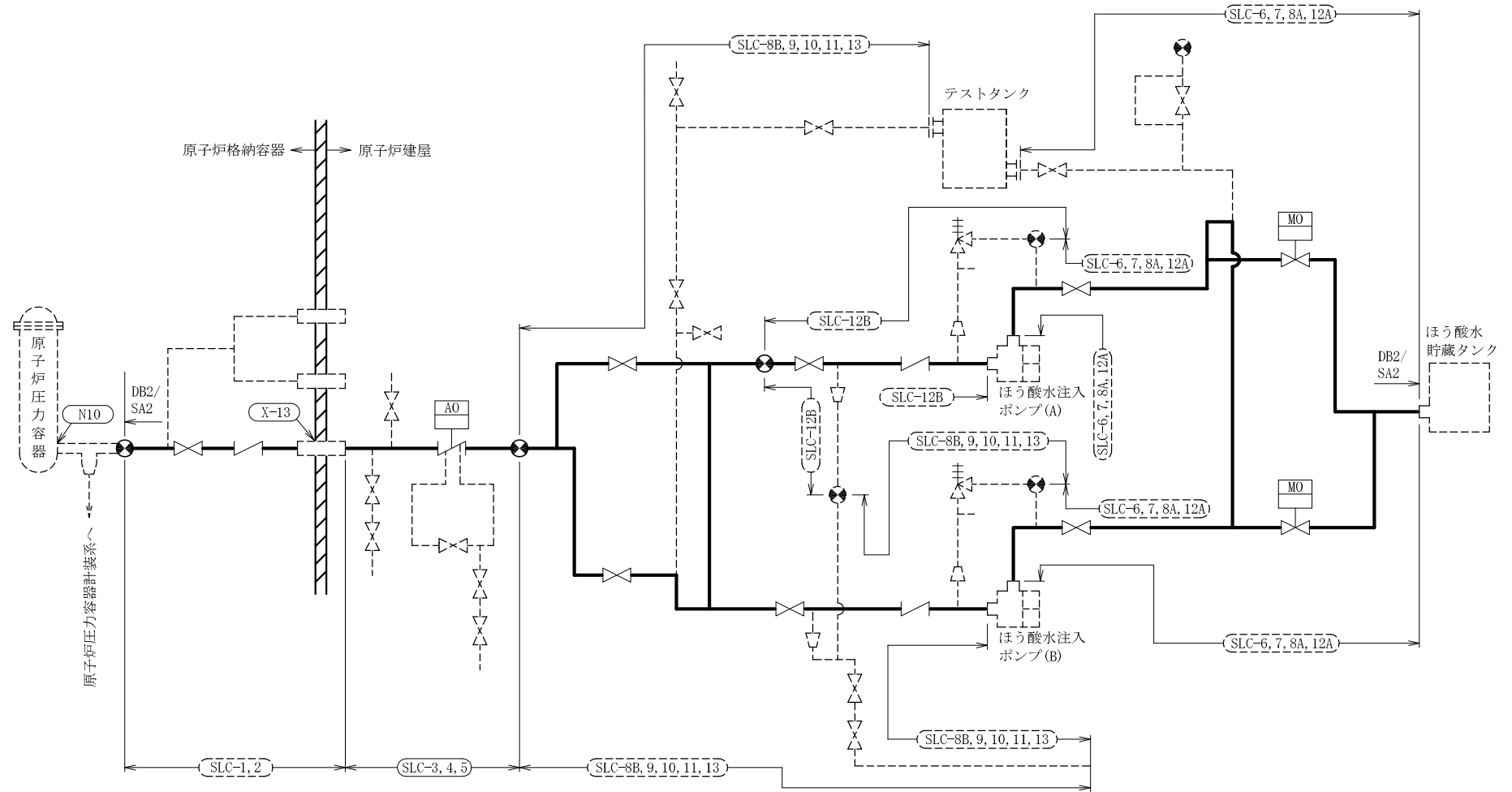
ほう酸水注入系概略系統図
