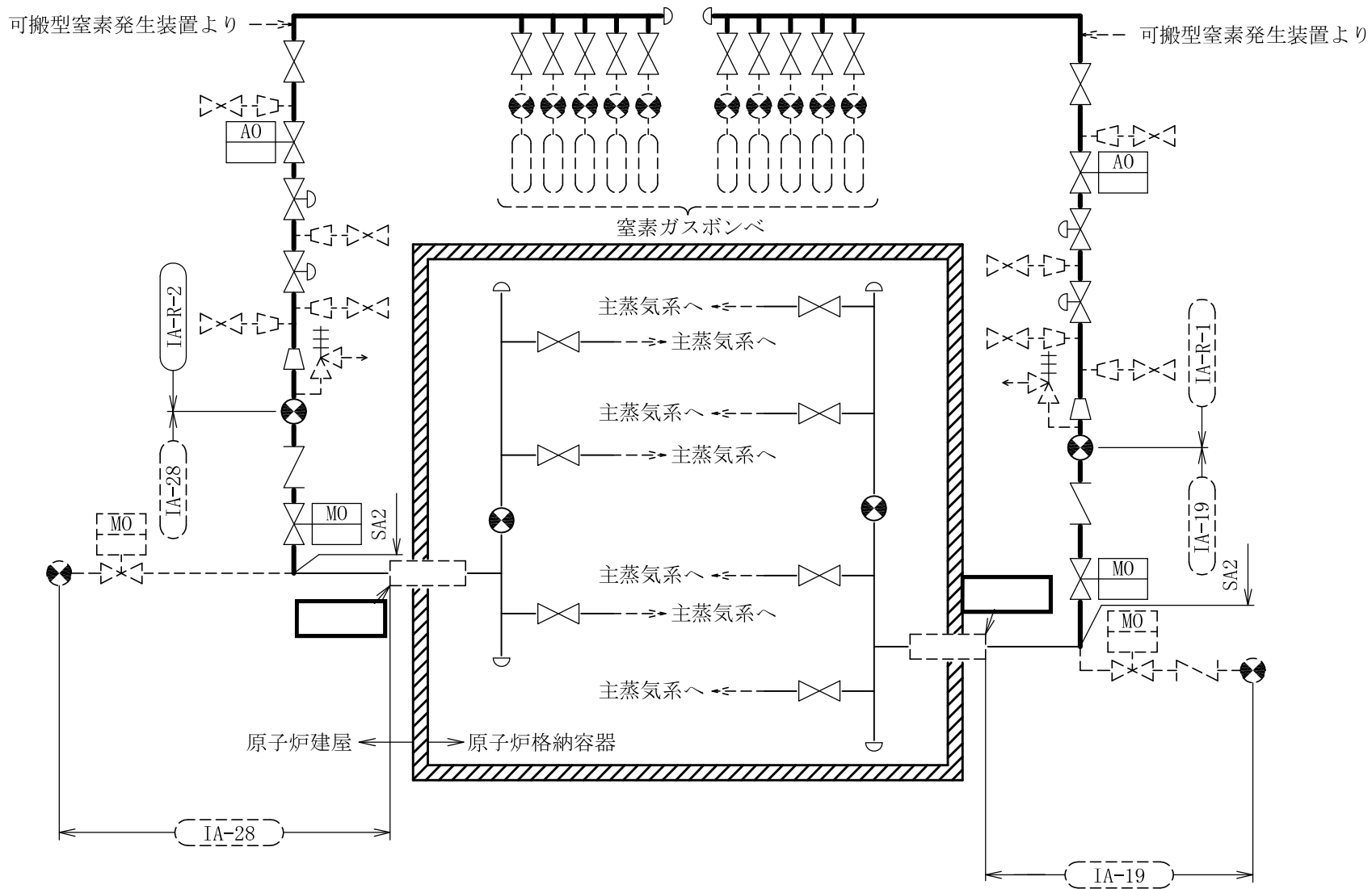
非常用窒素供給系概略系統図
