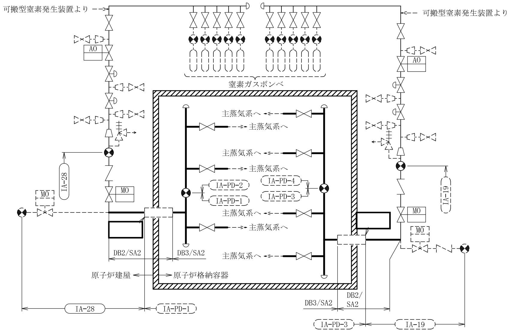
窒素供給系概略系統図
