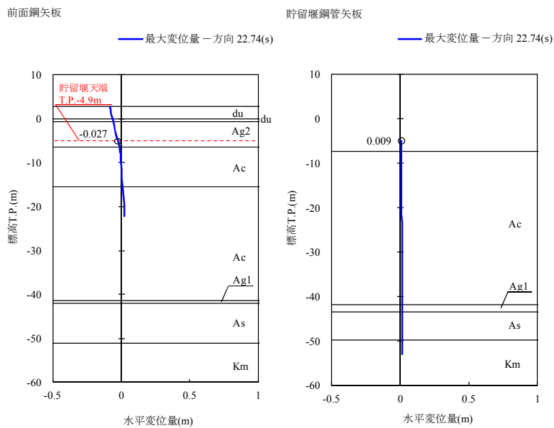
図 5.2-4 (4) 相对変位量 ( S_s - D1 [H-, V-]) (相对変位量 \delta y (-)) (EW-1 検討ケース⑤: 原地盤において非液状化の条件を仮定した解析ケース)
