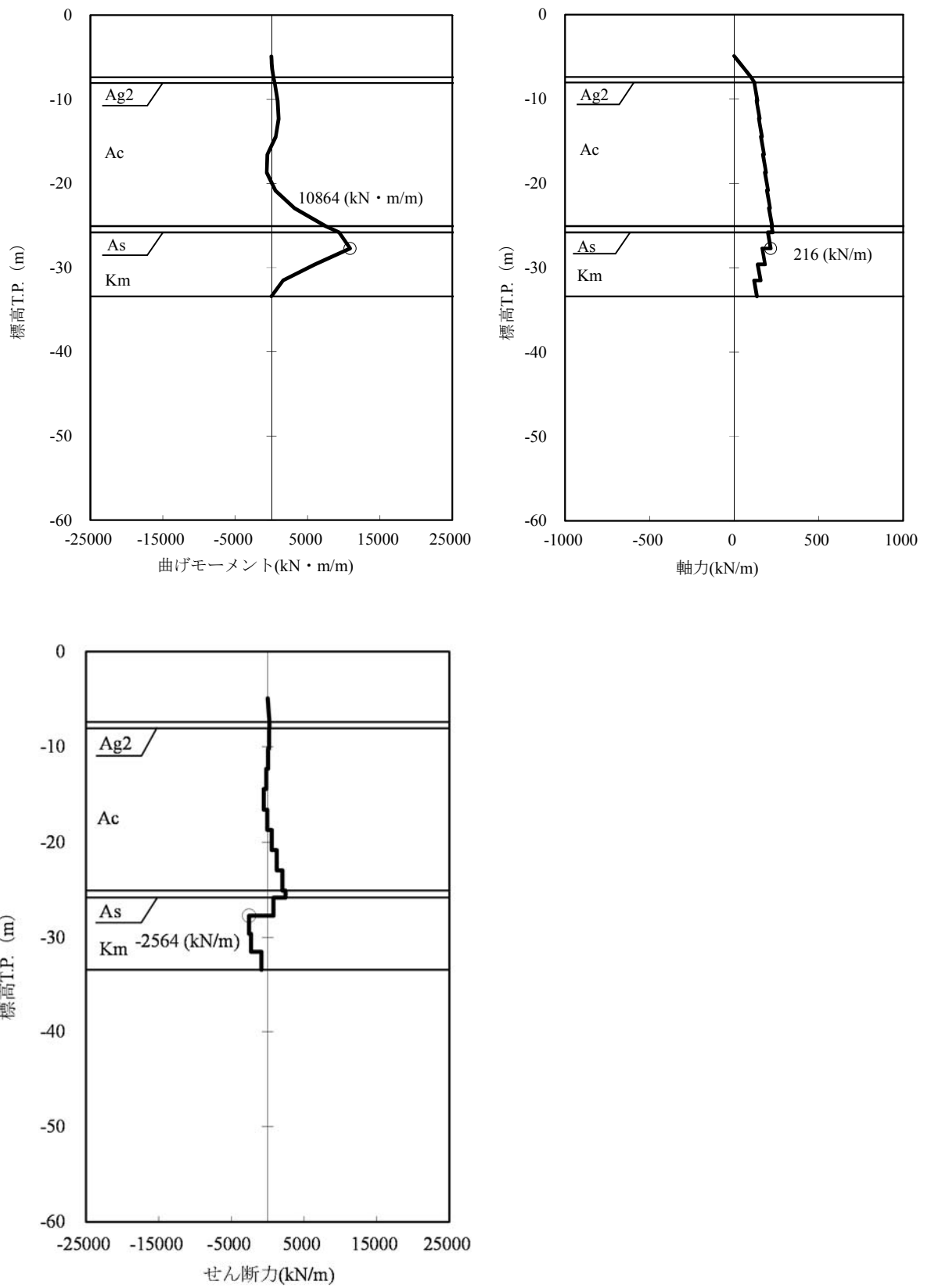
図 4.2-5 (3) 断面 3 の発生断面力 (重畳時, 地盤ばね 5)
