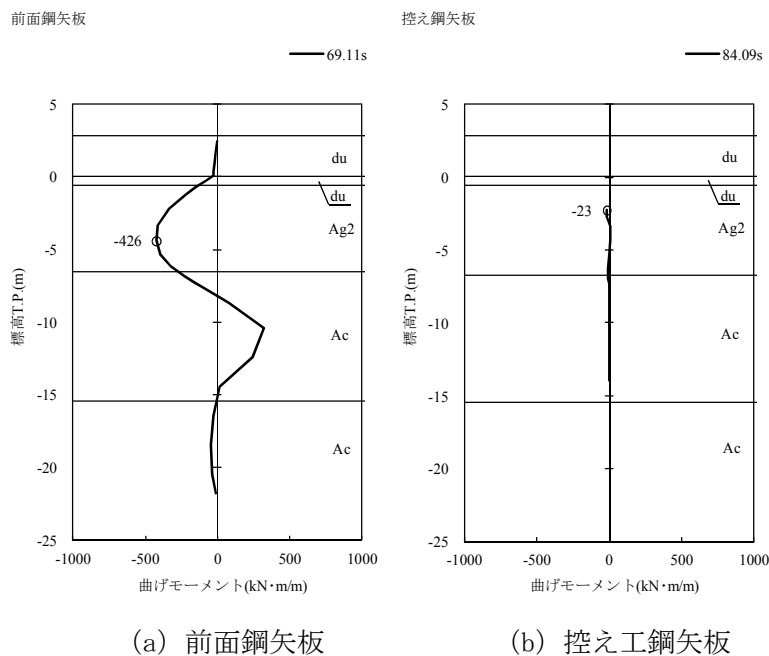
図 5.1-1 (10) 最も厳しい照査値となる時刻の断面力 ( S_s - 2 2 )
