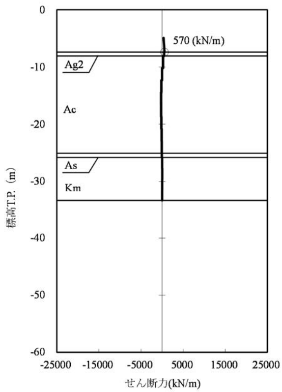
図 4.1-3 (1) 断面3の発生断面力(津波時, 地盤ばね1)
