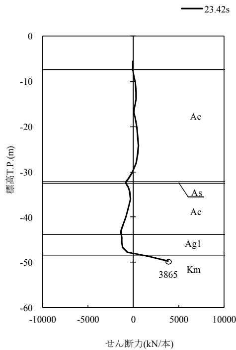
図 5.1-2 (4) 地震時断面力 (S s -D1 [H-,V-])
