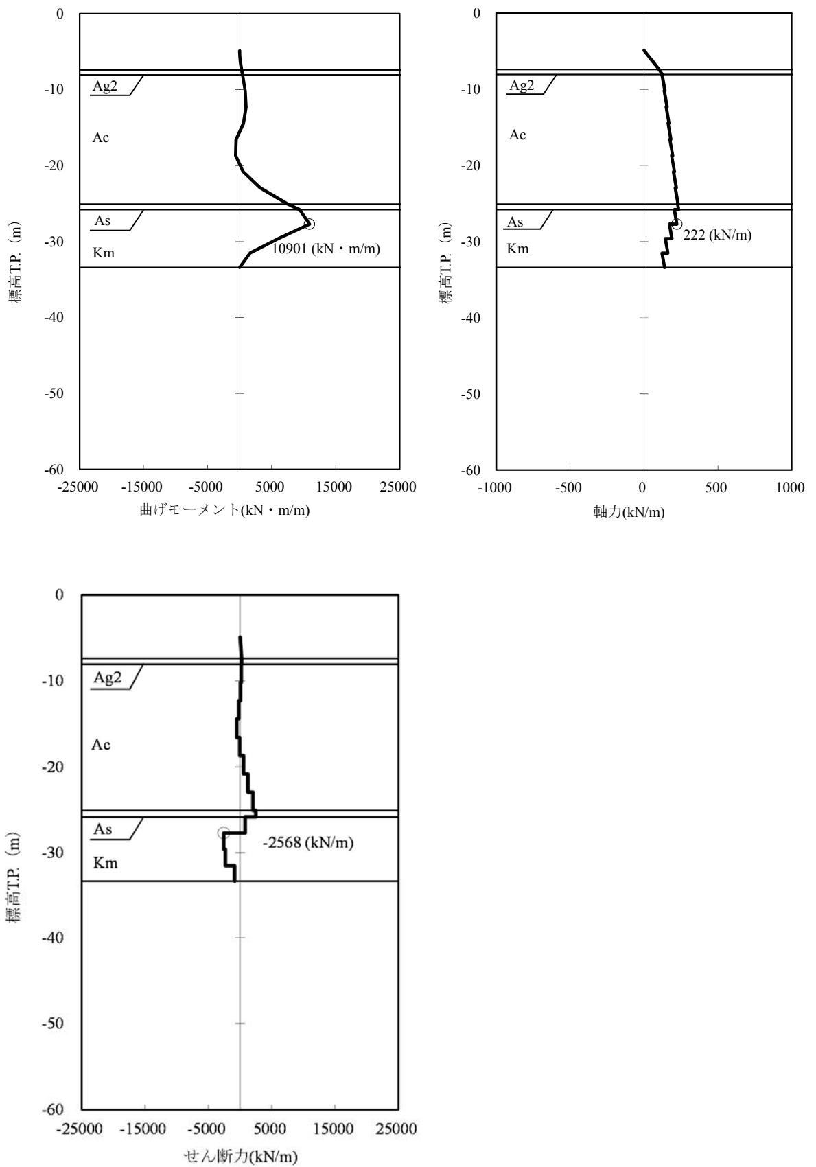
図 4.2-5 (2) 断面 3 の発生断面力 (重畳時, 地盤ばね 4)
