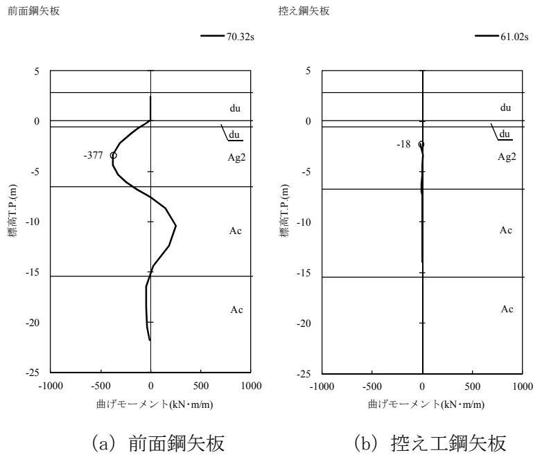
図 5.1-1 (9) 最も厳しい照査値となる時刻の断面力 ( S_s - 2 1 )
