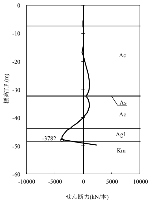
図 5.1-2 (3) 地震時断面力 ( S_s - D1 [H-, V+])
