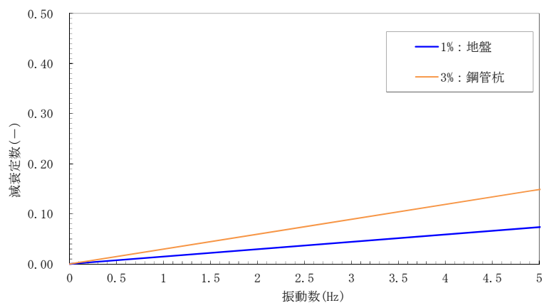
図 1-2 (4) 設定した Rayleigh 減衰
