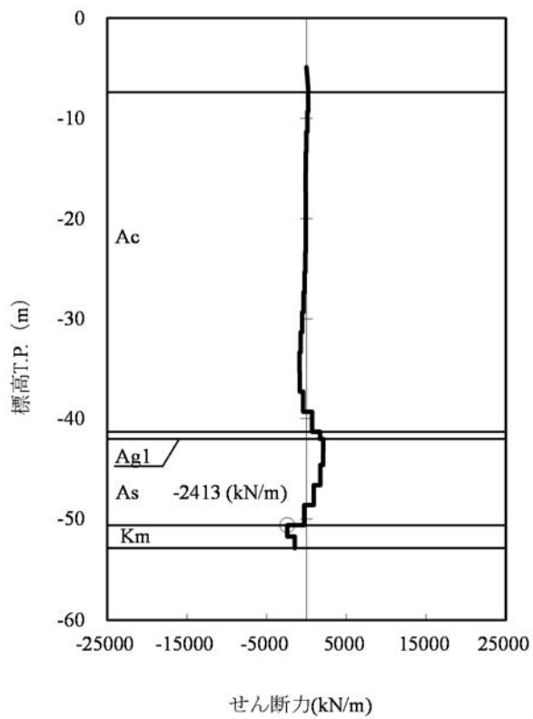
図 4.2-6 (2) 断面 4 の発生断面力 (重畳, 地盤ばね 4)
