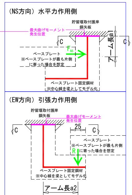
図 3.5-12 照査モデル図 (止水ゴム取付部鋼材 ベースプレート固定鋼材)
