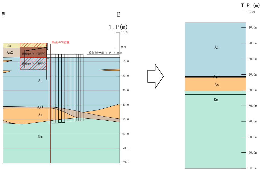
図 3.2-3 (4) 地層構成 (断面 4)
