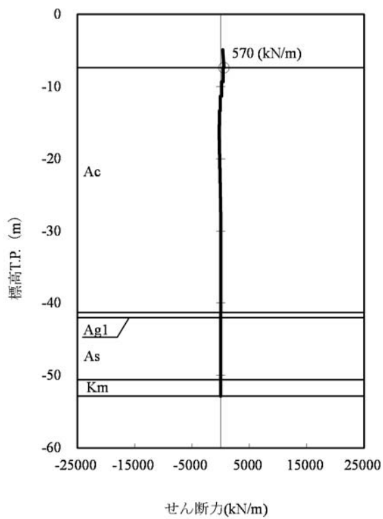
図 4.1-4 (1) 断面 4 の発生断面力 (津波時, 地盤ばね 1)
