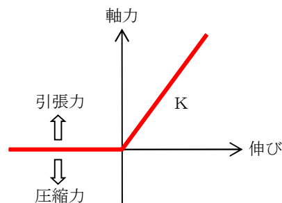
図 3.5-9 タイ材のモデル化に用いる非線形ばね要素の考え方
