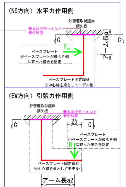
図 4.4-11 照査モデル図 (止水ゴム取付部鋼材 ベースプレート固定鋼材)
