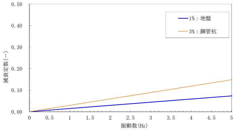
図 1-2 (2) 設定した Rayleigh 減衰
