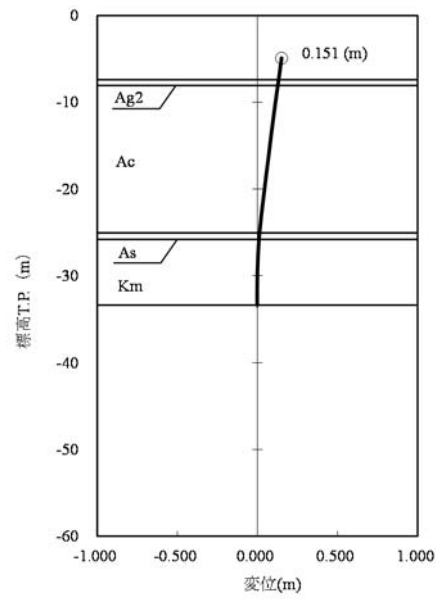
図 4.2-10 相対水平変位量 \delta x (+) (重畳時 最大変位量)
