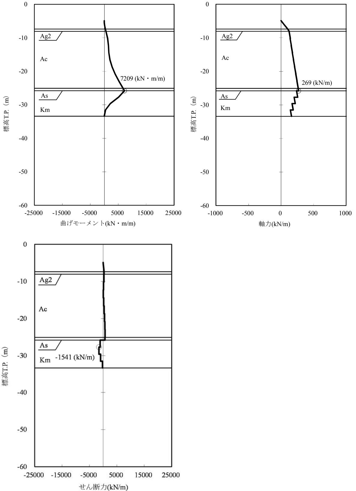
図 4.2-5 (1) 断面 3 の発生断面力（重畳時，地盤ばね 3）
