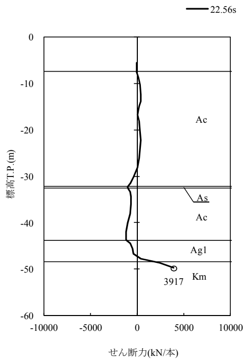
図 5.1-2 (14) 地震時断面力 ( S_s - D1 [H+, V+])
