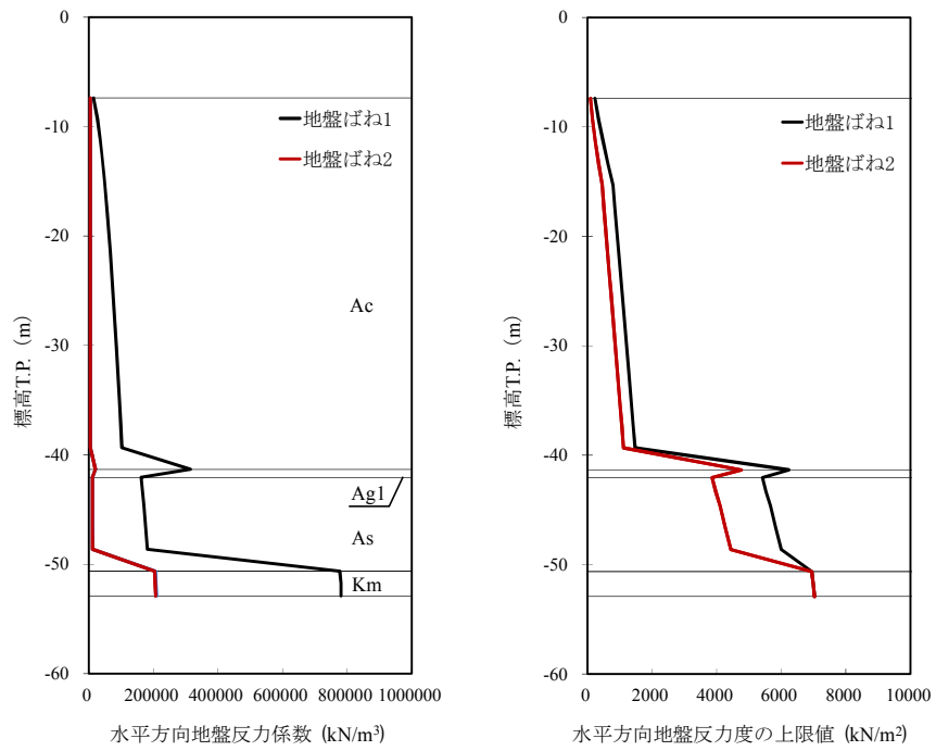
図 4.1-2 (3) 地盤ばね 1 及び地盤ばね 2 の比較 (断面 4)
