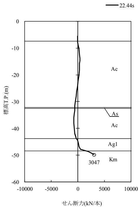
図 5.1-2 (17) 地震時断面力 ( S_s - D1 [H+, V+] )
