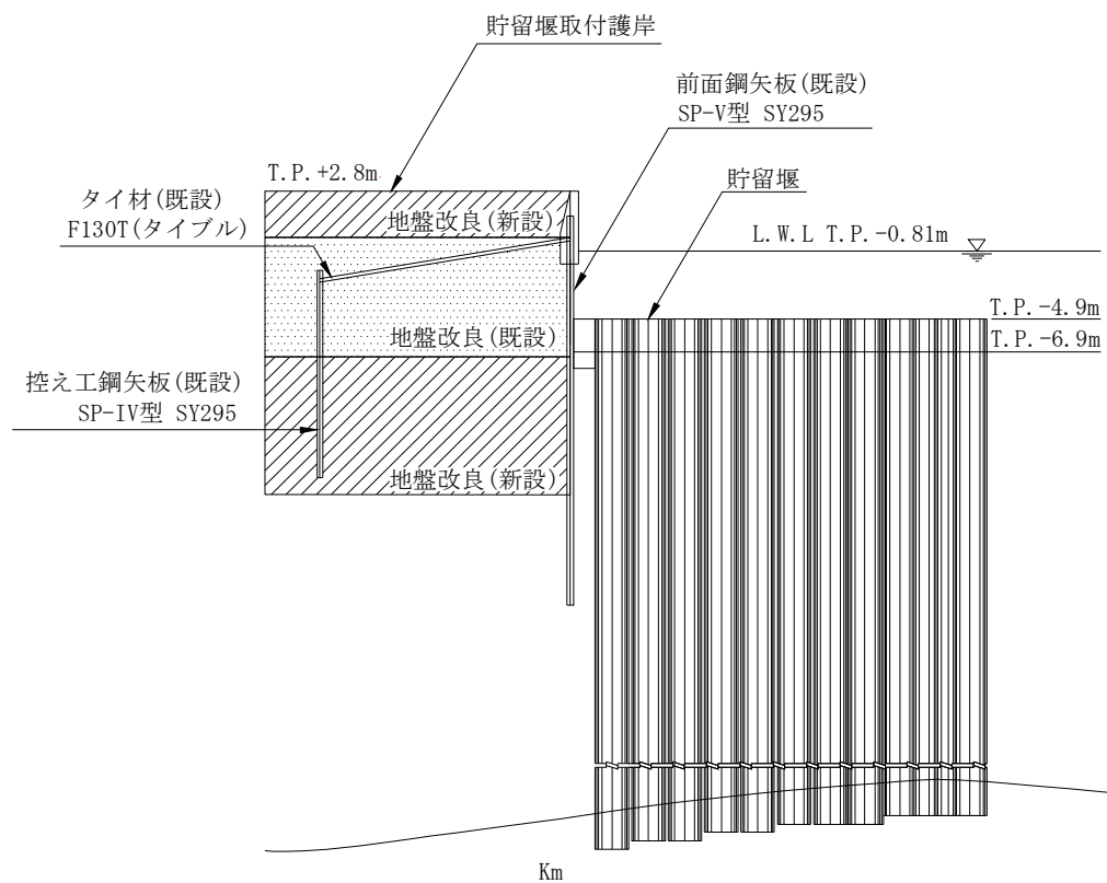
図 2. 2-2 貯留堰取付護岸の標準断面図 (A-A 断面)
