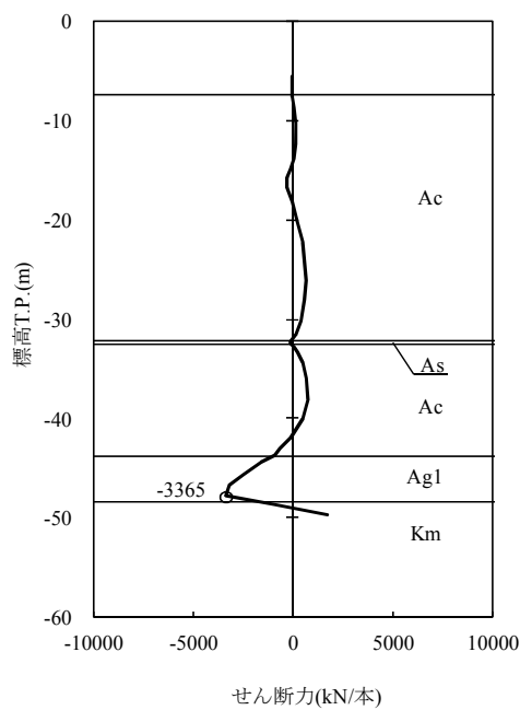
図 5.1-2 (8) 地震時断面力 ( S_s - 1.4 )
