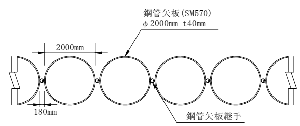
図 2.2-3 貯留堰の標準図
