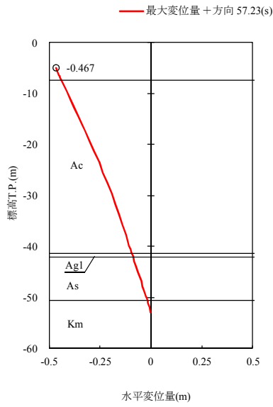
貯留堰鋼管矢板(北側)
