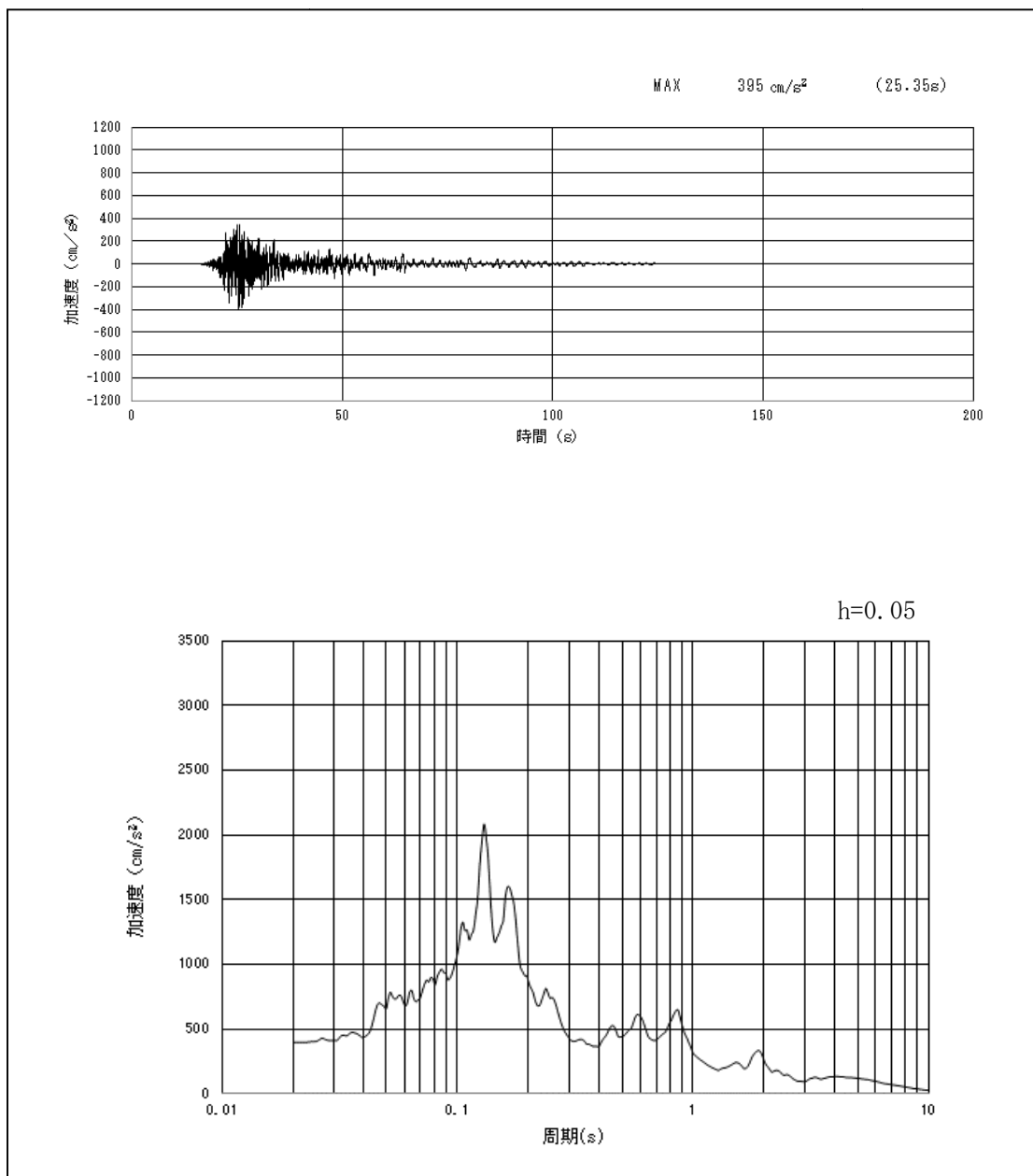
第2-8図(3) 南保管場所の入力地震動の加速度時刻歴波形及び加速度応答スペクトル (東西方向: S_s - 11 )
