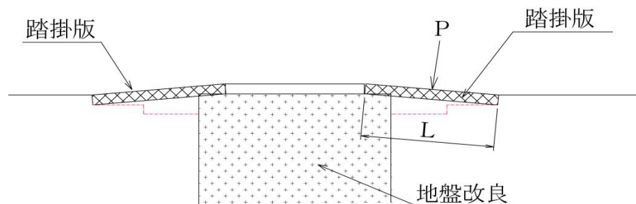
第9-15図 踏掛版断面図
