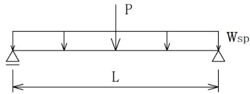
第9-14図 荷重図
