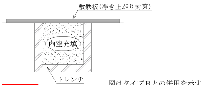
タイプC (内空充填)
