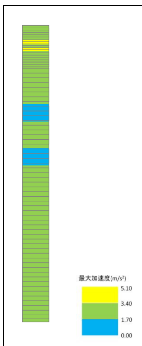
最大水平加速度分布 第2-10図(6)
