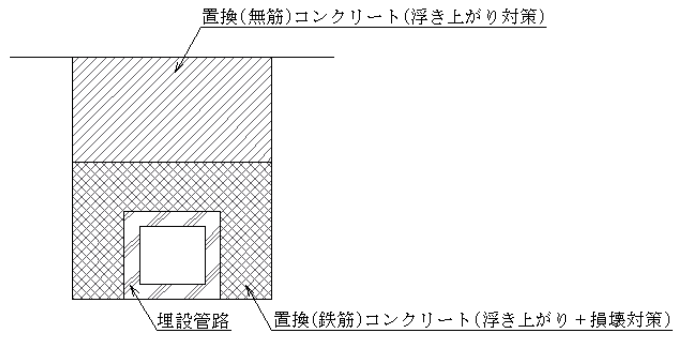
タイプA (置換コンクリート)
