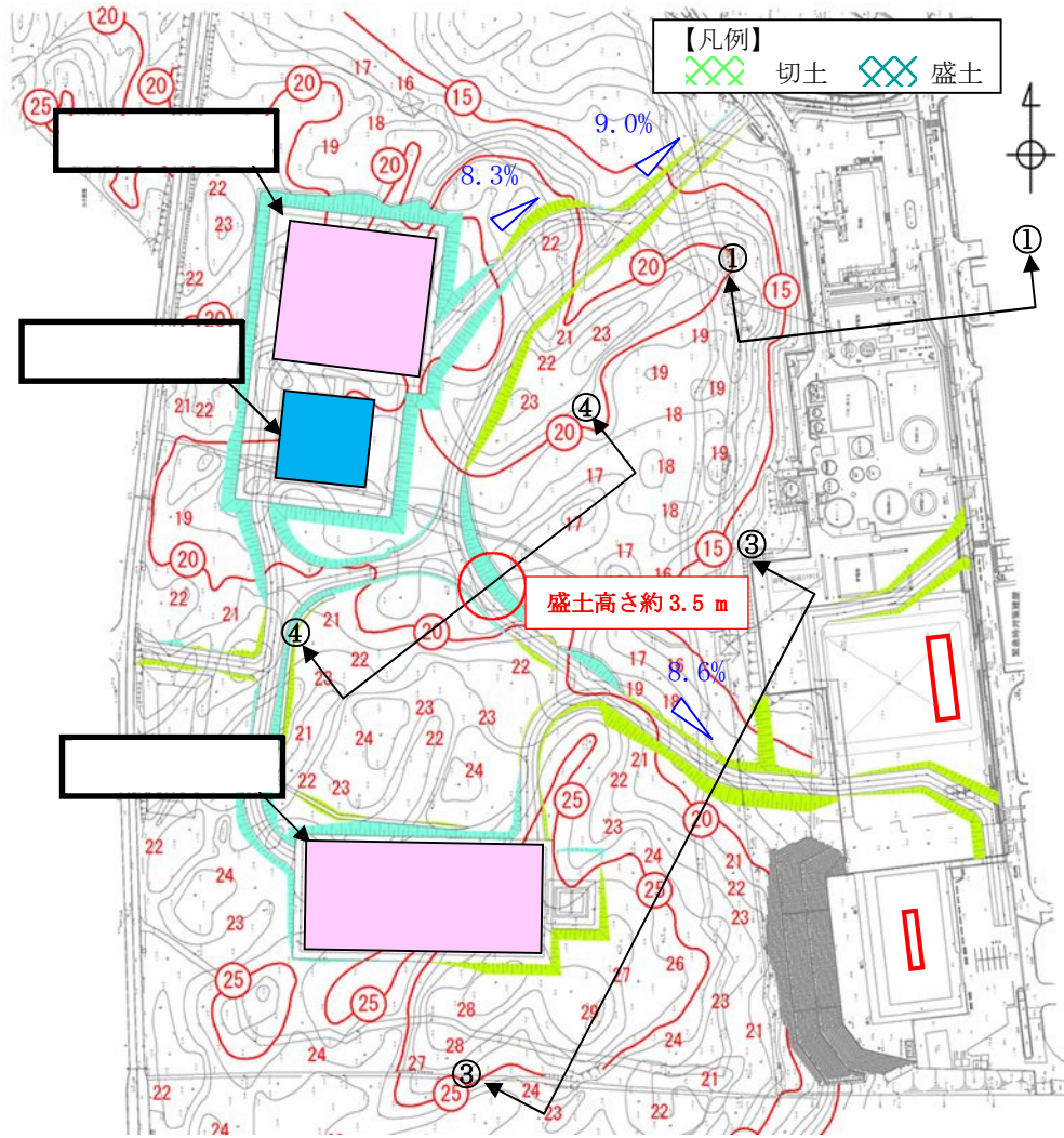
第 3-4 図 アクセスルート周辺の斜面の崩壊及び道路面のすべりに対する影響評価断面位置図 (2/2)
