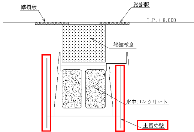
タイプD (踏掛版)
