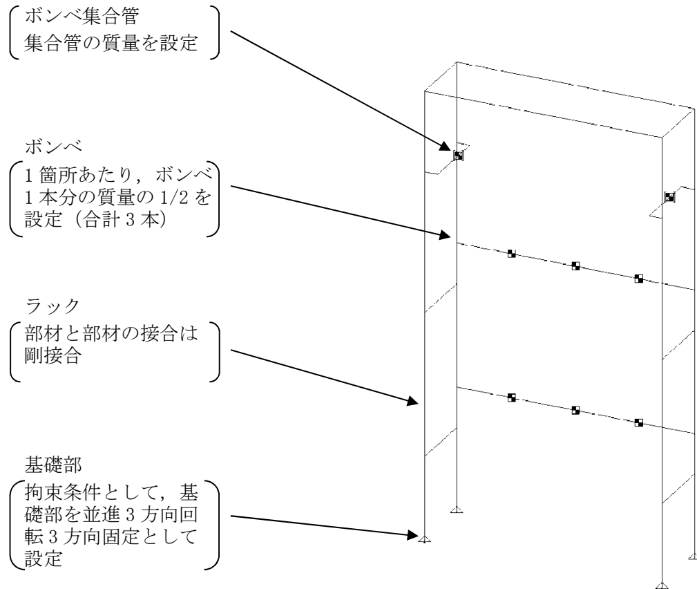
図3-1 解析モデル
