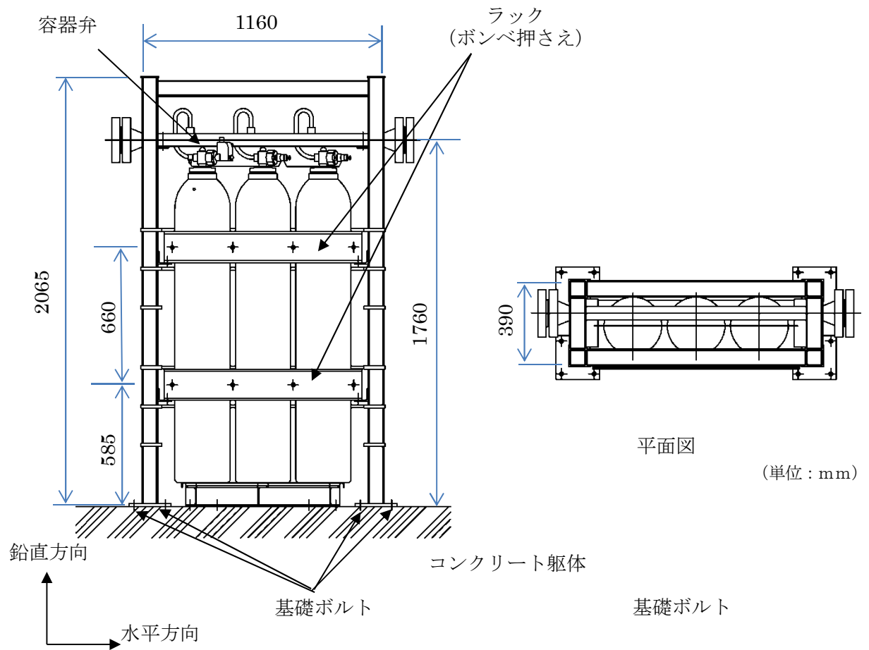
図 2-1 ハロンポンベ設備 外観図
