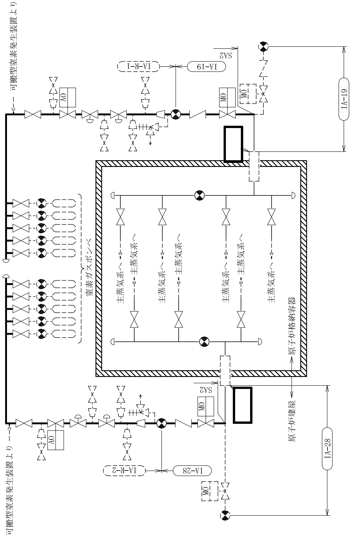
非常用窒素供給系概略系統図
