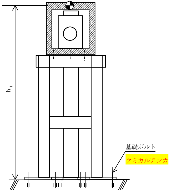
正面 (左右方向)
