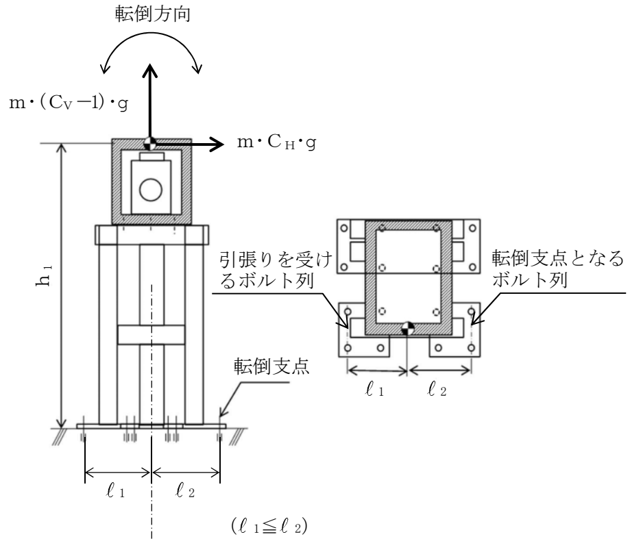
図5-1(1) 計算モデル (直立形 正面方向転倒-2 ( 1 - C_v < 0 )の場合)
