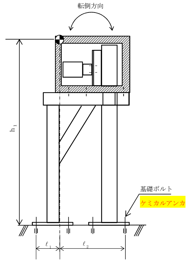
側面 (前後方向)
