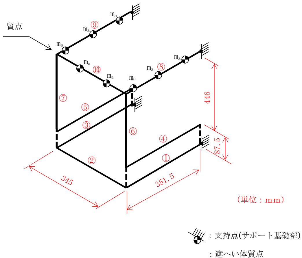
図 2-2 低圧代替注水系原子炉注水流量 （可搬ライン用）遮へい体 解析モデル
