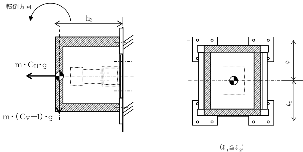
図 2-3(1) 低圧代替注水系原子炉注水流量（可搬ライン用）遮へい体 計算モデル (壁掛形 正面方向転倒の場合)
