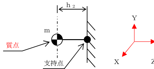
図 1-1 固有周期の計算モデル
