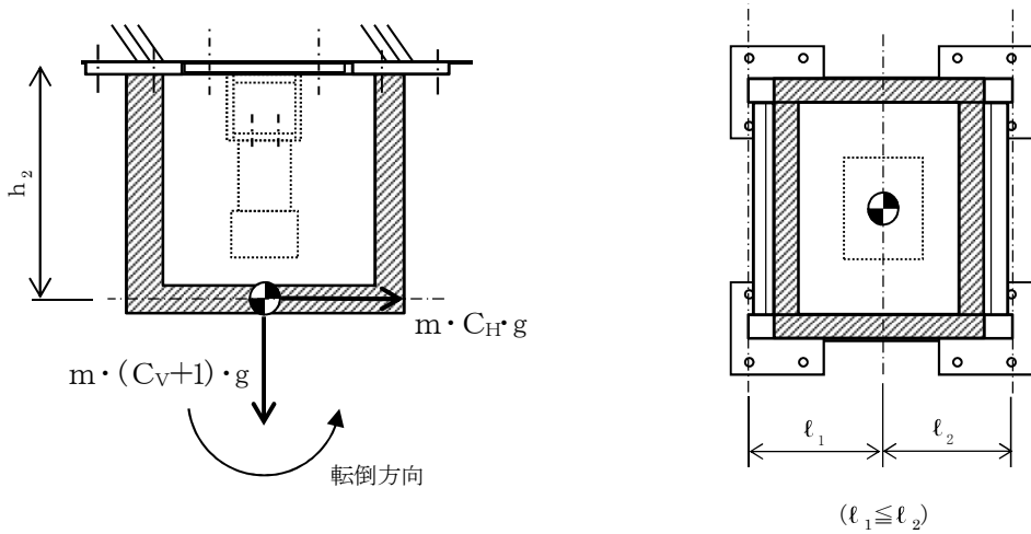
図 2-3(1) 低圧代替注水系原子炉注水流量（可搬ライン用）遮へい体 計算モデル (壁掛形 正面方向転倒の場合)
