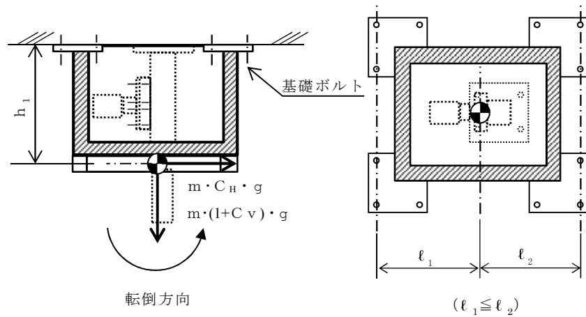
図4-3(2) サプレッション・プール水位 (LT-26-79.60用遮へい体) 計算モデル (壁掛形 側面方向転倒の場合)
