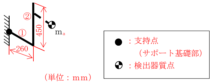
図 1-2 サプレッション・プール水位 (LT-26-79.5A) 解析モデル
