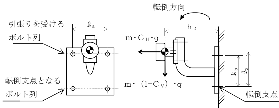
図2-3(2) サプレッション・プール水位 (LT-26-79.5B) 計算モデル (壁掛形 側面方向転倒の場合)
