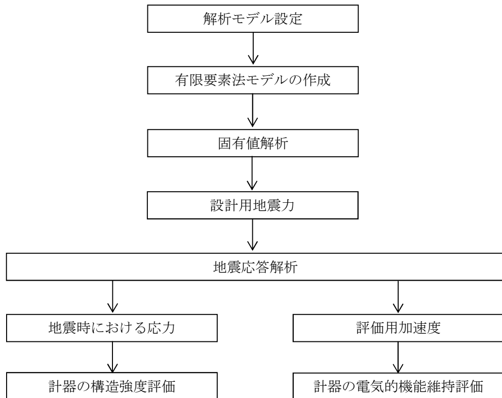
図 1-1 サプレッション・プール水位 (LT-26-79.5A) の耐震評価フロー
