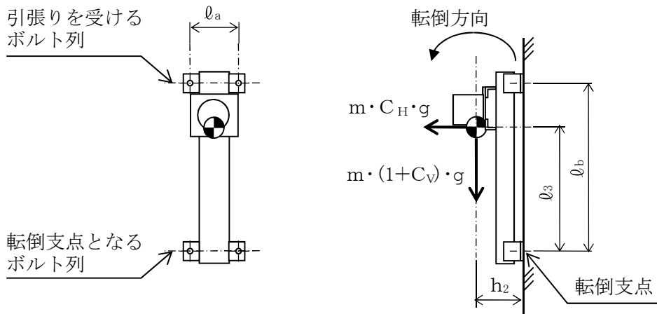
図3-5(2) LT-26-79.60 計算モデル (壁掛形 側面方向転倒の場合)
