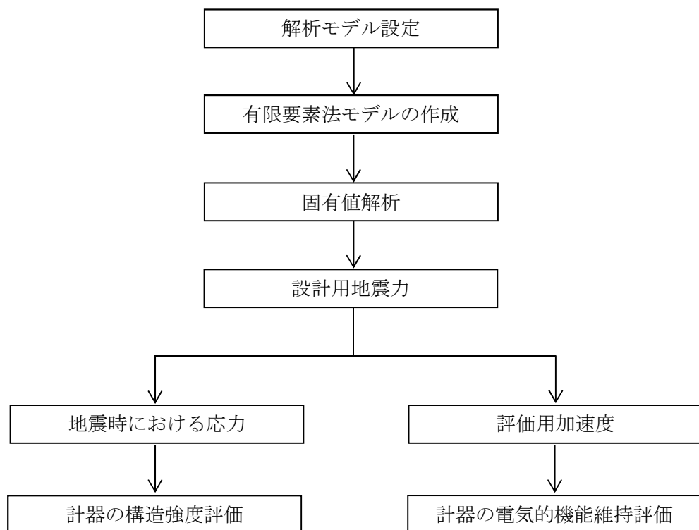
図 2-1 サプレッション・プール水位 (LT-26-79.5B) の耐震評価フロー
