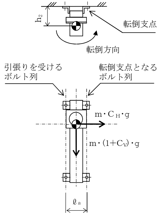
図3-5(1) LT-26-79.60 計算モデル (壁掛形 正面方向転倒の場合)
