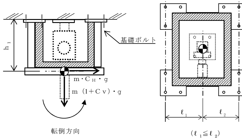
図4-3(1) サプレッション・プール水位 (LT-26-79.60用遮へい体) 計算モデル (壁掛形 正面方向転倒の場合)
