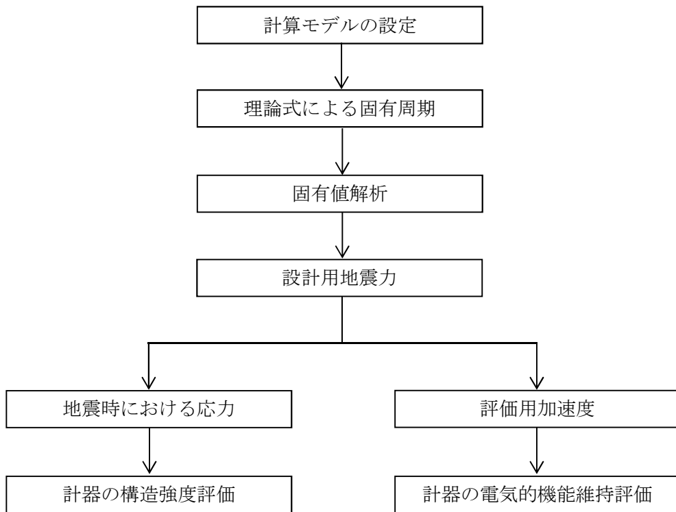
図 3-1 サプレッション・プール水位 (LT-26-79.60) の耐震評価フロー
