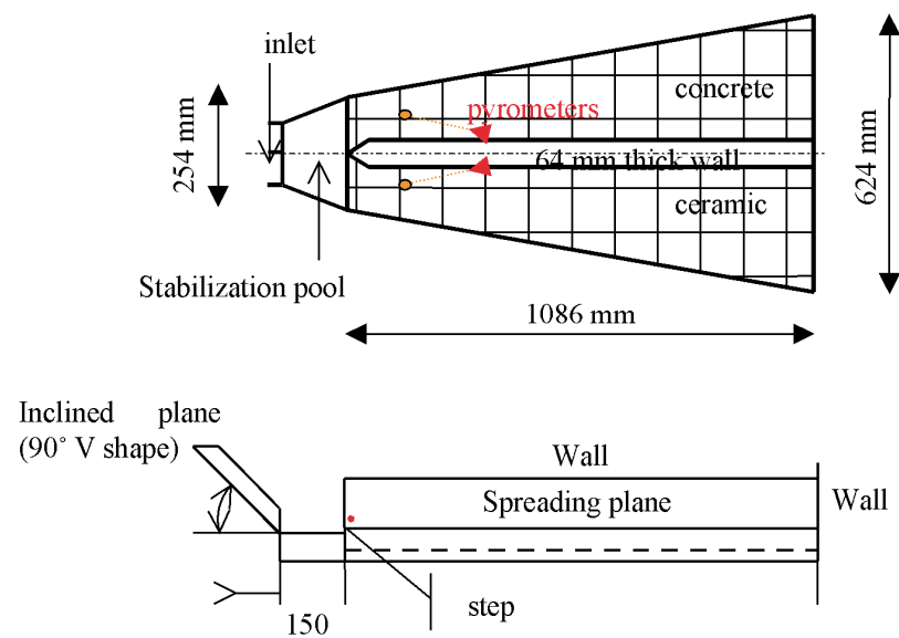
図 5 VULCANO 実験装置の概要図 [6]
