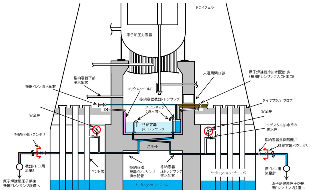
ペDESTAL概要図(断面図)
