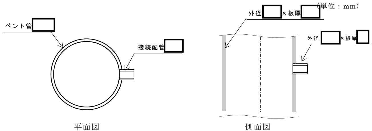
図1 ベント管と排水配管の取り付け形状と主要寸法
