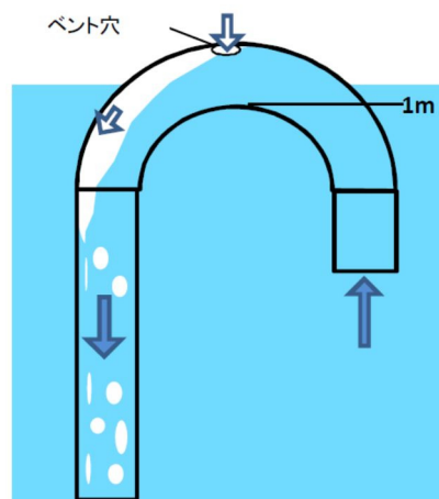
図10-5 水位がベント穴に達した時の状況（模式図）
