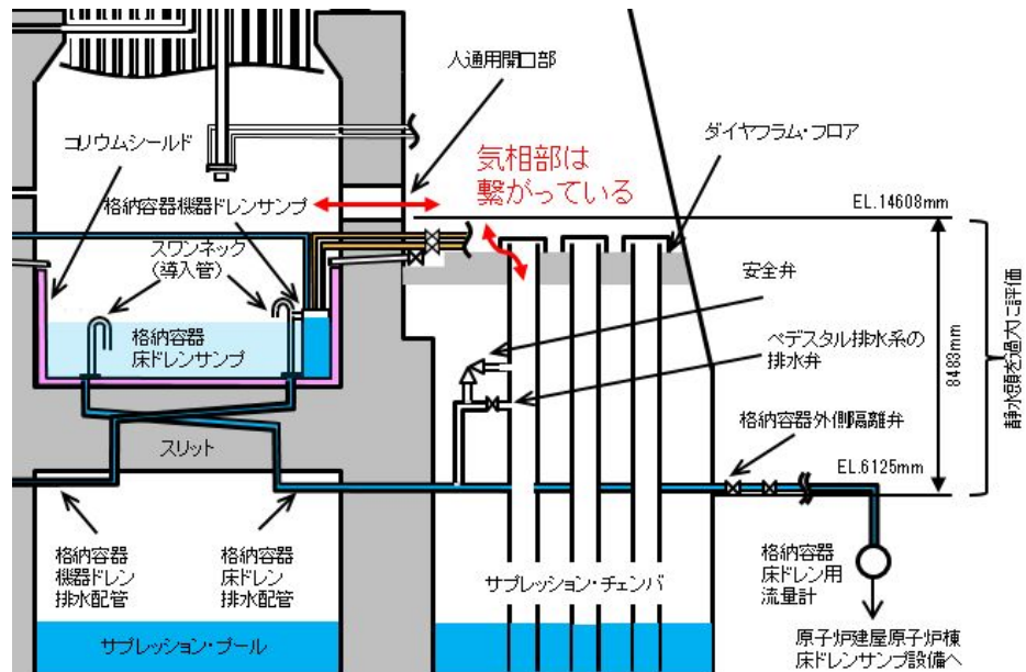
ペDESTAL概要図(断面図)
