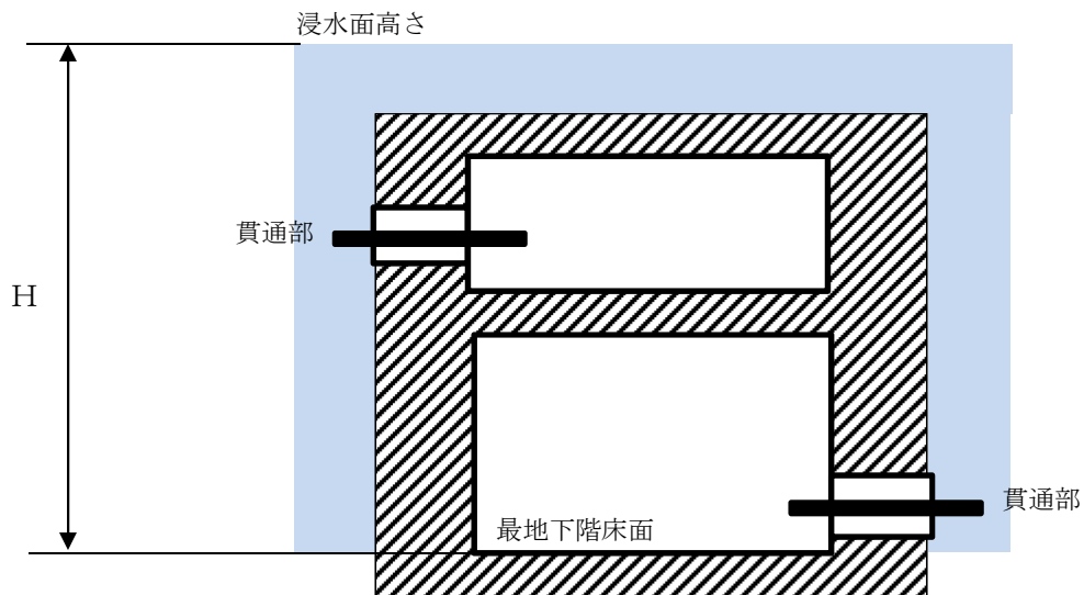
図 4-5 津波による溢水による貫通部の浸水深 h の設定
