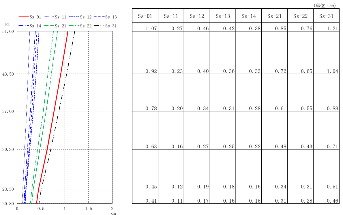
図 4-3 最大応答変位 (S s , NS 方向)
