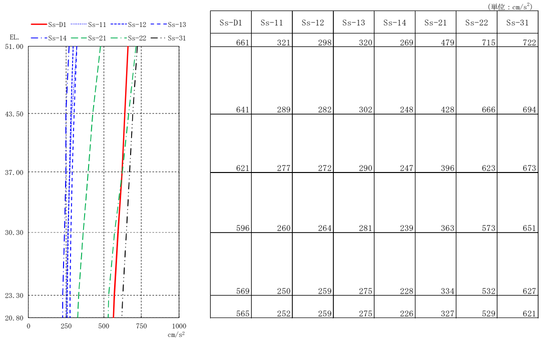
图 4-6 最大応答加速度 (S s , EW 方向)
