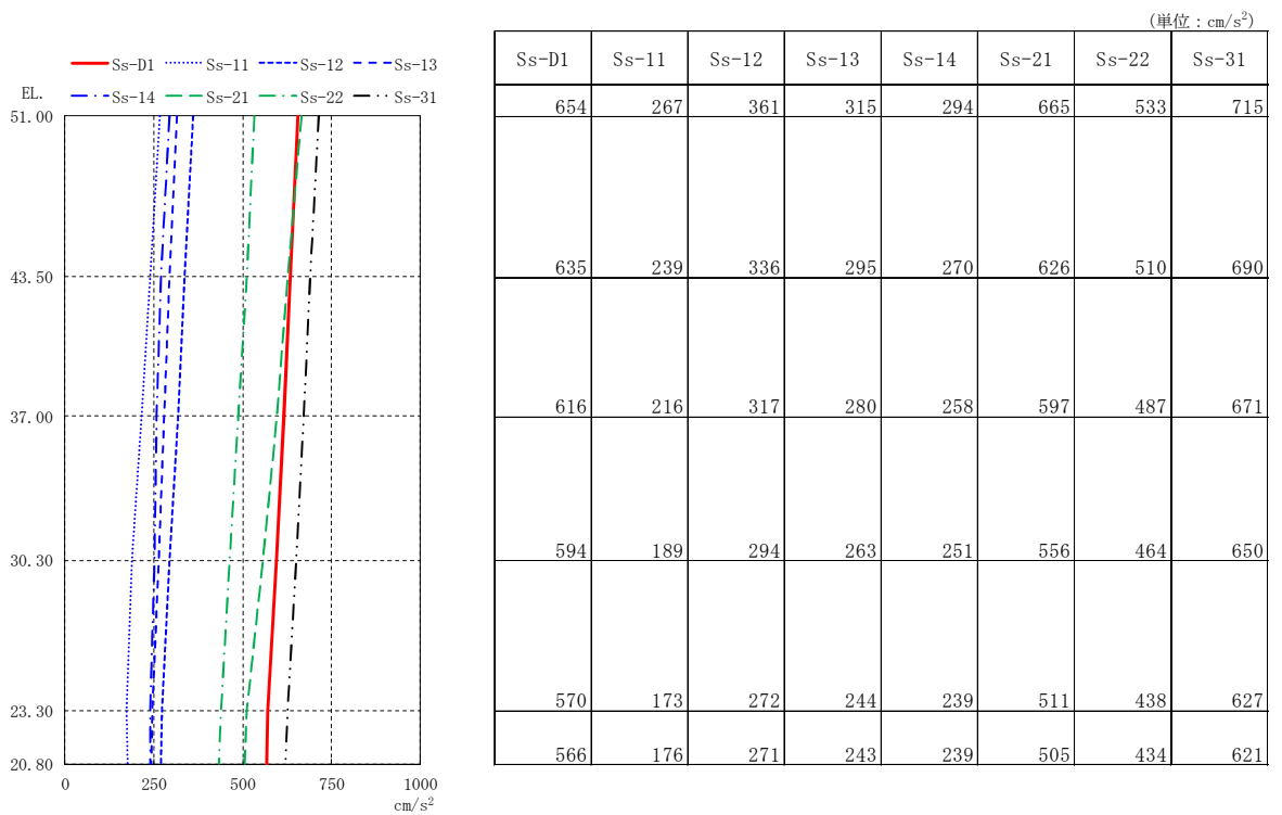
図 4-2 最大応答加速度 (S s , NS 方向)
