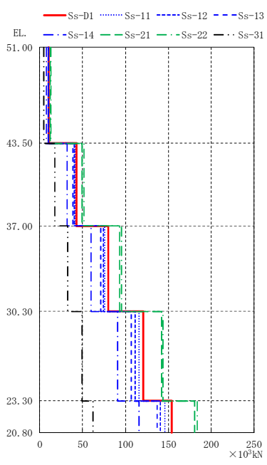
图 4-12 最大応答軸力 ( S_s , UD 方向)
