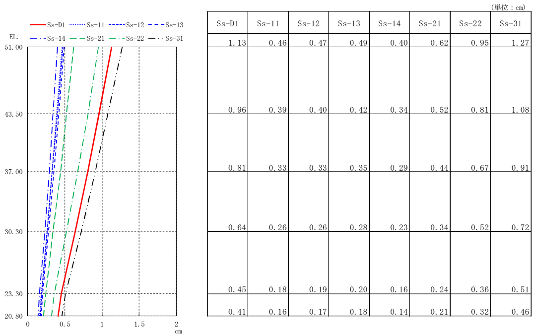
图 4-7 最大応答変位 (S s , EW 方向)
