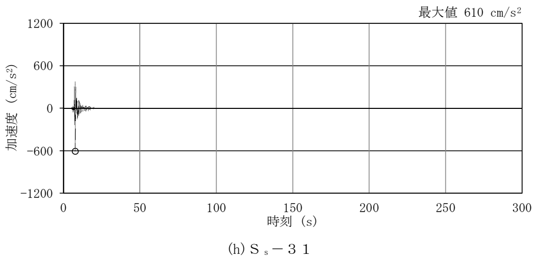
図 3-1 (3/3) 加速度時刻歴波形 ( S_s , NS 方向)
