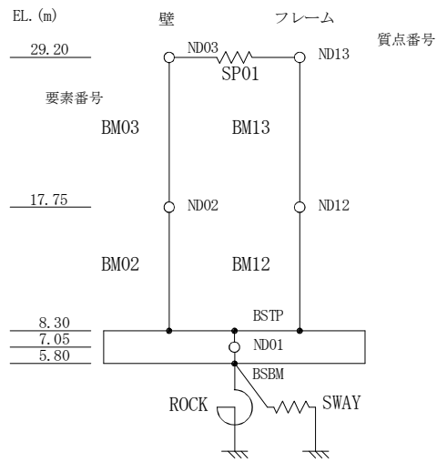
図 2-1 DC 今回工認モデル (EW 方向)
