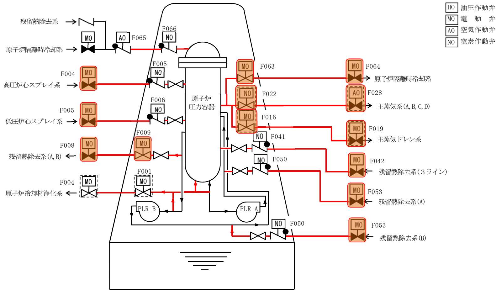
第 1 図 原子炉冷却材圧力バウンダリ
