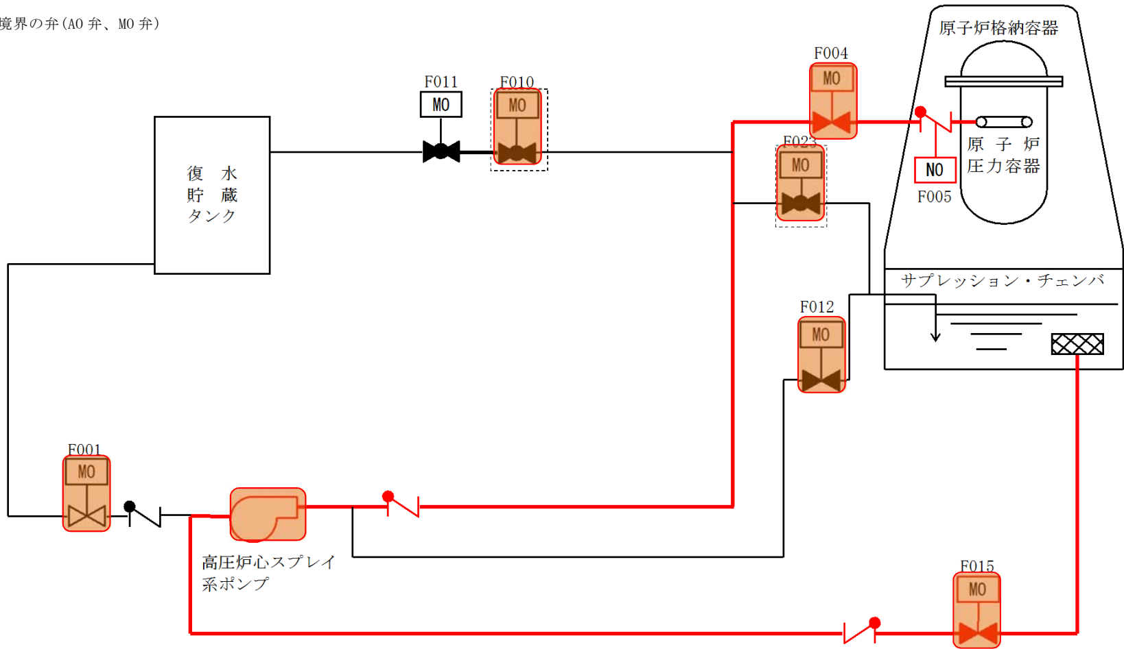
第 7 図 高圧炉心スプレイ系
