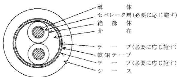
CCV-S 構造 (例)
