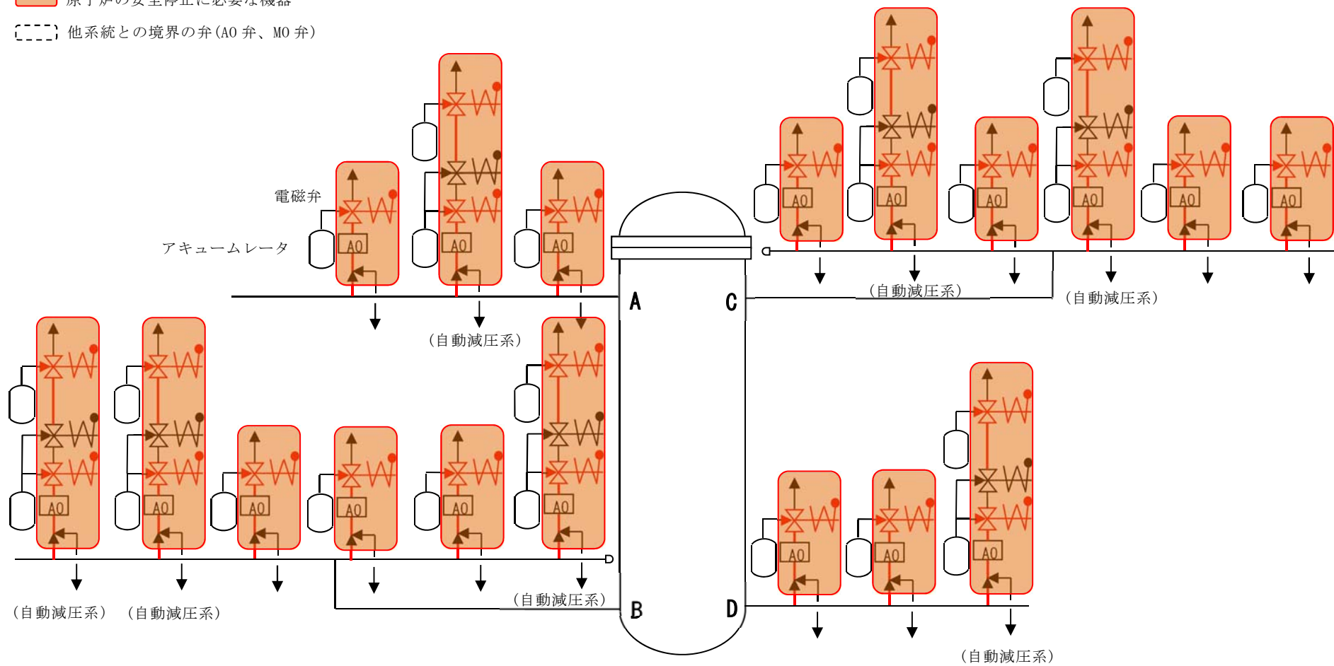
第 3 図 自動減圧系
