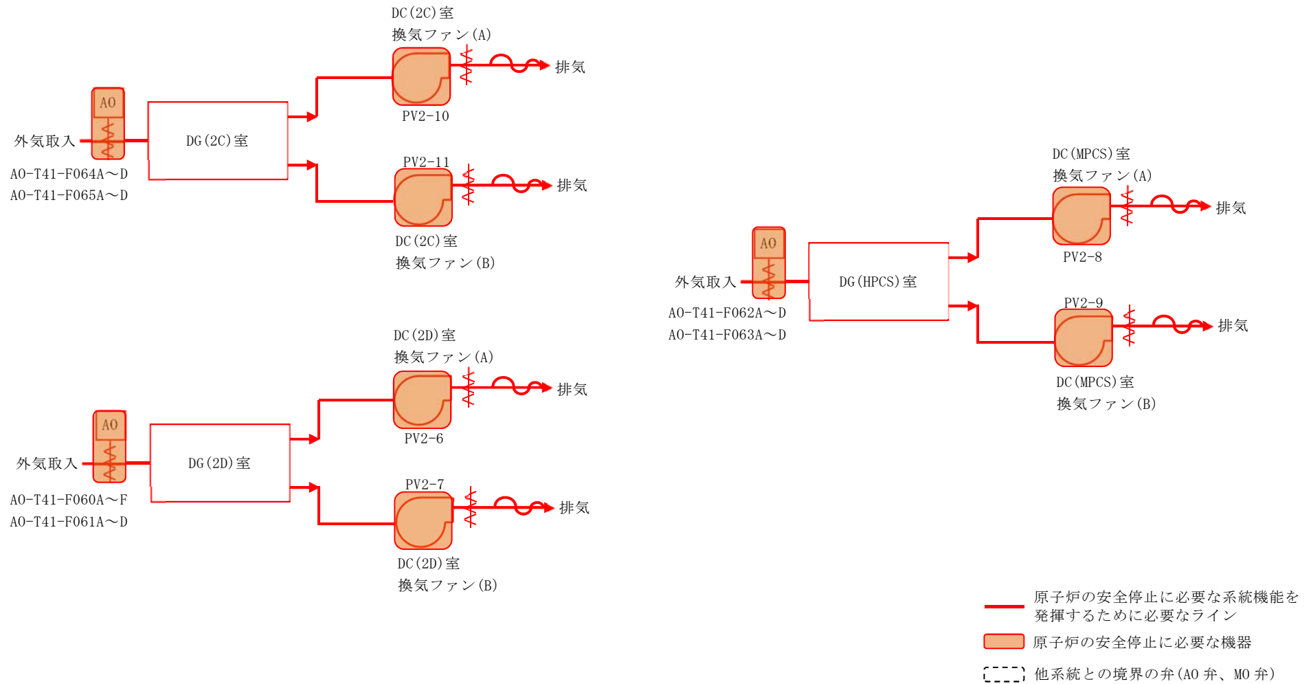
第 9 図 非常用換気空調系 (その 3)
