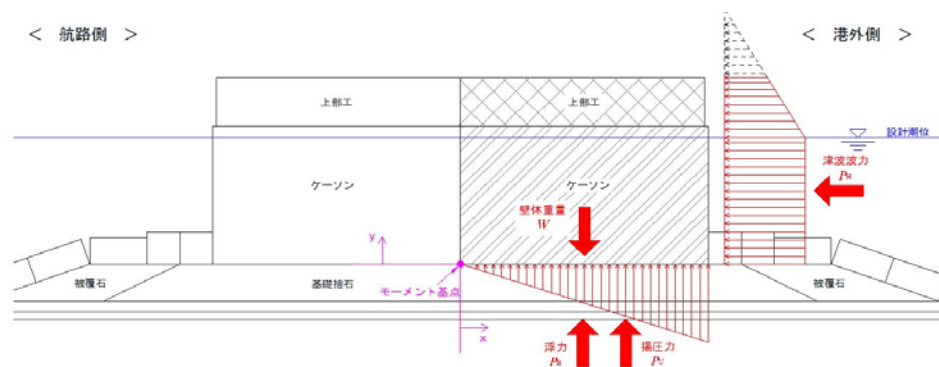
第 32 図 ケーソン堤照査図
