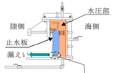
〔C-C 断面図〕
