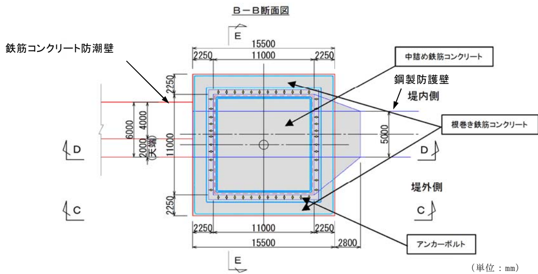
第 1-13 図 鋼製防護壁—地中連続壁基礎 結合部構造図 (B-B断面)
