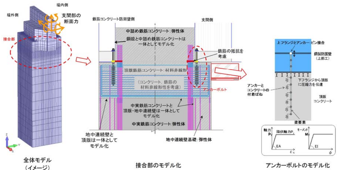
第 1-52 図(1) 接合部の三次元解析モデル化方針
