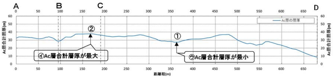
㊧ Ac層合計層厚が最大(37.8m)
