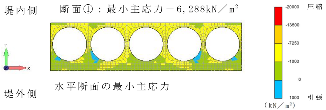
第 3-82 図 津波+余震時の解析結果
