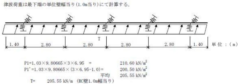
第 3-69 図 津波荷重 (水平)
