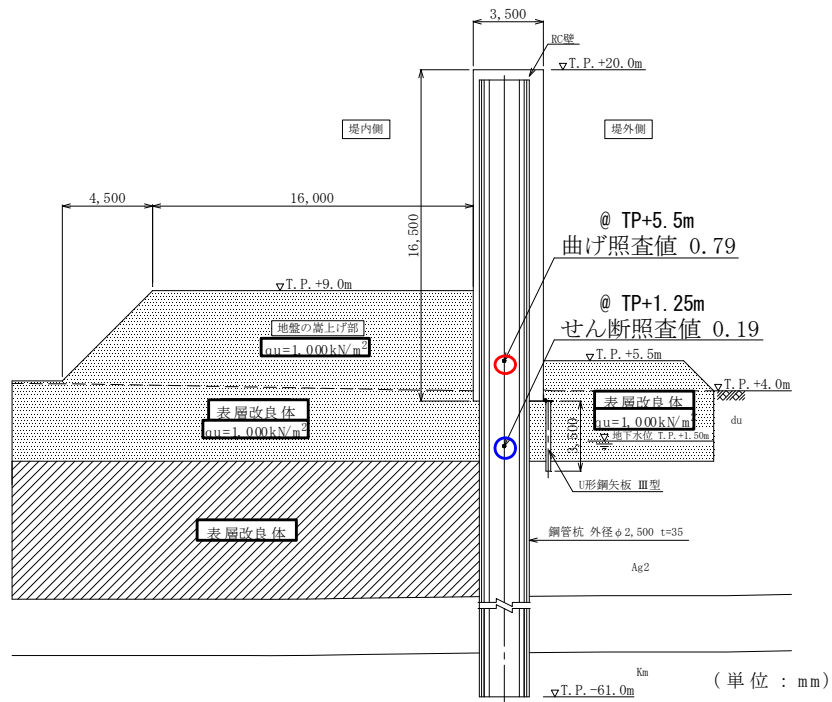
第 3-50 図 曲げ・せん断照査値
