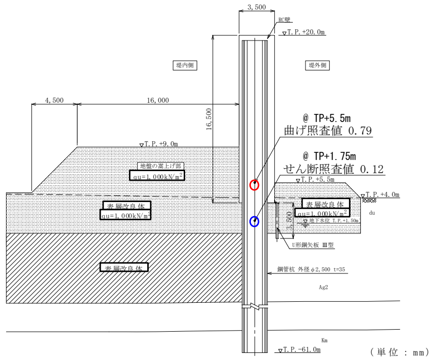
第 3-58 図 曲げ・せん断照査値 (T.P. +24m 津波 + 余震時) (その 2 のバネ)
