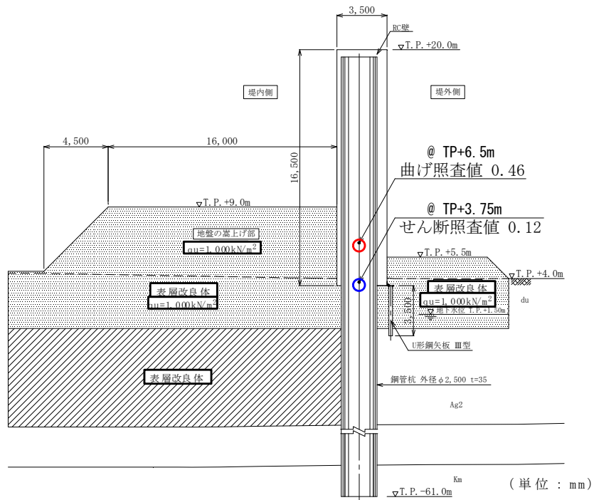
第 3-46 図 曲げ・せん断照査値
