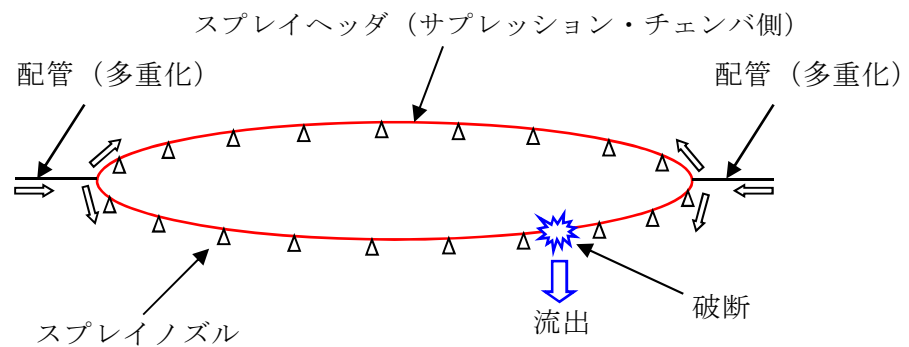
第2.1-5図 スプレイヘッダ（サプレッション・チェンバ側）
