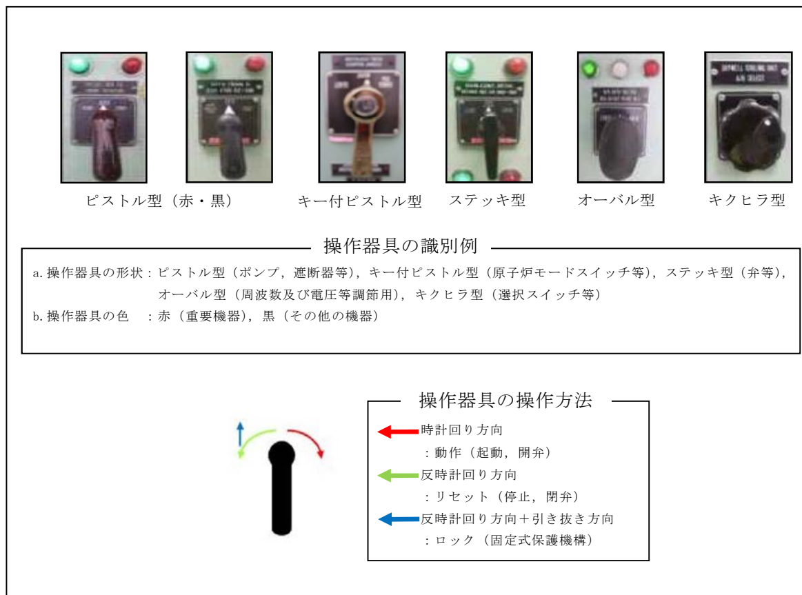
第 2. 4. 1－13 図 操作器具の識別（例）
