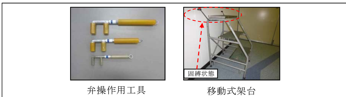
第 2. 4. 2－6 図 弁操作作用工具及び移動式架台（例）
