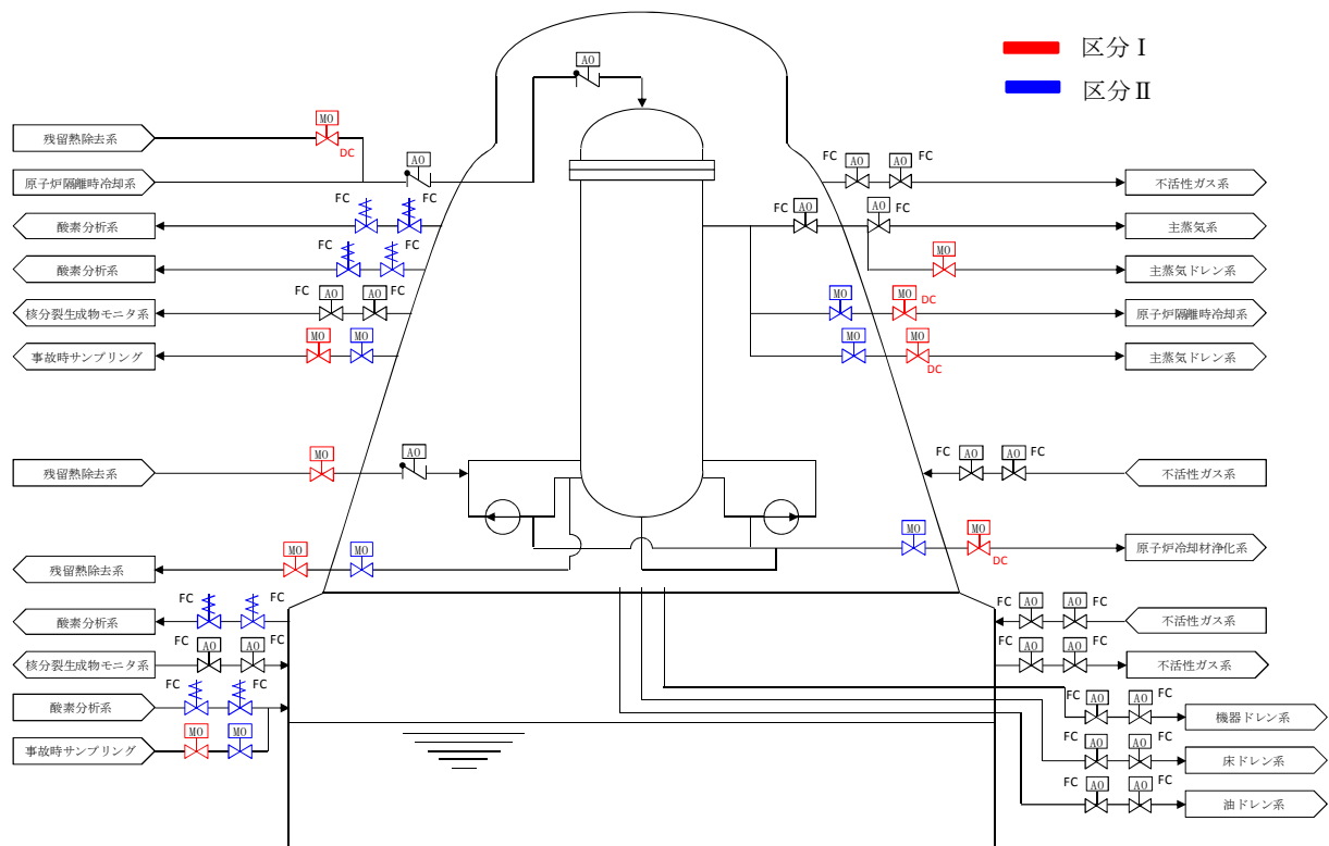
第 23-1 図 原子炉格納容器バウンダリ隔離弁 システム概略図
