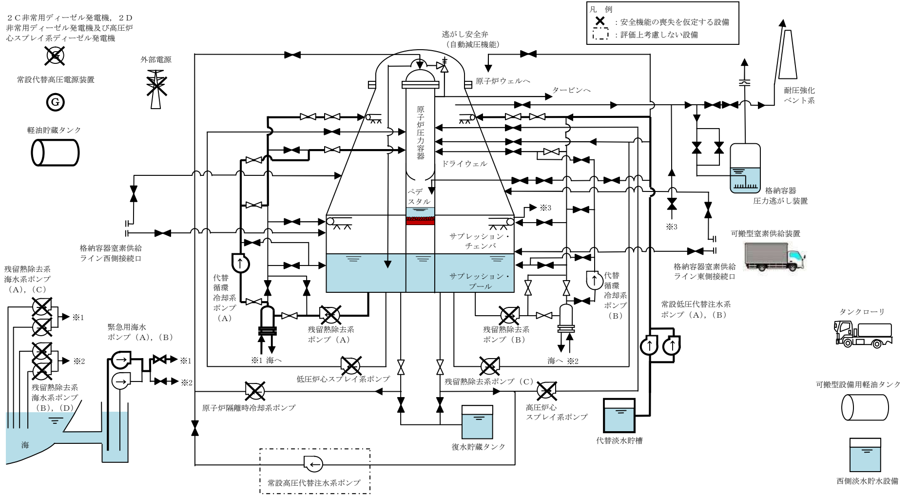
第 3.2-1 図 高圧溶融物放出／格納容器雰囲気直接加熱時の重大事故等対策の概略系統図 (4/5) (原子炉圧力容器破損後の代替循環冷却系による格納容器除熱、 代替格納容器スプレイ冷却系(常設)による格納容器冷却段階)
