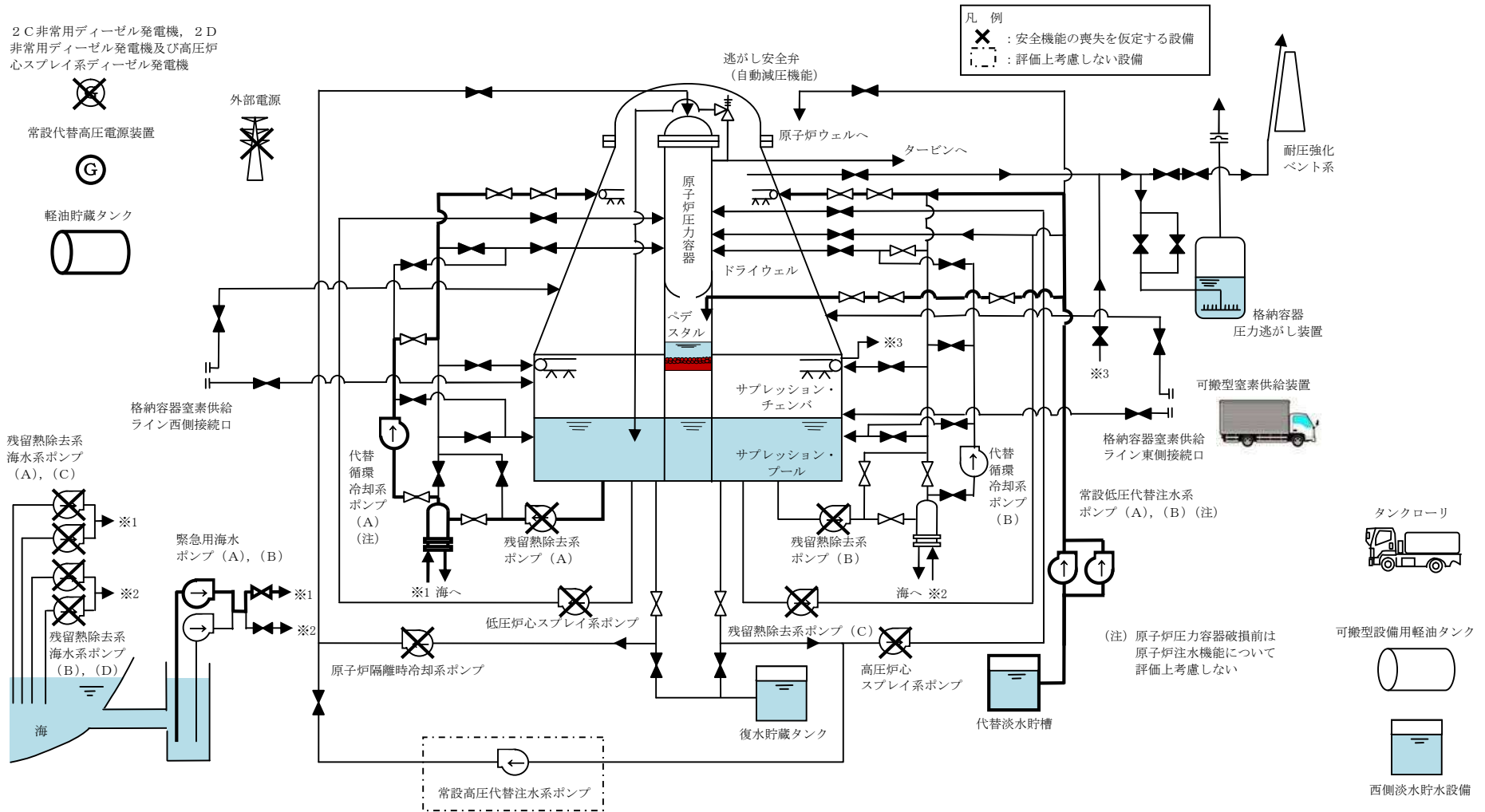
第 3.2-1 図 高压溶融物放出／格納容器雰囲気直接加熱時の重大事故等対策の概略系統図 (3/5) (原子炉压力容器破損後の代替循環冷却系による格納容器除熱，代替格納容器スプレィ冷却系 (常設) による格納容器冷却及び格納容器下部注水系 (常設) によるペDESTAL (ドライウエル部) 注水段階)
