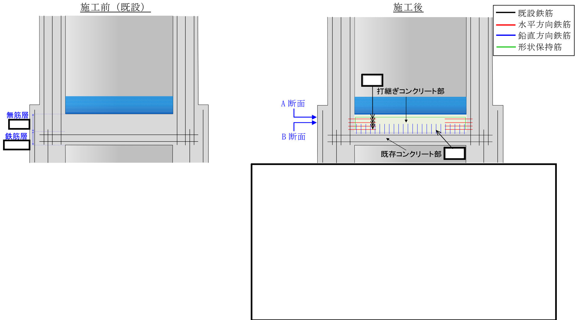
※今後の設計進捗により、詳細については安全裕度を低下させない範囲で変更となる可能性がある。 第4図 施工前後でのペDESTAL構造の比較
