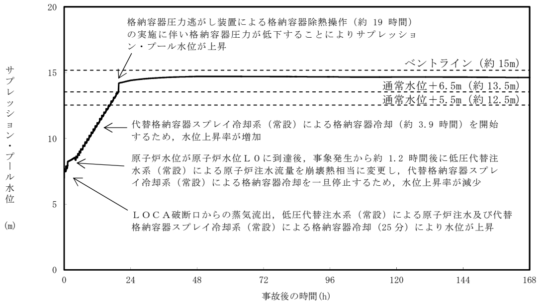
第 3.1.3-14 図 サプレッション・プール水位の推移
