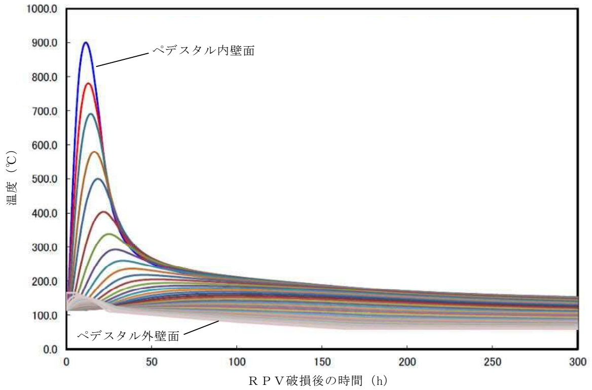
第 9 図 ペDESTAL側壁の温度変化
