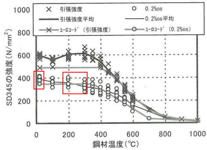
(c)SD345 の高温時強度 1), 4), 5), 9)
