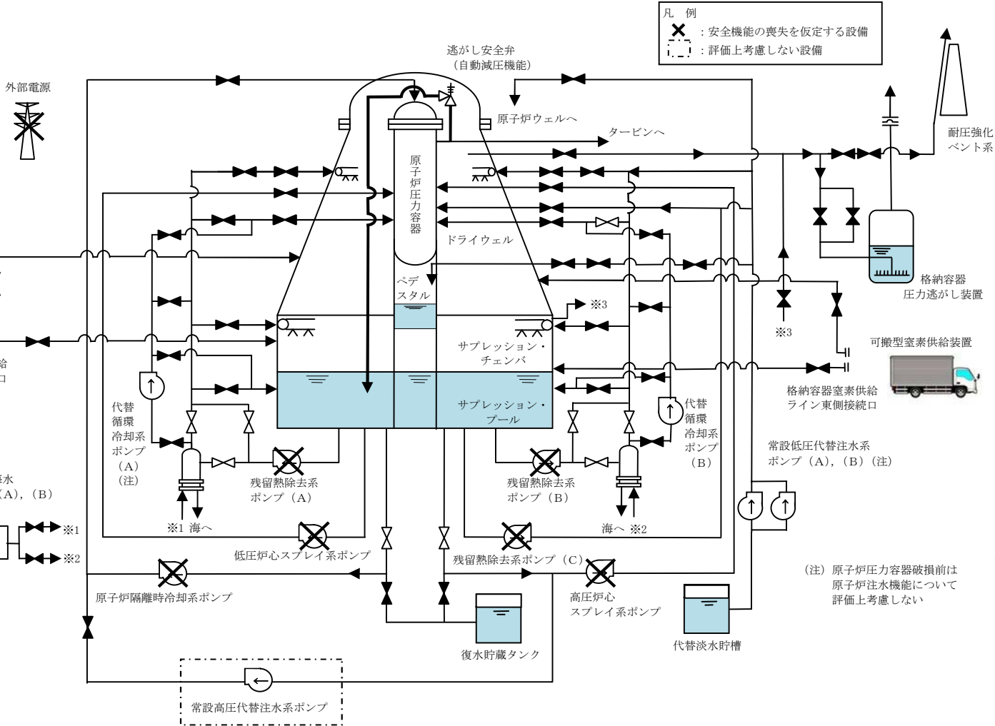
第 3.2-1 図 高圧溶融物放出／格納容器雰囲気直接加熱時の重大事故等対策の概略系統図 (1/5) (原子炉压力容器破損前の逃がし安全弁 (自動減圧機能) による原子炉減圧段階)
