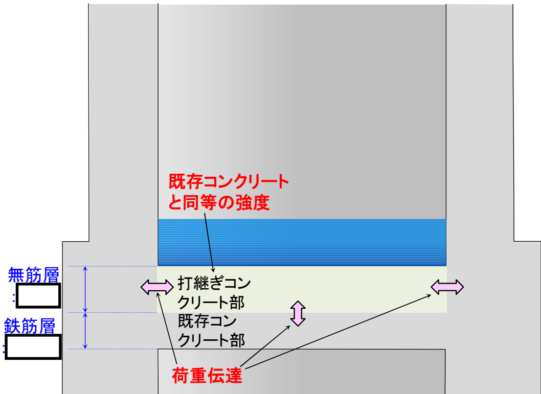
第2図 ペDESTALでの荷重伝達
