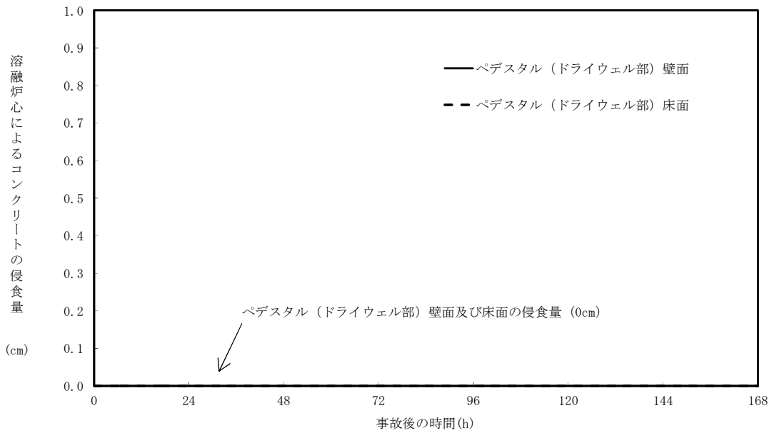
第 3.5-2 図 ペDESTAL (ドライウエル部) の壁面及び床面のコンクリート侵食量の推移
