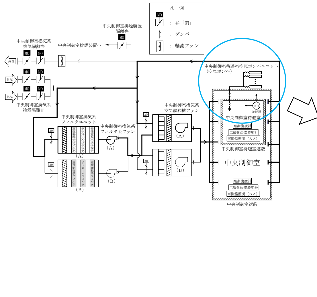
第59-4-2図 中央制御室待避室空気ポンプユニット 系統概要図
