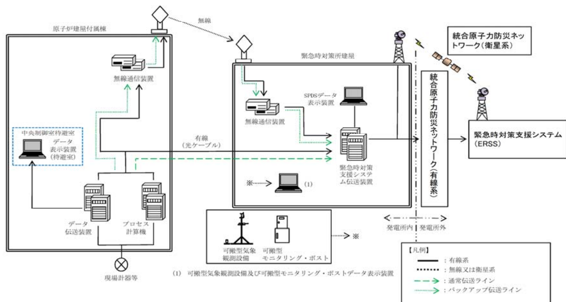
第 62-6-6 図 過去のプラントパラメータ閲覧の概要
