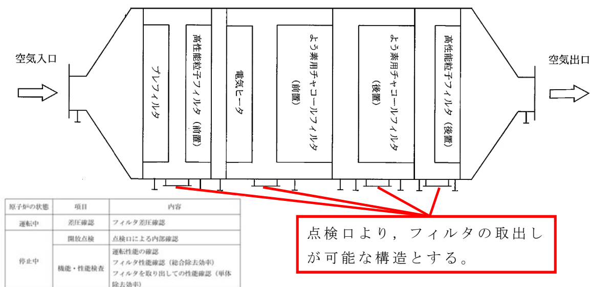
第 61-5-9 図 緊急時対策所非常用フィルタ装置
