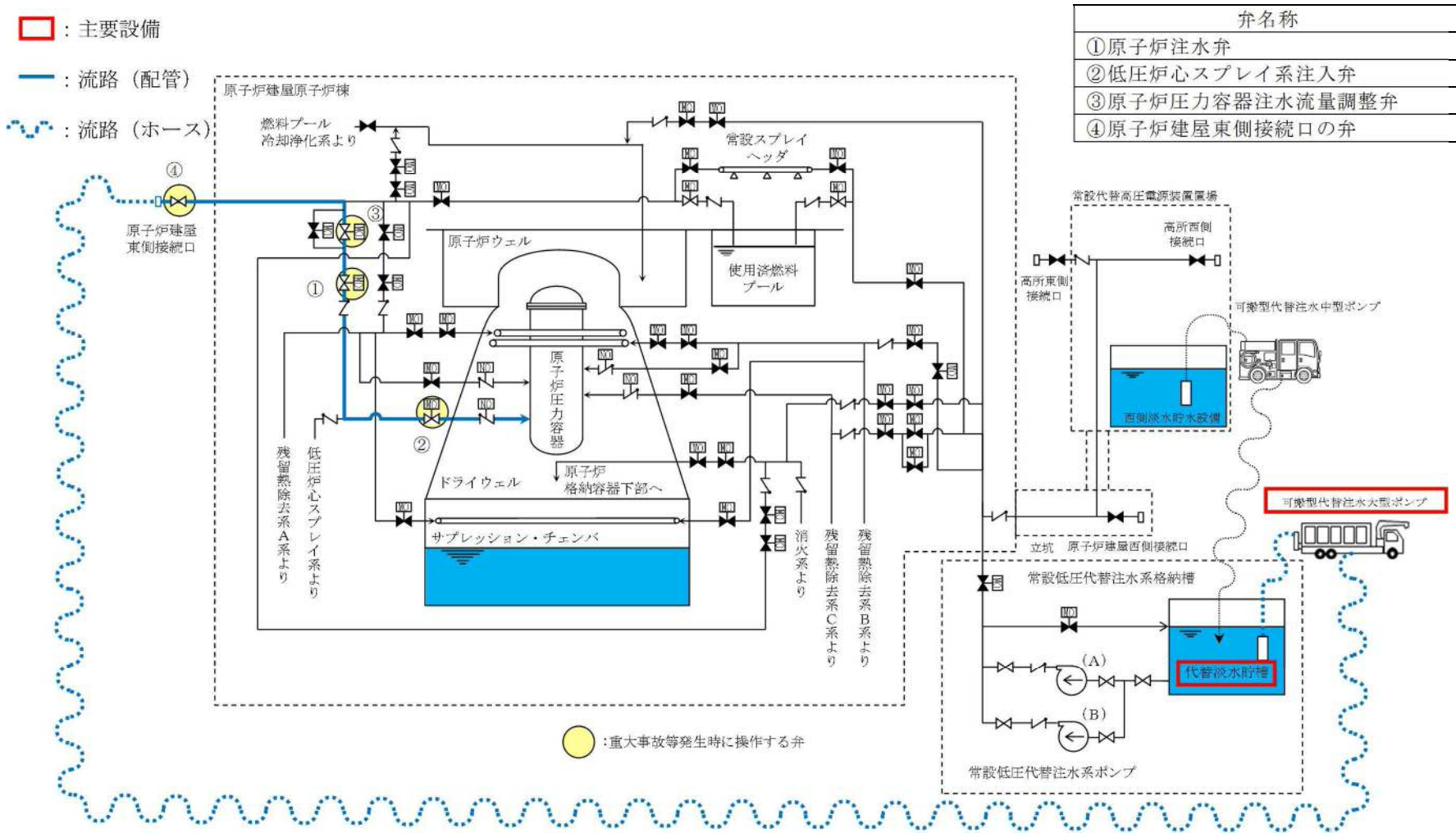
第 3.4-3 図 低压代替注水系（可搬型）系統概要図（代替淡水貯槽～原子炉建屋東側接続口）
