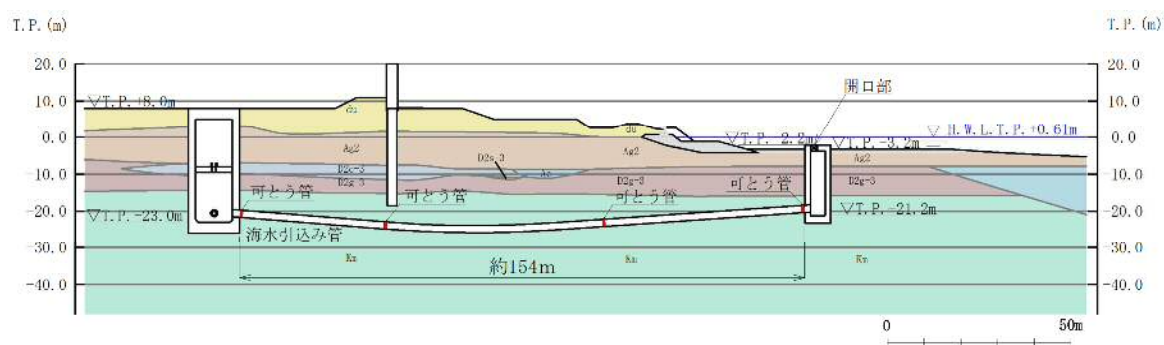
第 3.9-2 図 海水引込み管 縦断面図
