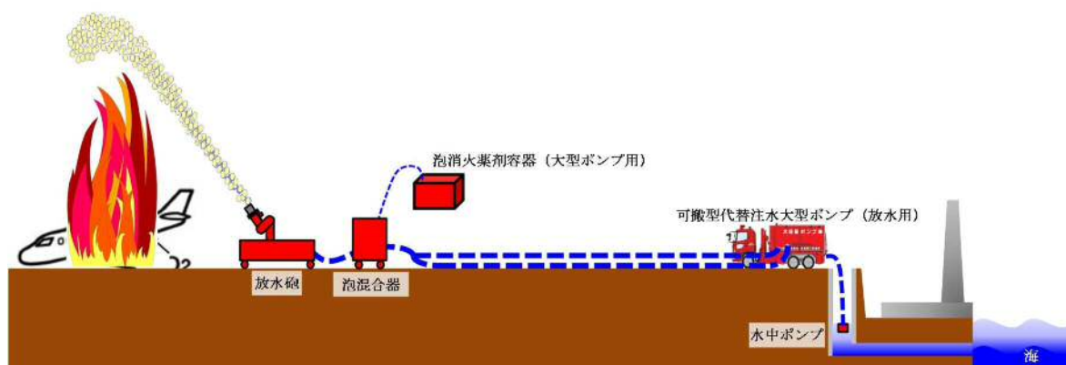
第3. 13－17図 系統概要図（海水を水源とした航空機燃料火災への泡消火）
