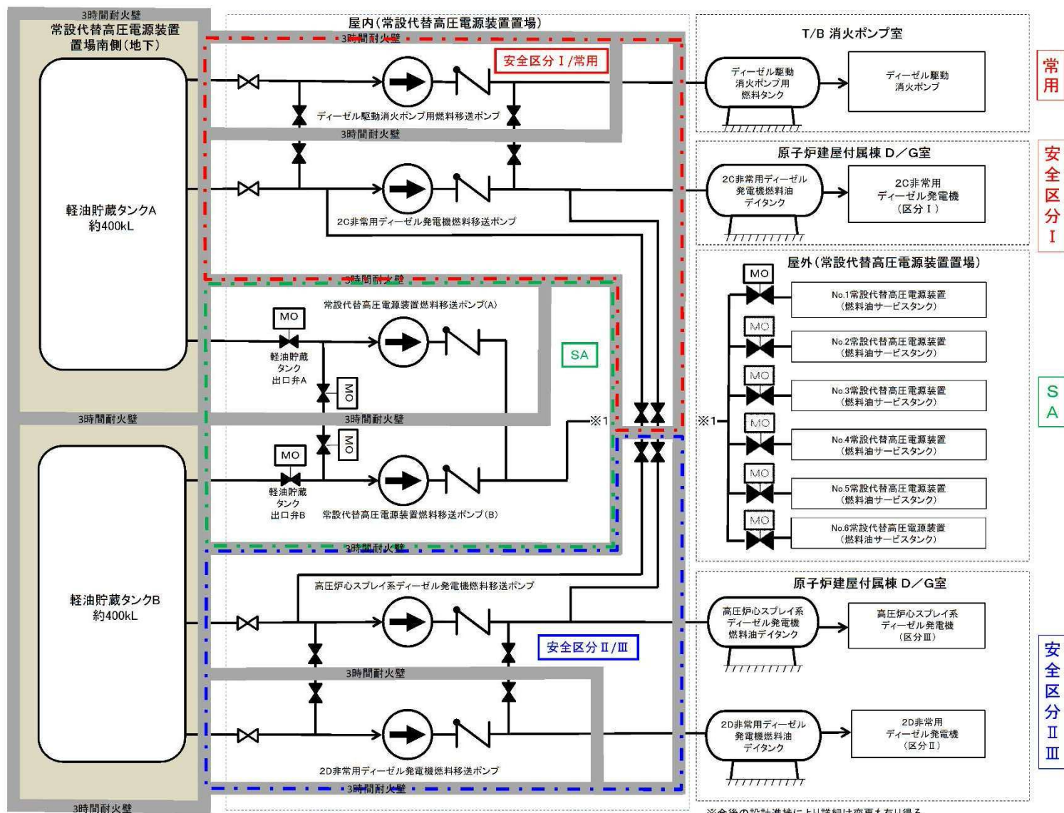
第 10.2-10 図 代替電源設備 系統図 (軽油貯蔵タンクから常設代替高圧電源装置への給油)
