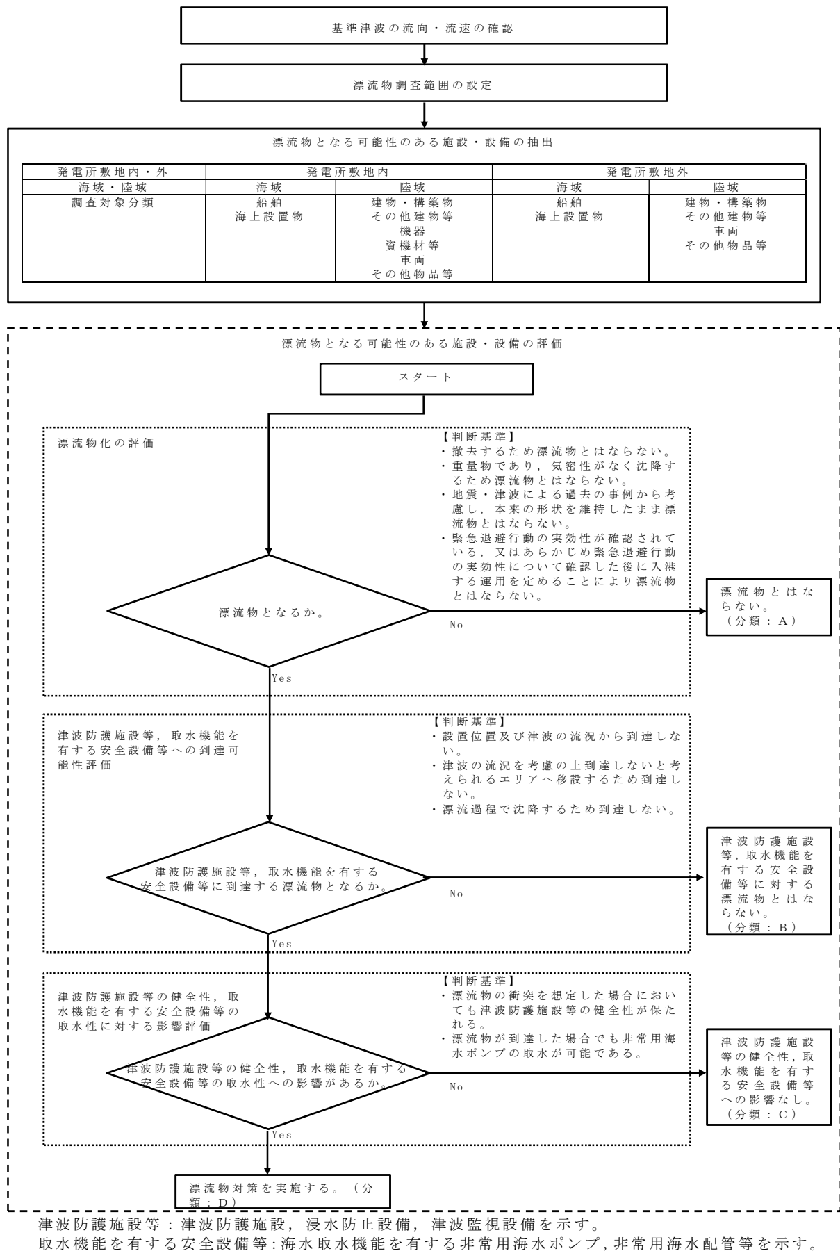
第 2.1.3-12 図 漂流物影響評価フロー
