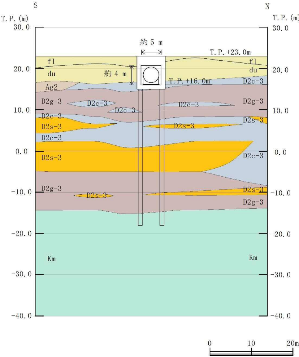
第 3.11-2 図 緊急時対策所用発電機燃料油貯蔵タンク基礎 断面図
