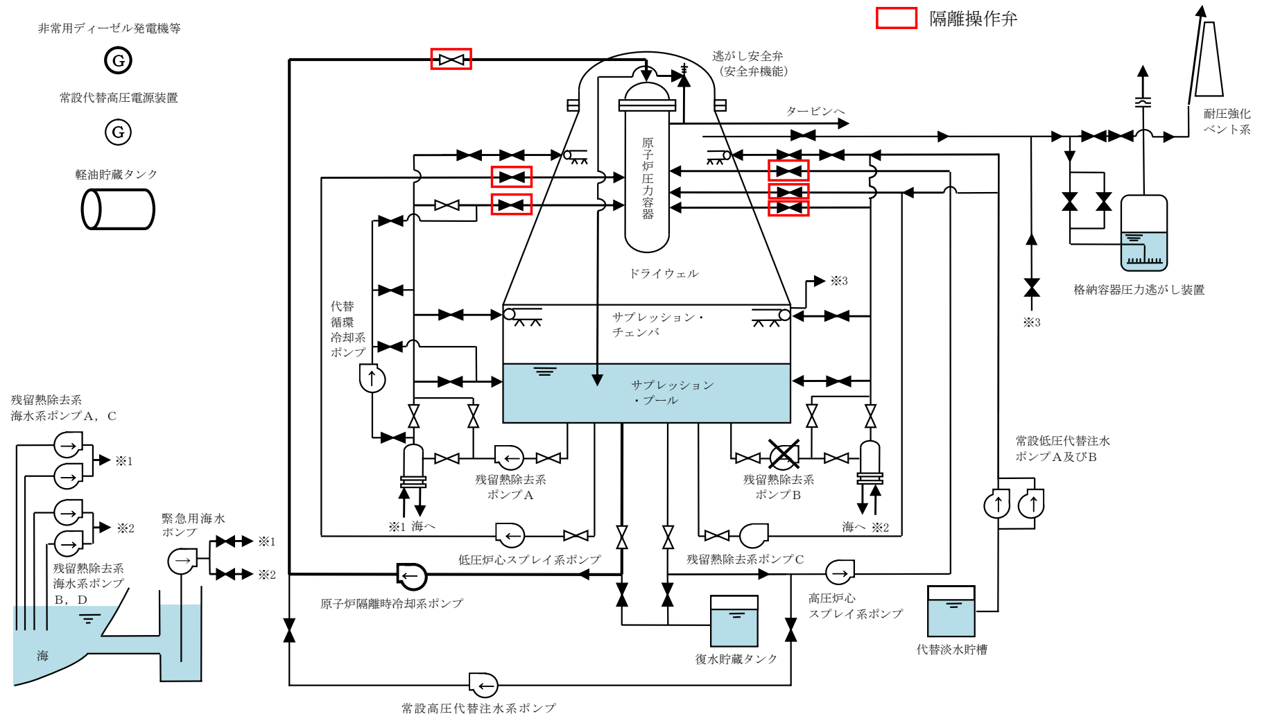
第 3.3-3-6 図 インターフェイスシステム LOCA 隔離弁 系統概要図
