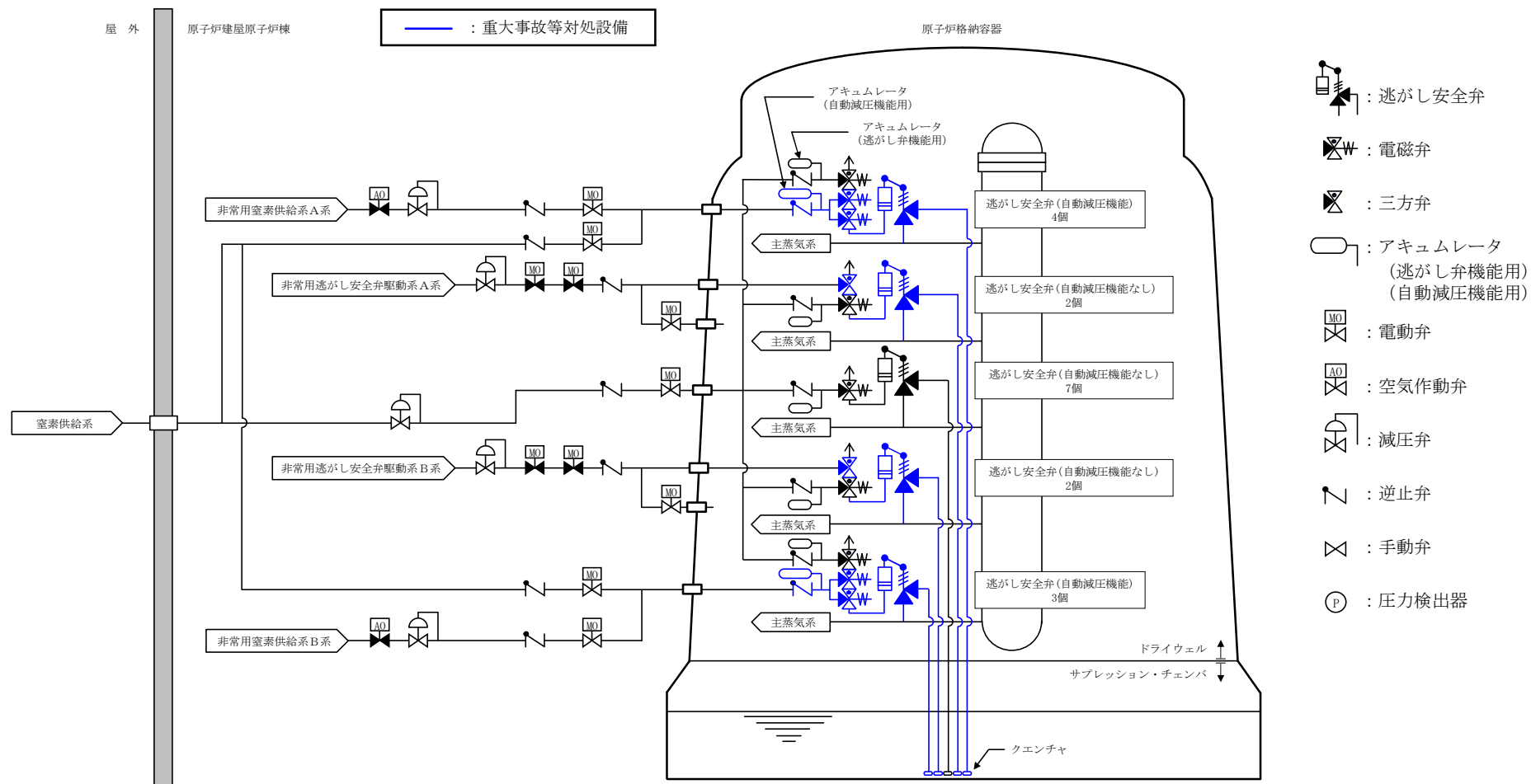
第 3.3-1 図 逃がし安全弁及びアキュムレータに関する系統概要図
