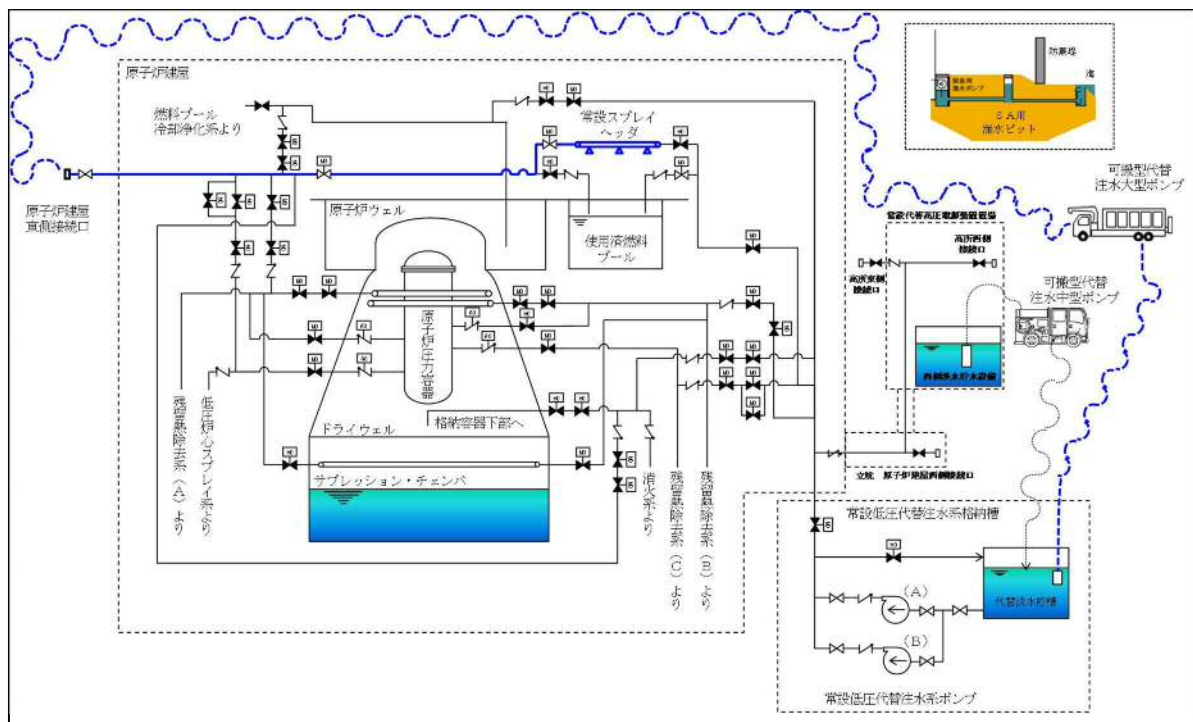
第 3.13-10 図 系統概要図 (代替淡水貯槽を水源とした代替燃料プール注水系(常設スプレイヘッド)(可搬型)) 原子炉建屋東側接続口使用時
