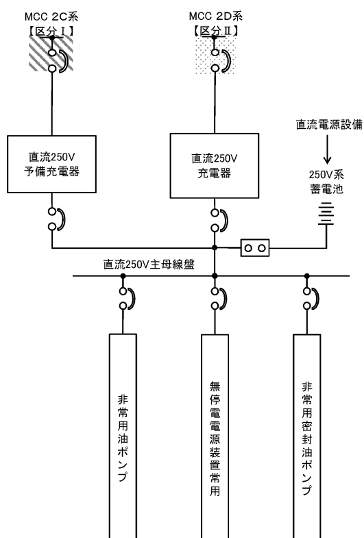
第 10.1-3 図 直流電源単線結線図 (3/3)
