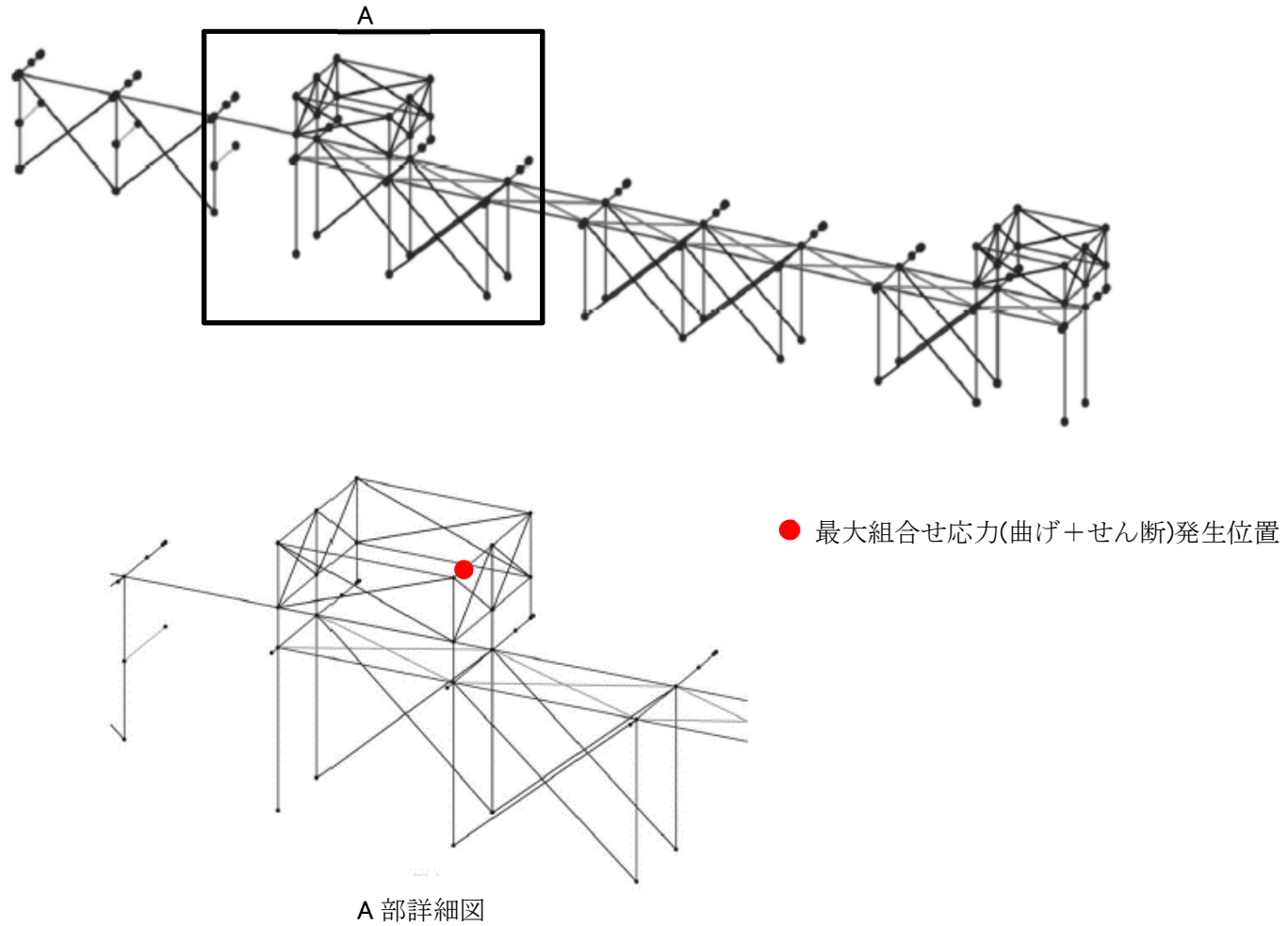
(b) 鉄骨架構における最大応力発生位置(エリア⑧)
