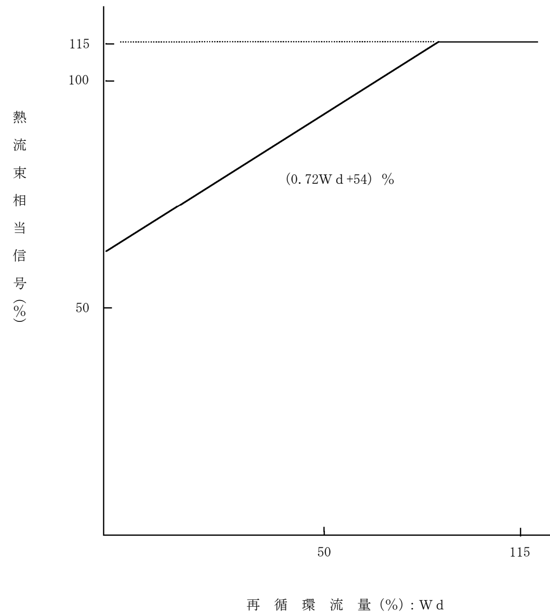
図 6-1 中性子束高—自動可変設定（熱流束相当）の原子炉非常停止信号の設定値
