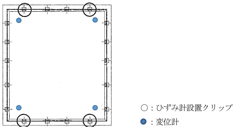
第11図 計測器取付位置図
