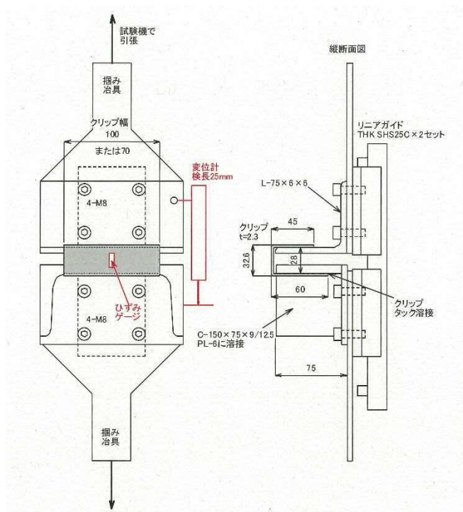
第 2-15 図 クリップの引張試験概要図
