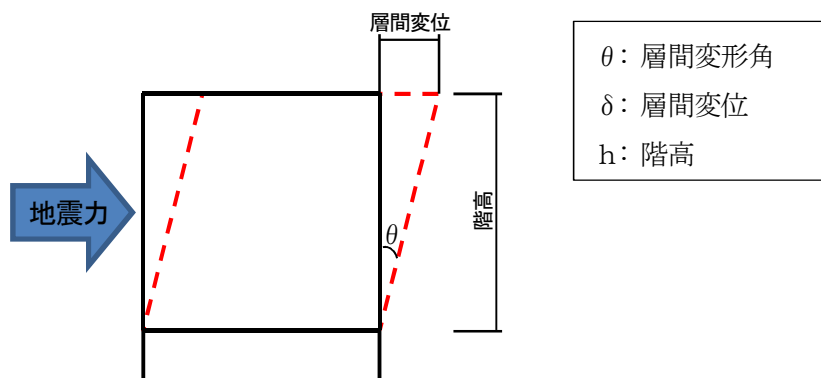
第4図 層間変形角
