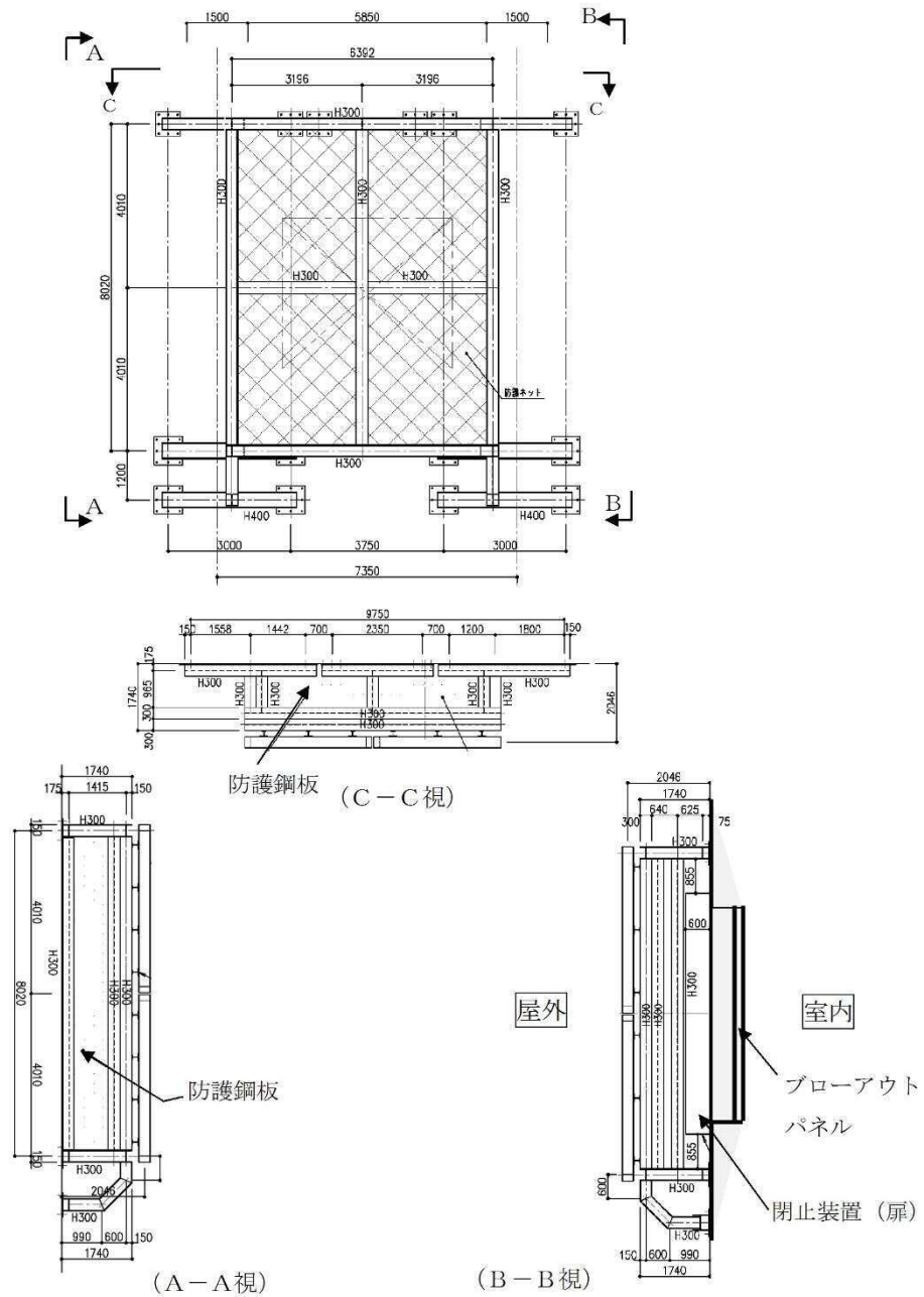
第5-1図 竜巻防護ネットの構造図
