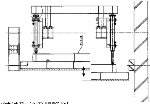
第2図 ブローアウトパネル及び取付け架台の概略図
