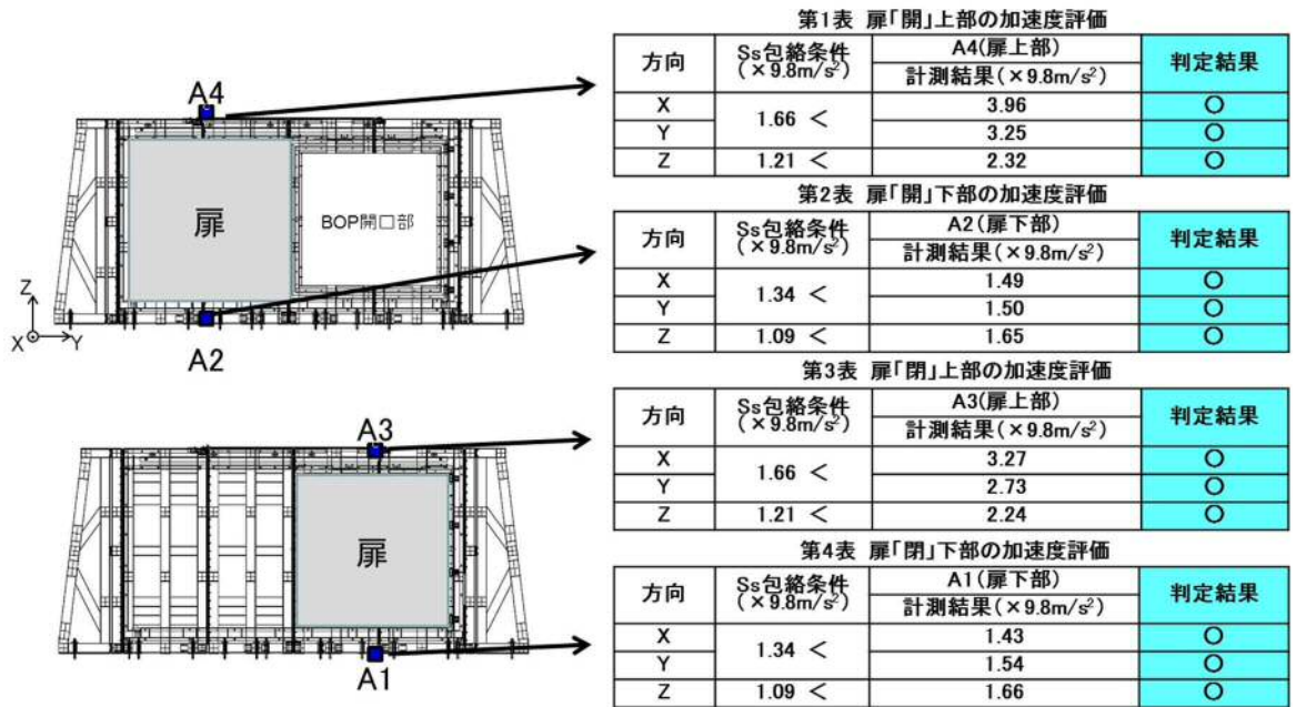
第8-1図 加振試験時の加速度評価 (本試験時)
