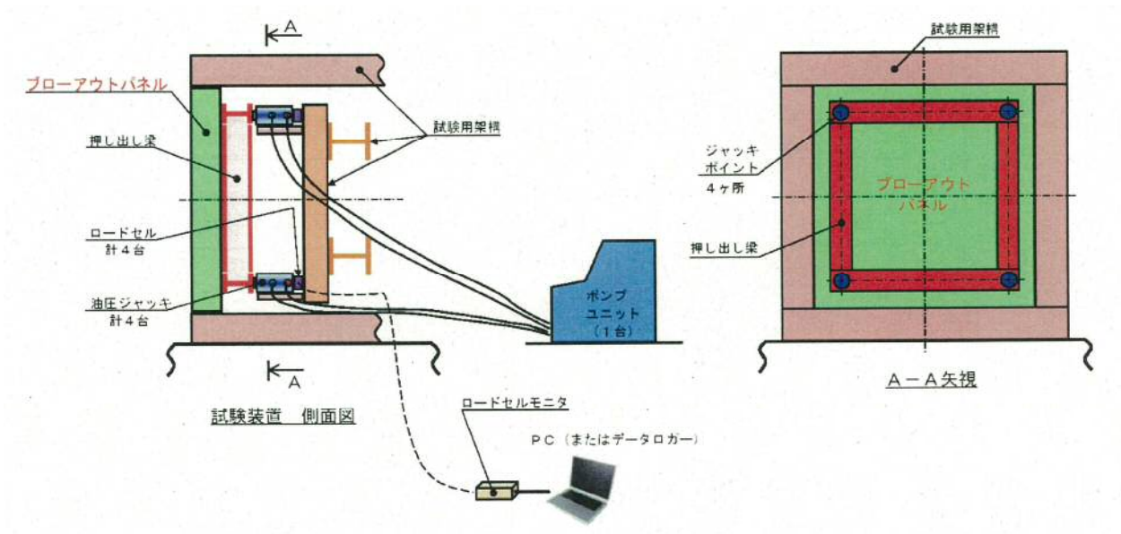
第6図 試験機器配置及び構成概念図
