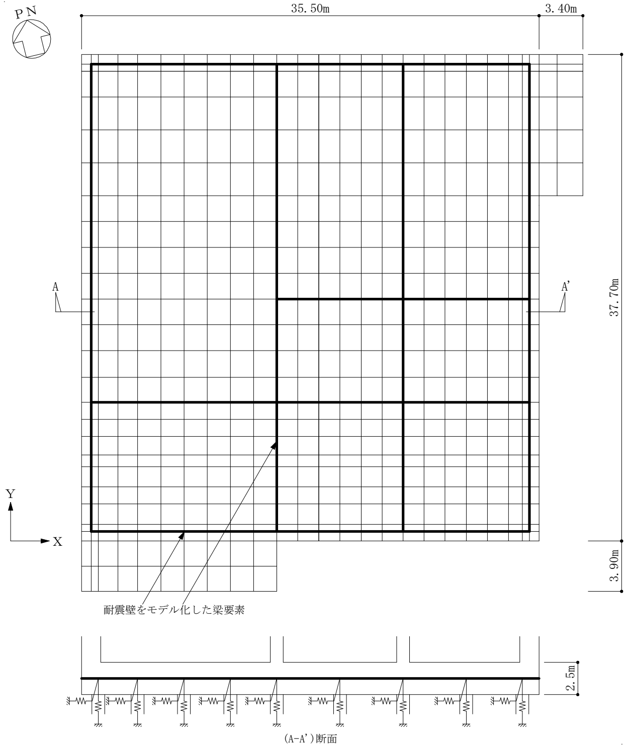
図 4-3 解析モデル
