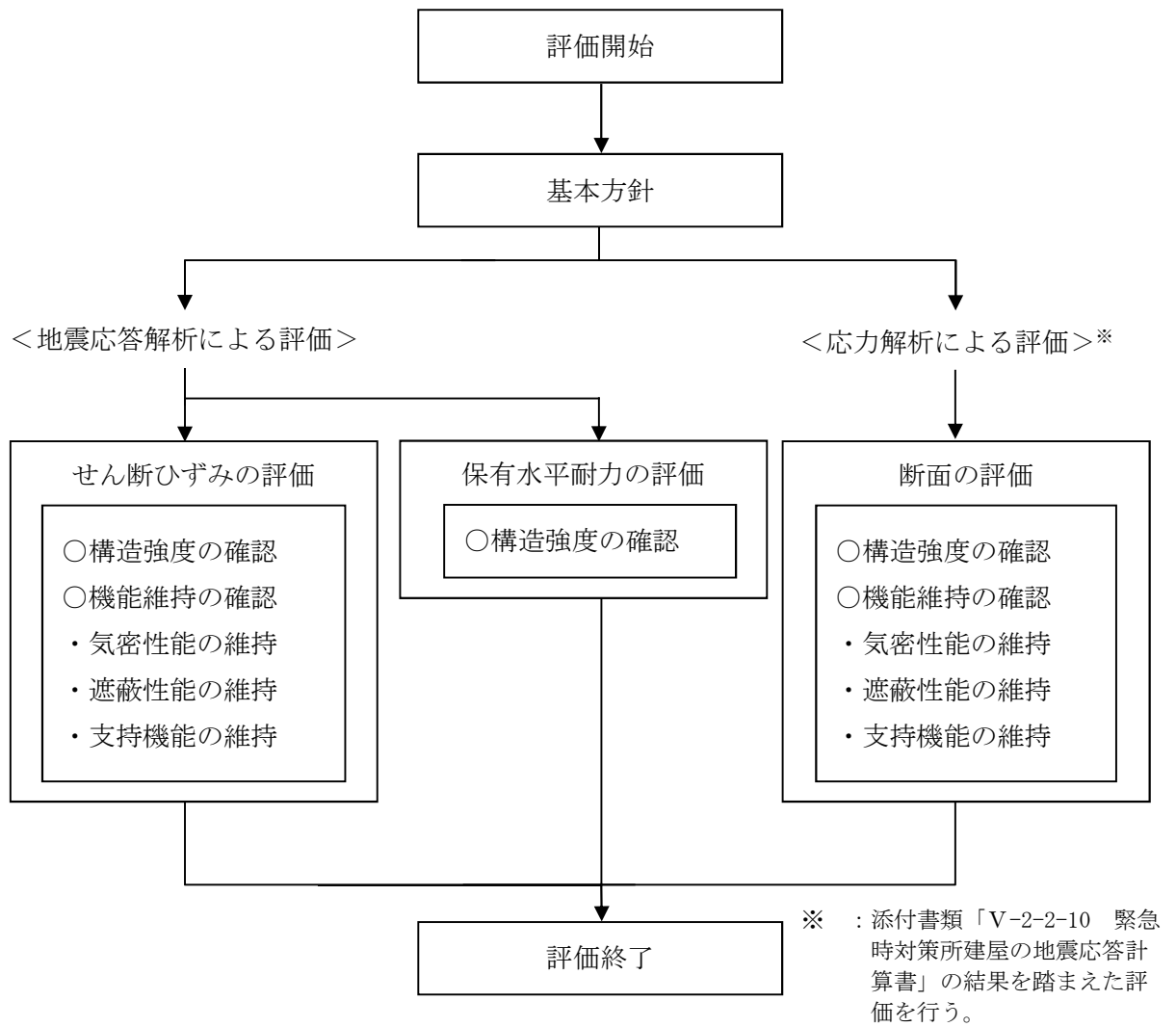
図 2-7 緊急時対策所建屋の評価フロー
