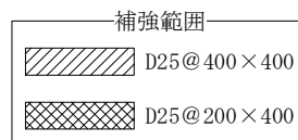
図 5-3 セン断補強筋の設定範囲
