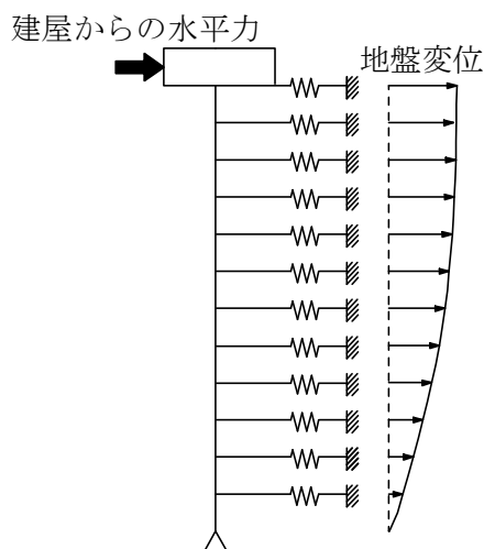
図4-4 解析モデル
